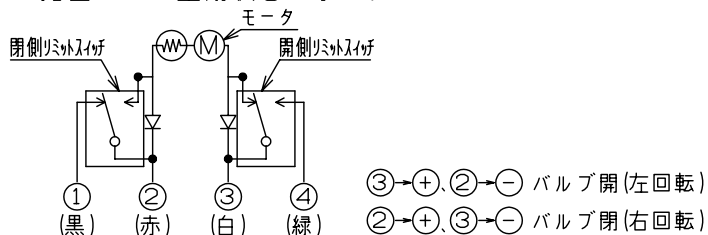
回路図 ※全閉状態を示す。
