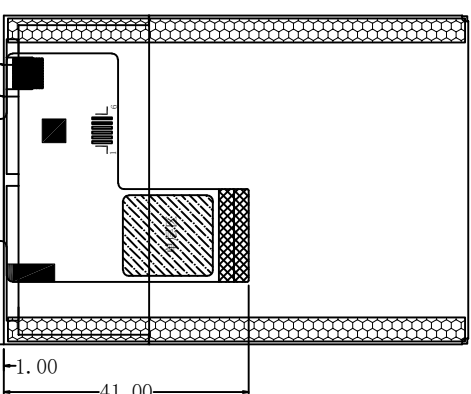
FPC弯折示意图 FPC展开出货
