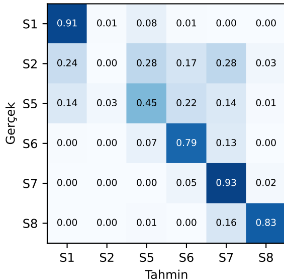
YOLO26n-cls füzyon
