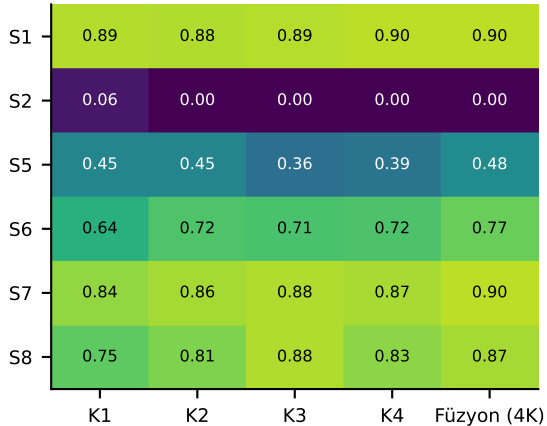
yolo26n-cls
