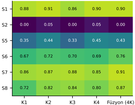
yolo11n-cls
