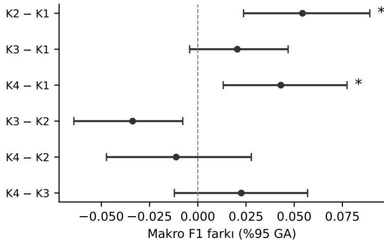
yolo11n-cls
