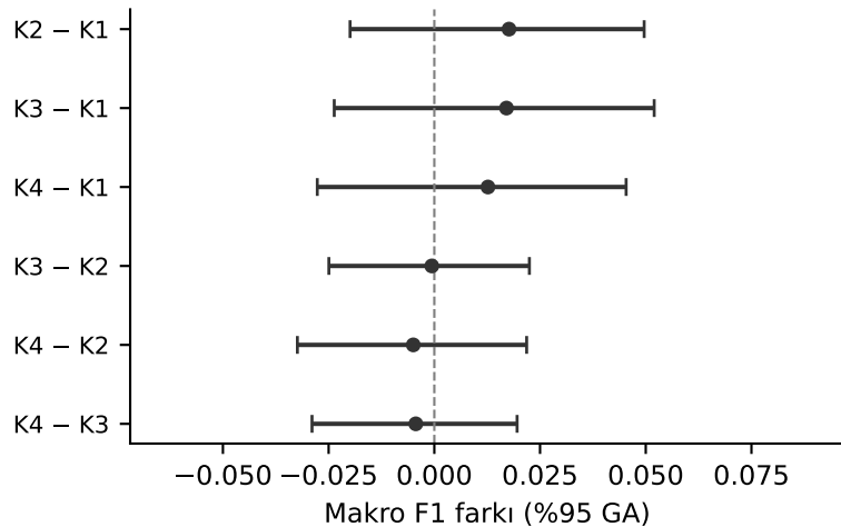
yolo26n-cls
