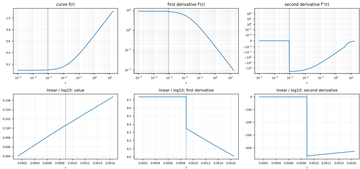
FUJIFILM F-Log
