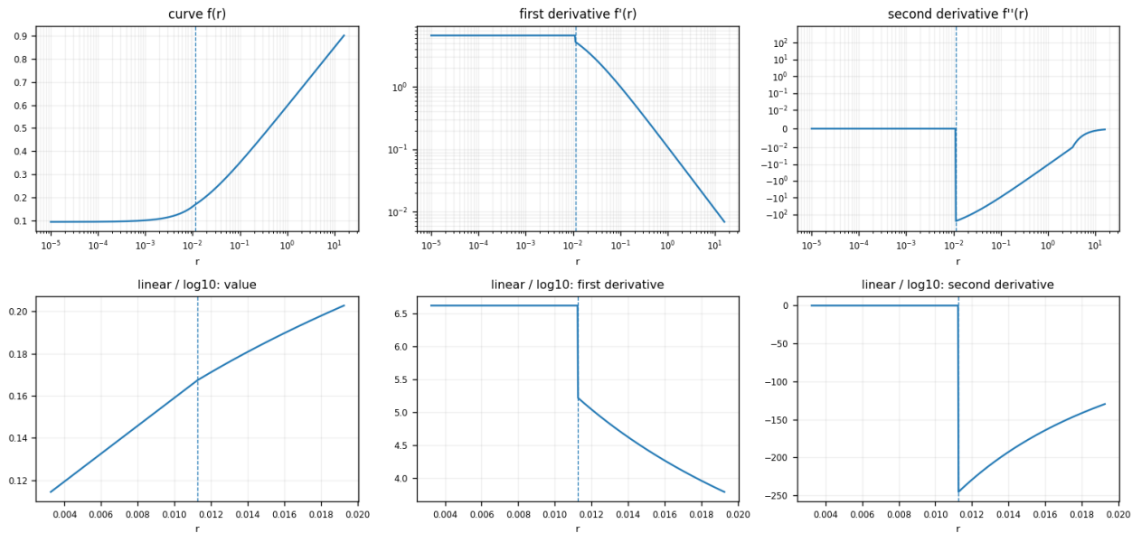
Sony S-Log3
