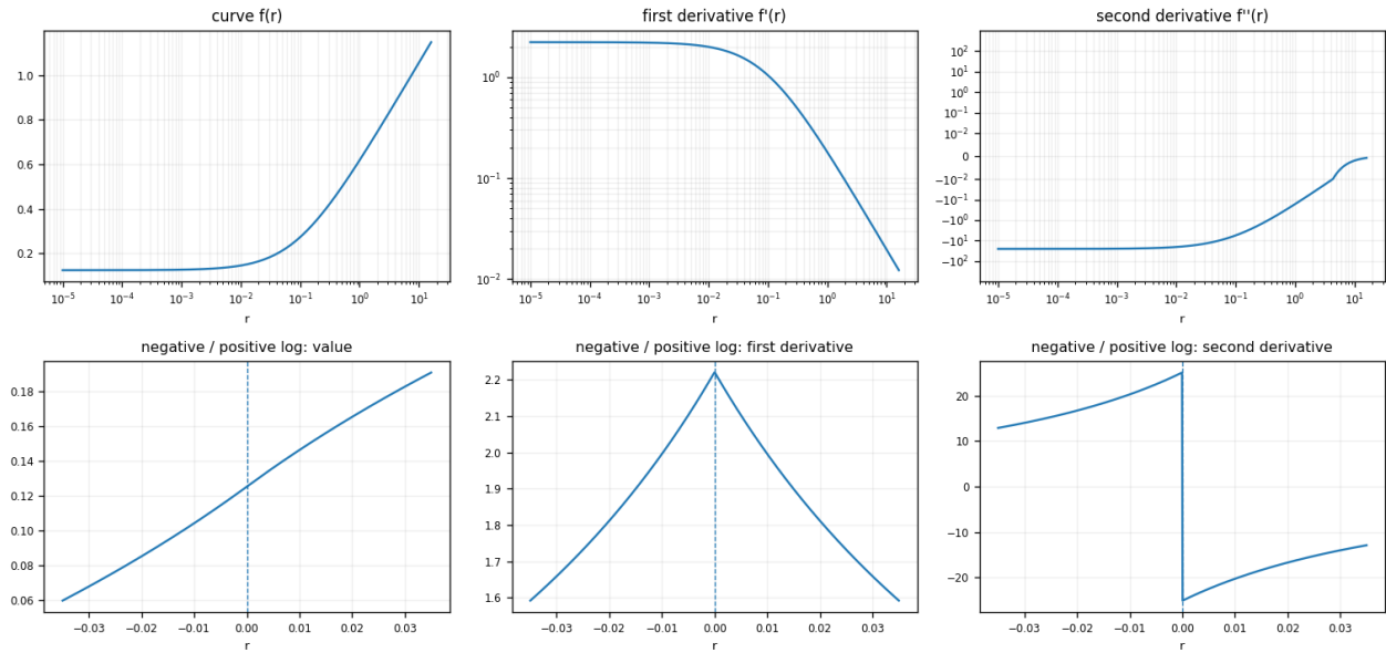
Canon Log
