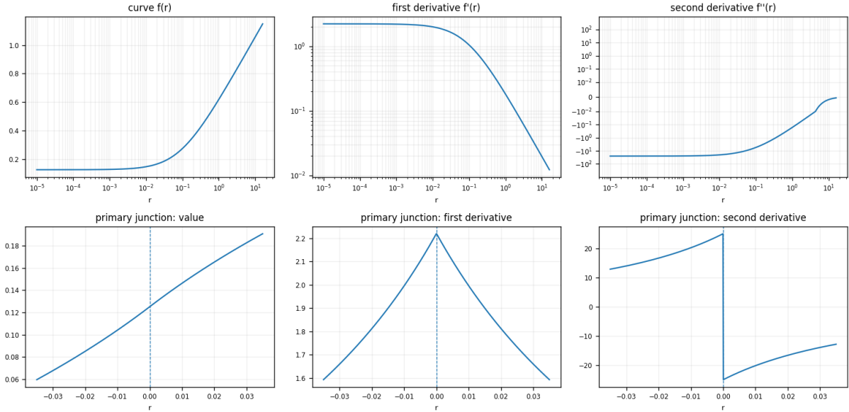
Canon Log
