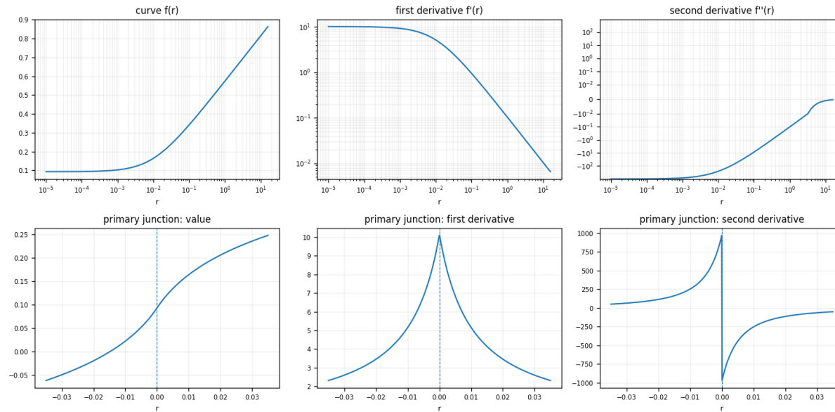
Canon Log 2
