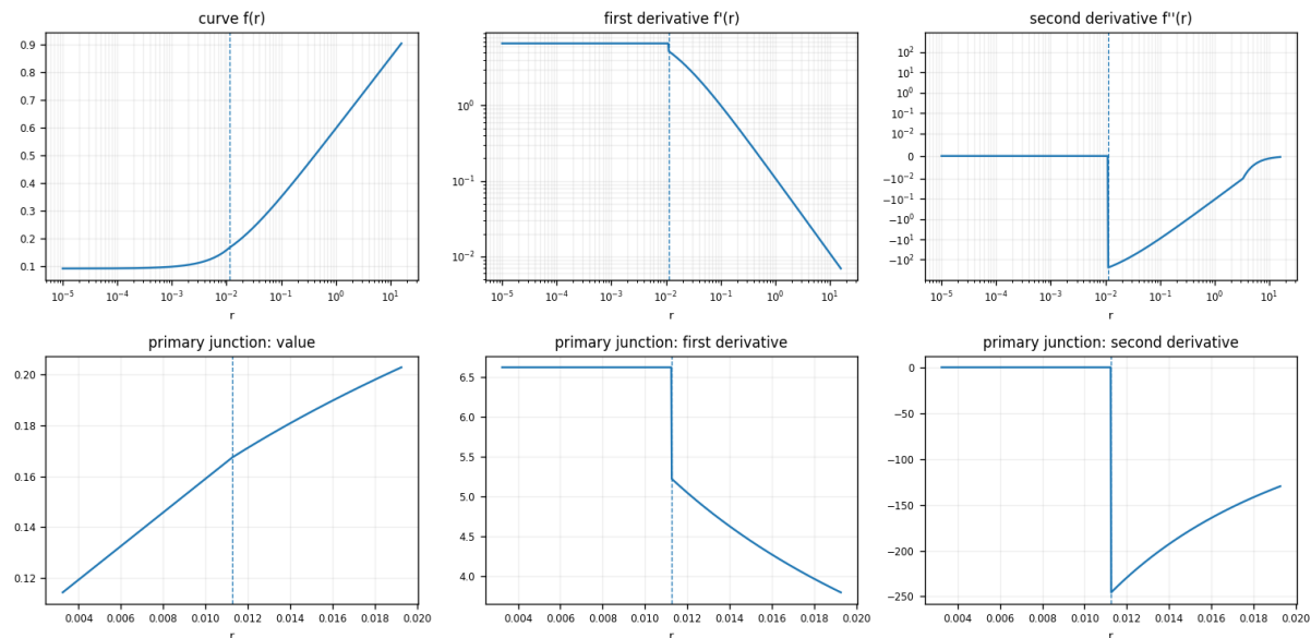
Sony S-Log3
