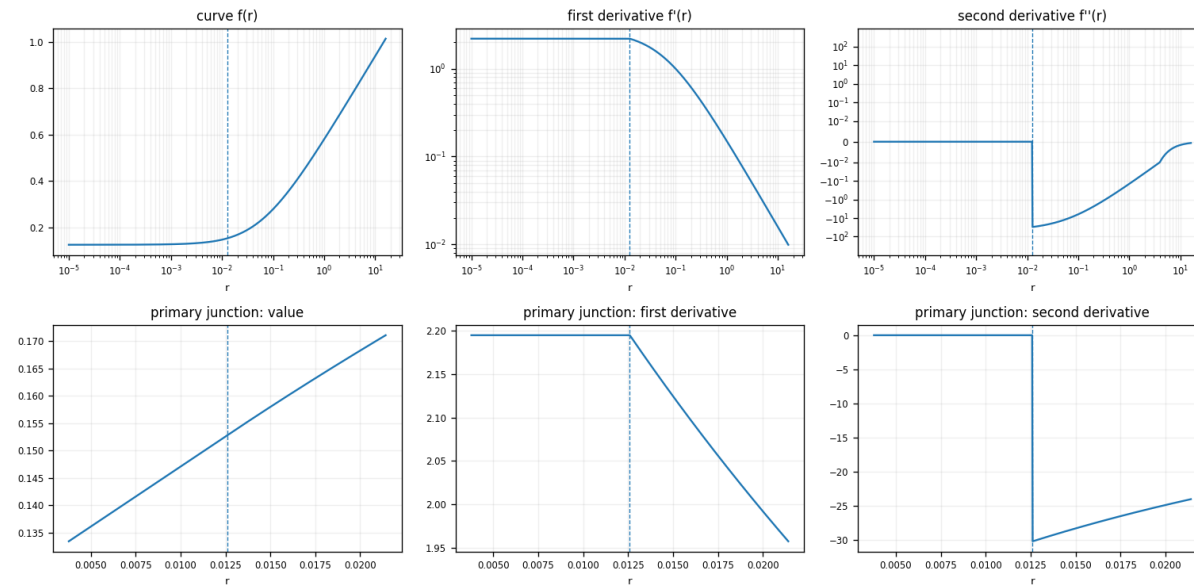
Canon Log 3
