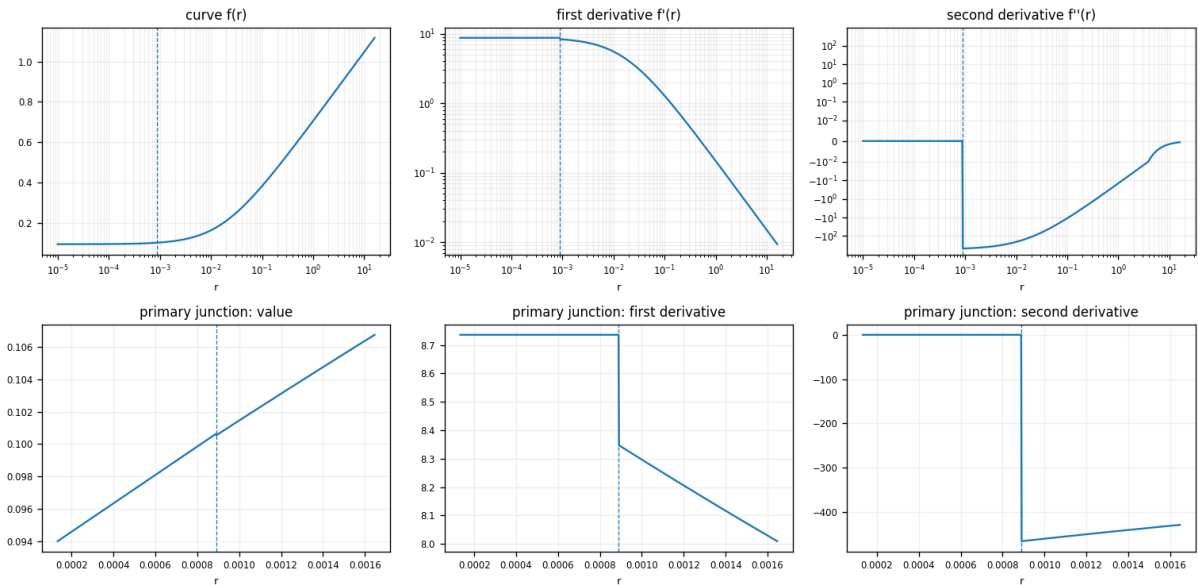
FUJIFILM F-Log
