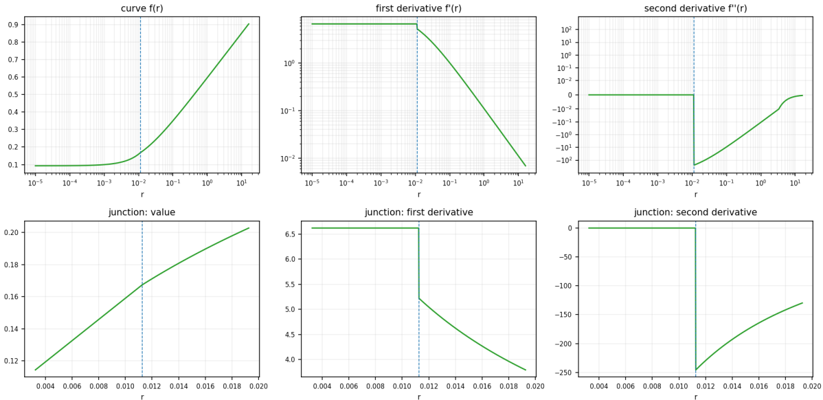
Sony S-Log3
