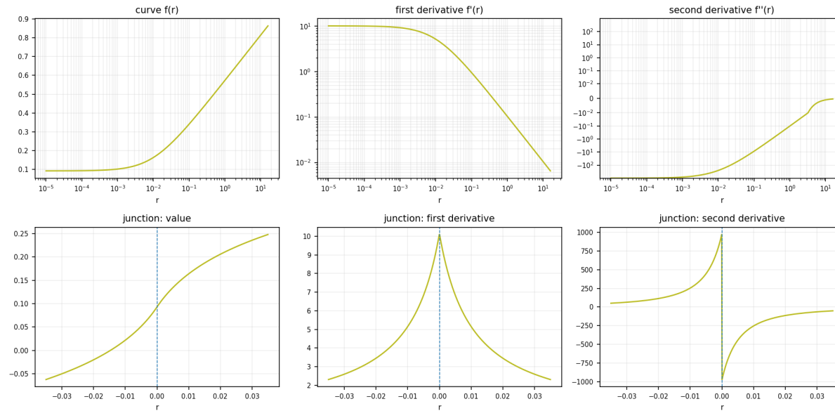
Canon Log 2
