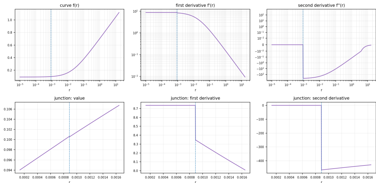
FUJIFILM F-Log
