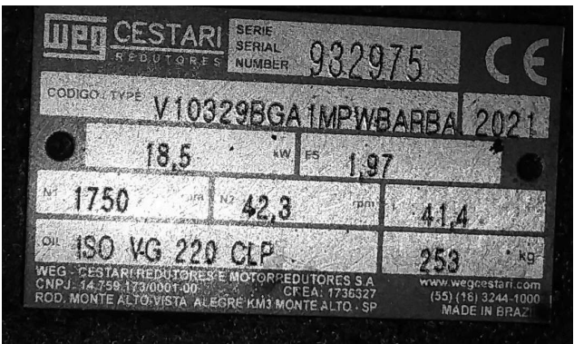
PLACA DE IDENTIFICAÇÃO
