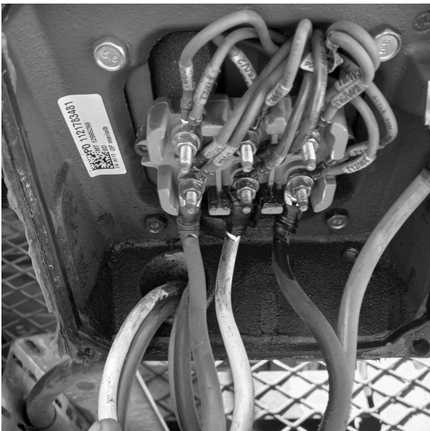
LIGAÇÃO ELETRICA MOMENTO DESMONTAGEM
