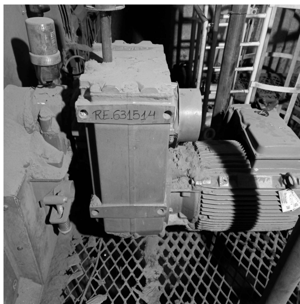
EQUIPAMENTO MONTADO - CX DE LIGAÇÃO MONTADA PARA LADO DIREITO (OLHANDO ATRAS DO MOTOR)
