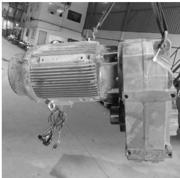
EQUIPAMENTO MOMENTO CHEGADA OFCINA
