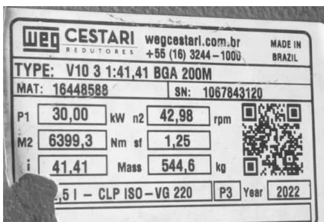
PLACA IDENTIFICAÇÃO ENVIADA PELO CLIENTE
