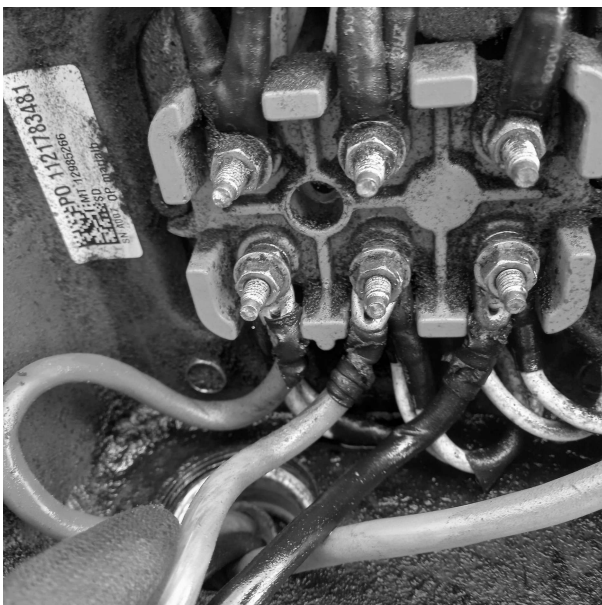
LIGAÇÃO ELÉTRICA MOMENTO DESMONTAGEM
