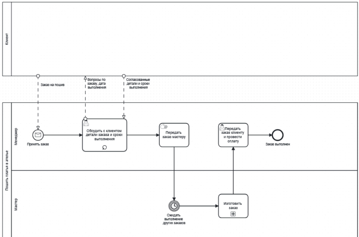
Рисунок 1 – Модель процесса «Пошить платье в ателье»
