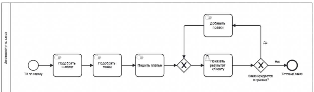
Рисунок 2 – Модель подпроцесса «Изготовить заказ»
