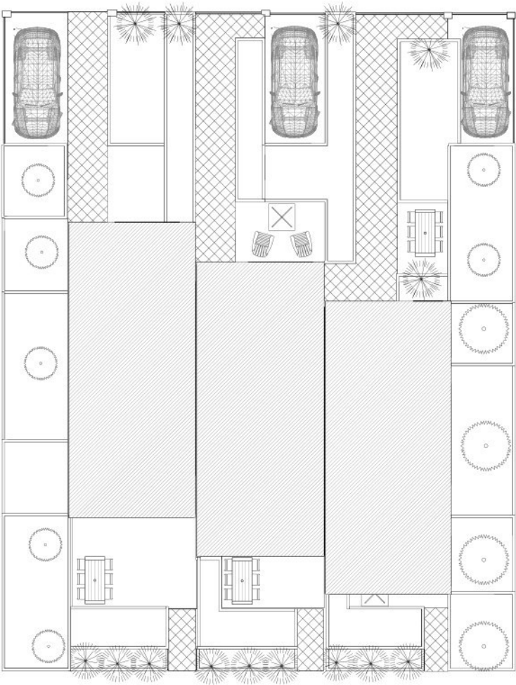
SITE PLAN SC 1:100
