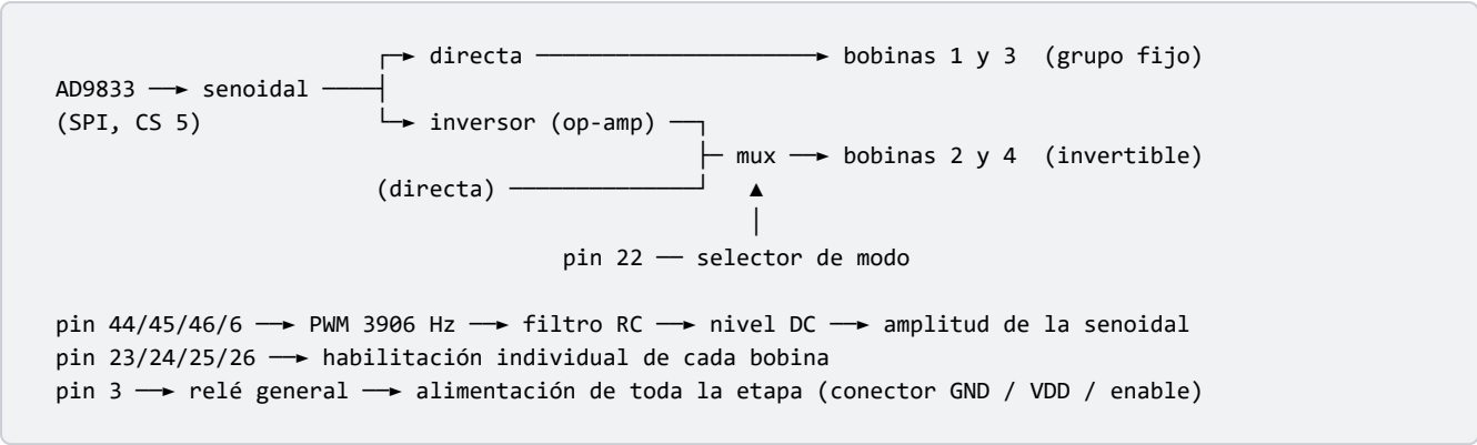
Figura 2. Cadena de señal desde la placa de control hasta las bobinas.
