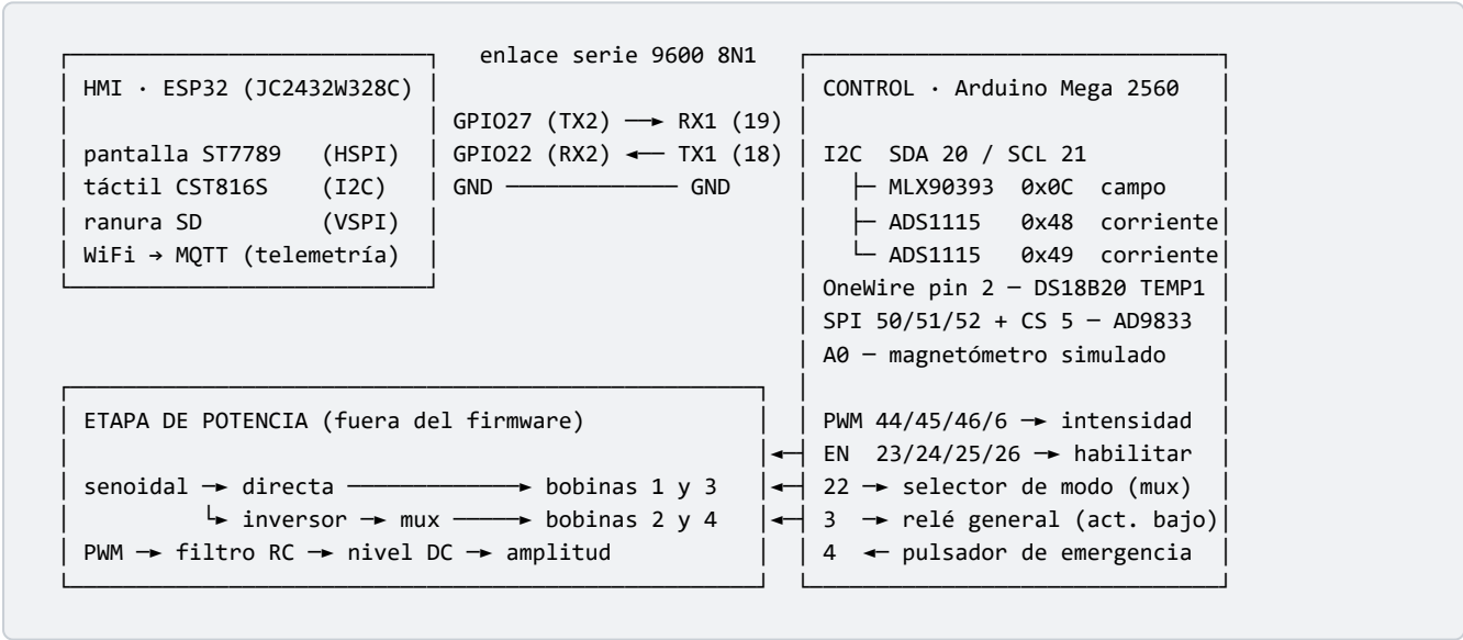
Figura 1. Diagrama de bloques del sistema con los pines que utiliza cada interfaz.
