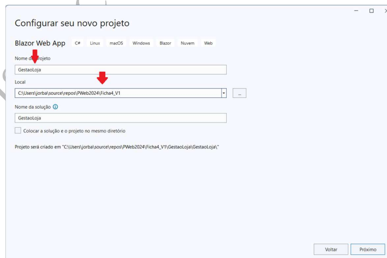
Figura 2- Configurações do projecto Blazor Web App – Passo Intermédio
