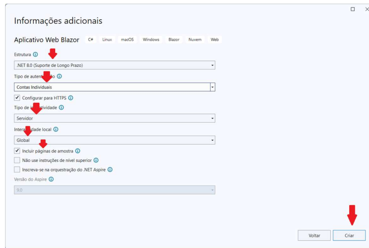
Figura 3- Configurações do projecto Blazor Web App – Passo Final
