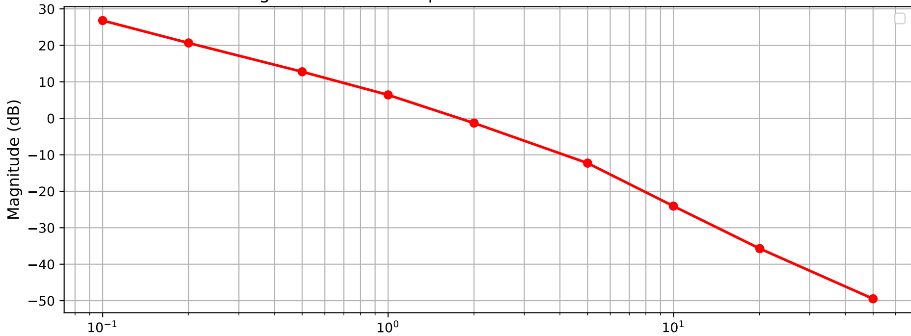
Diagrama de Bode Experimental Geométrico - Eixo Pitch
