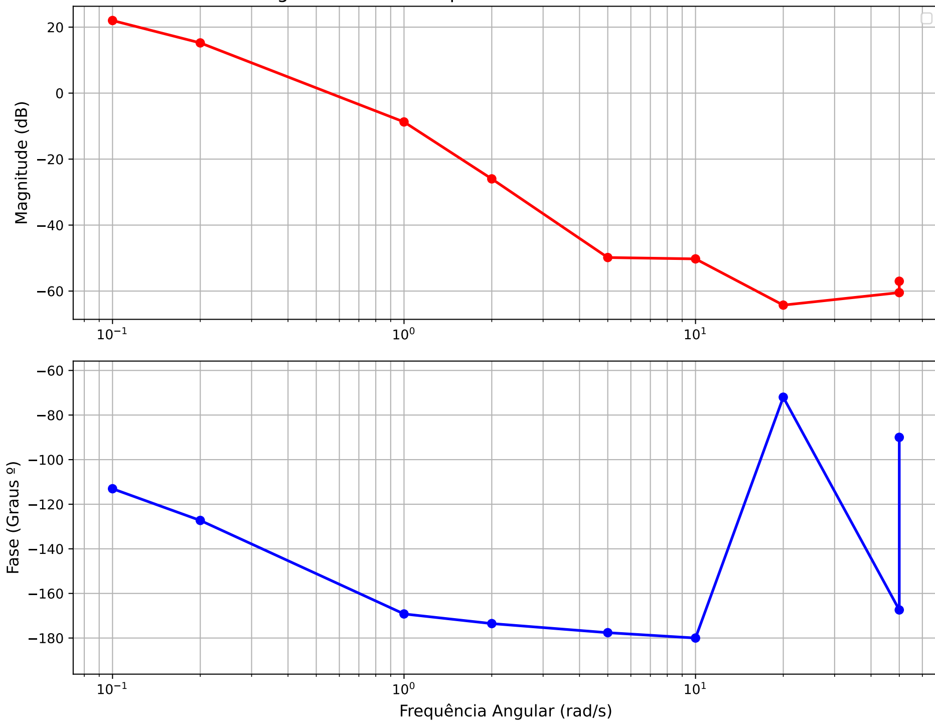
Diagrama de Bode Experimental Geométrico - Eixo Yaw
