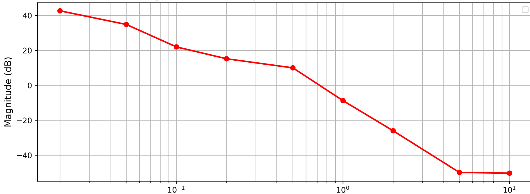
Diagrama de Bode Experimental Geométrico - Eixo Yaw
