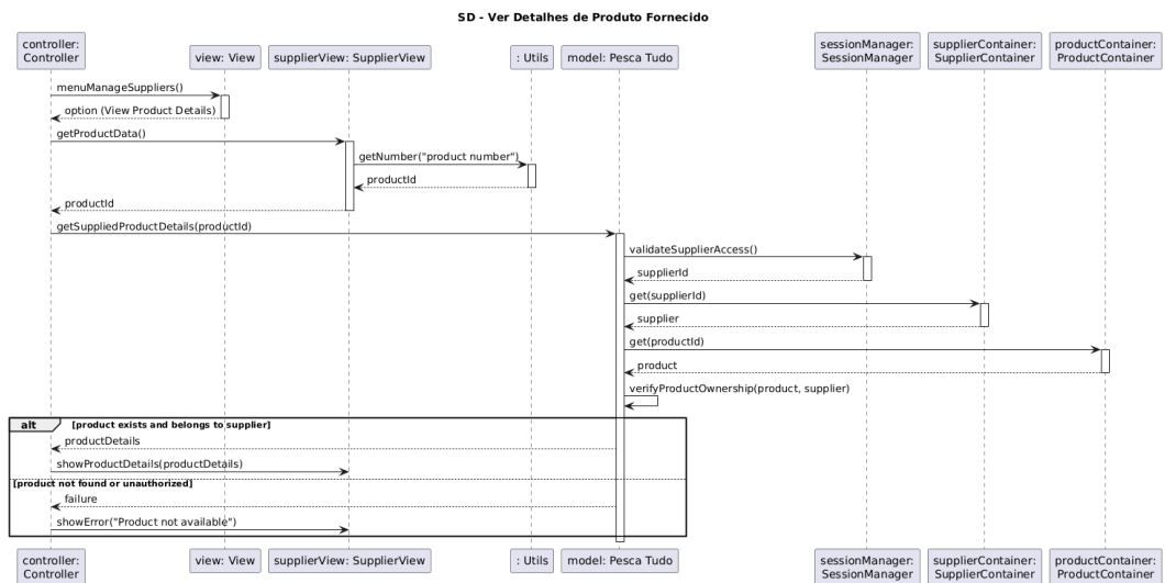
Figura 10 - Ver Detalhes de Produtos Fornecidos
