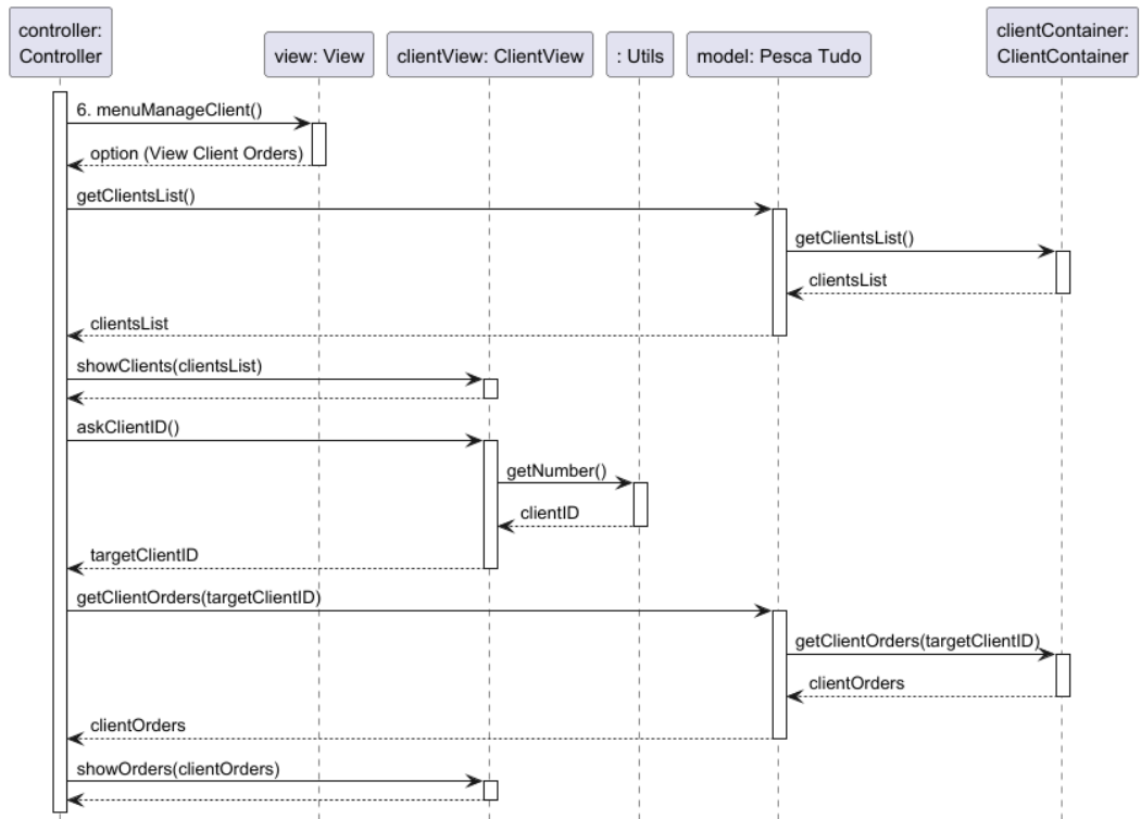
Figura 17 - Encomenda dos Clientes
