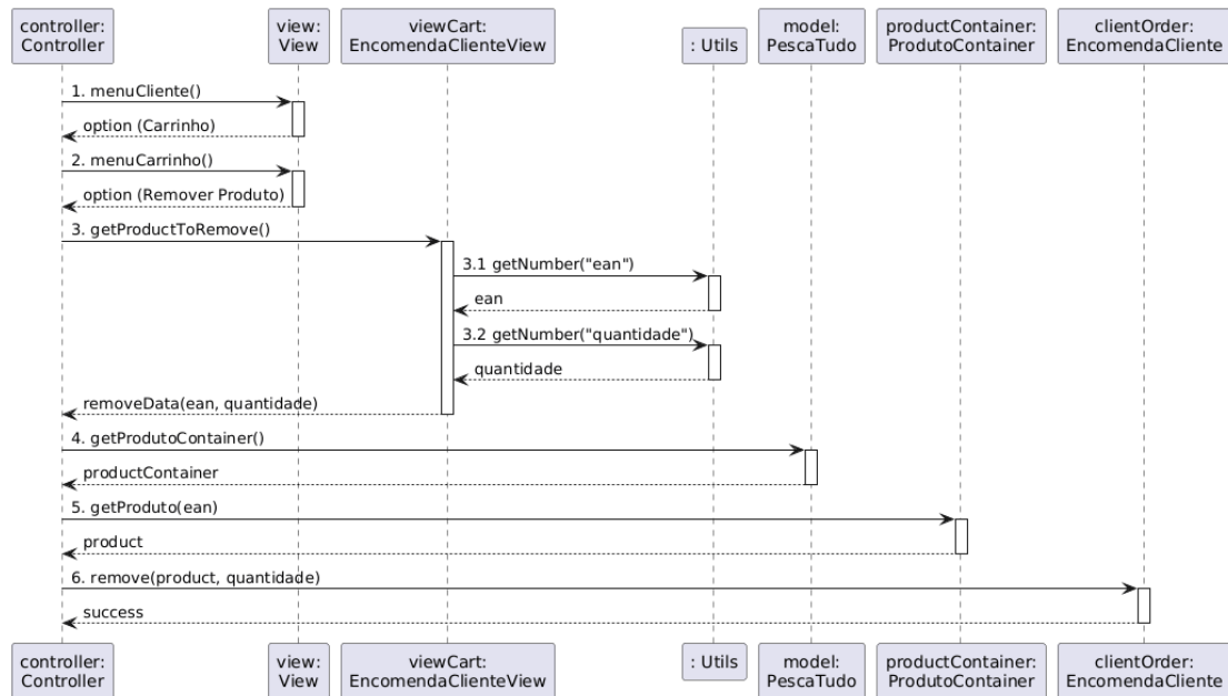
Figura 21 -Eliminar produto do carrinho
