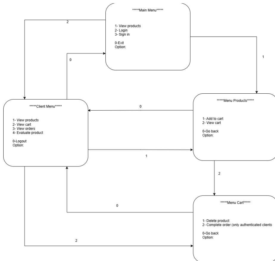
Figura 30 - User Interface do cliente
