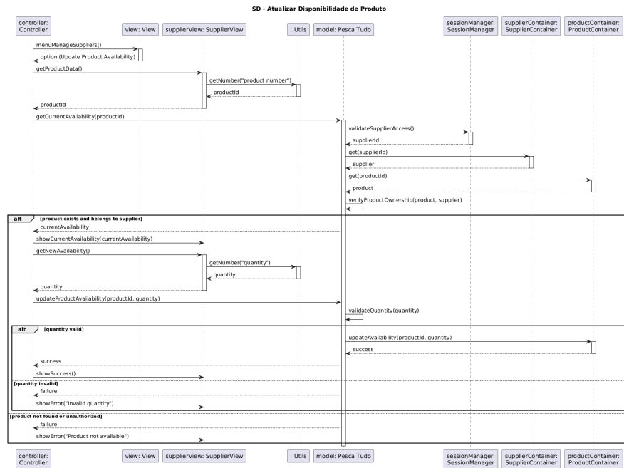
Figura 11 - Atualizar Disponibilidade do Produto
