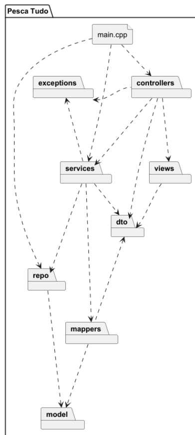
Figura 3 - Organização do código
