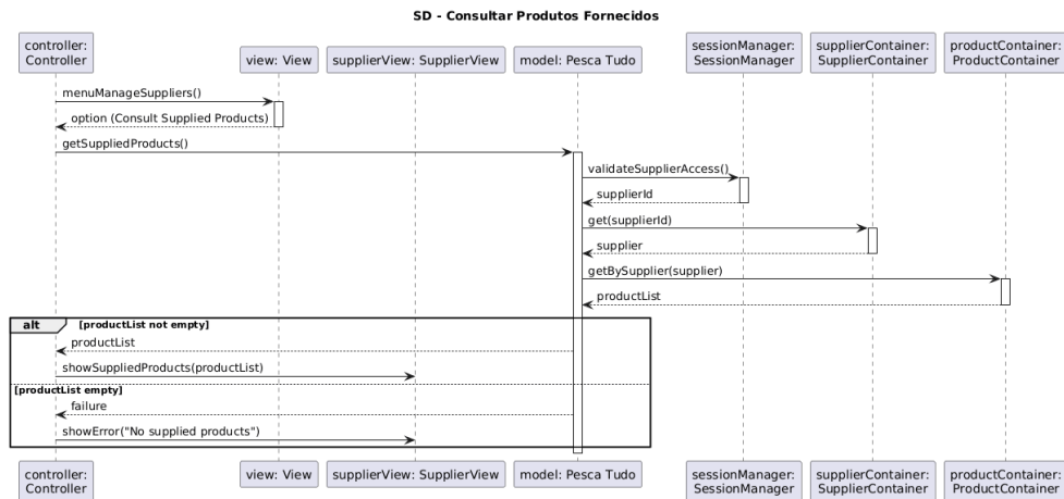
Figura 9 - Consultar Produtos Fornecidos
