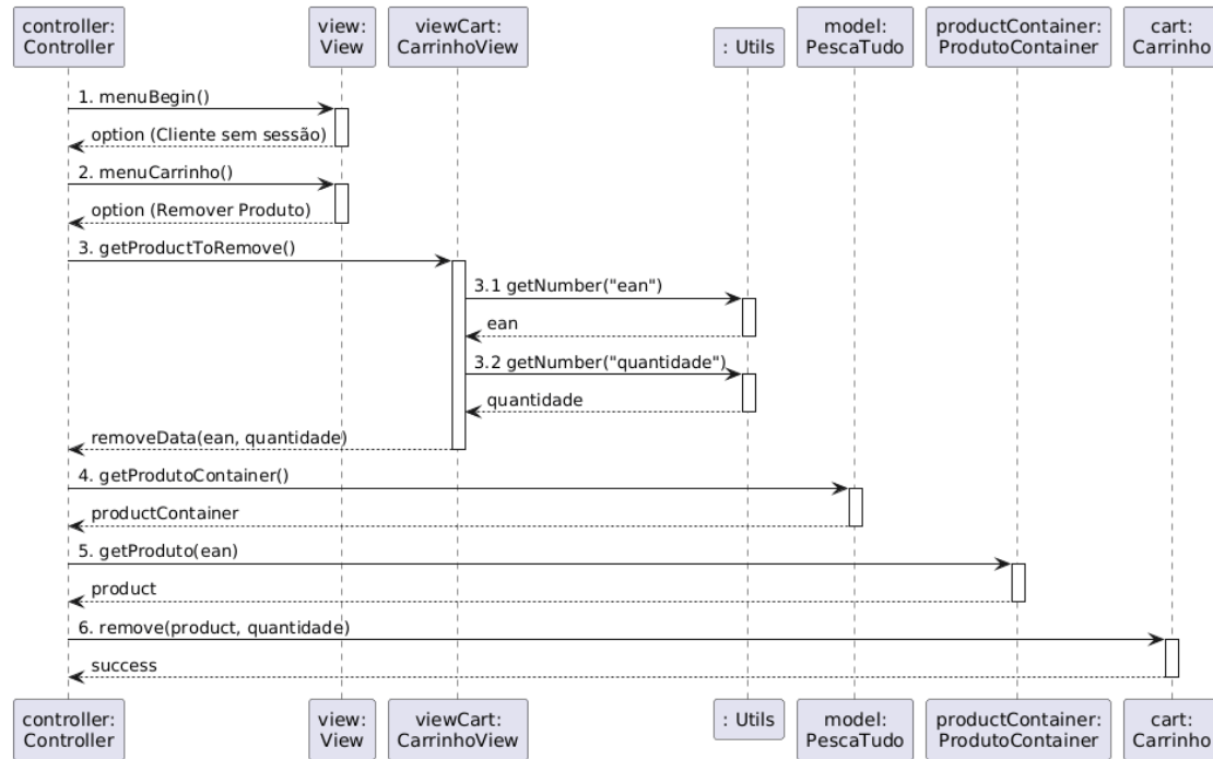
Figura 29 - Eliminar produto do carrinho
