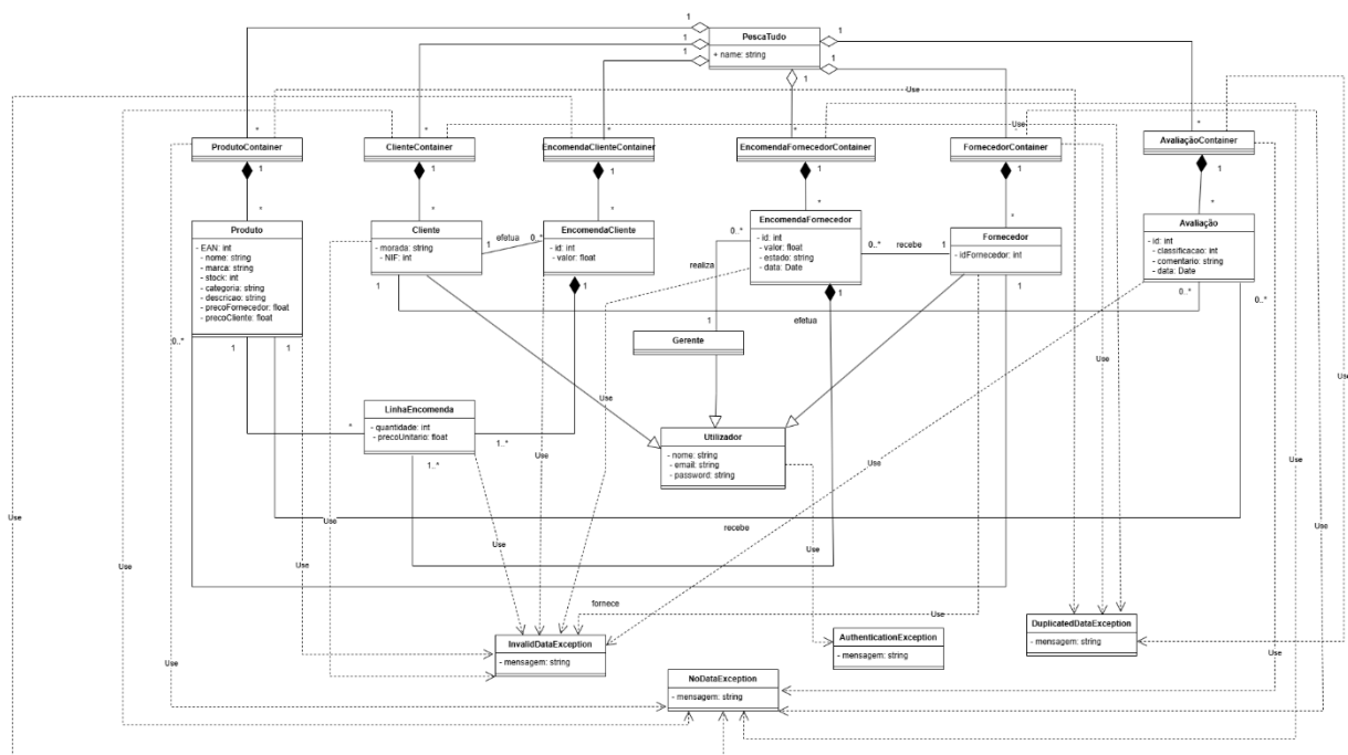
Figura 4 - Diagrama do modelo de classes
