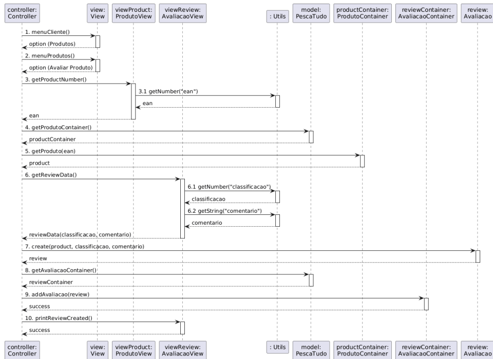
Figura 25 - Adicionar avaliação ao produto
