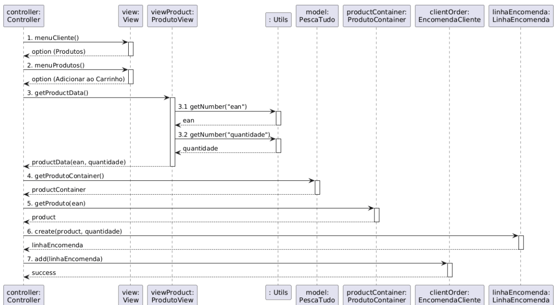
Figura 20- Adicionar produto ao carrinho
