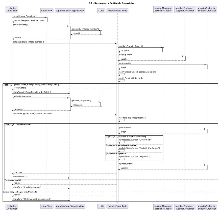
Figura 14 - Responder a Pedido de Reposição
