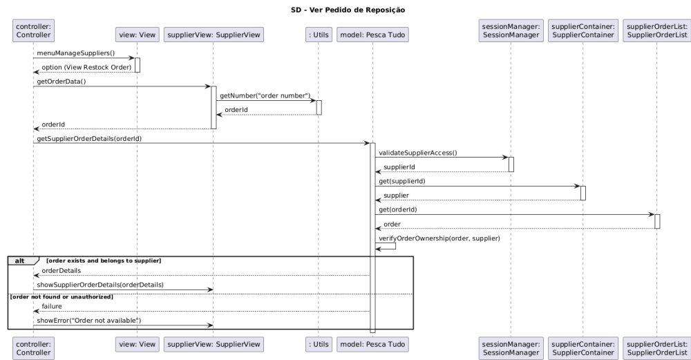
Figura 13 - Ver Pedidos de Reposição
