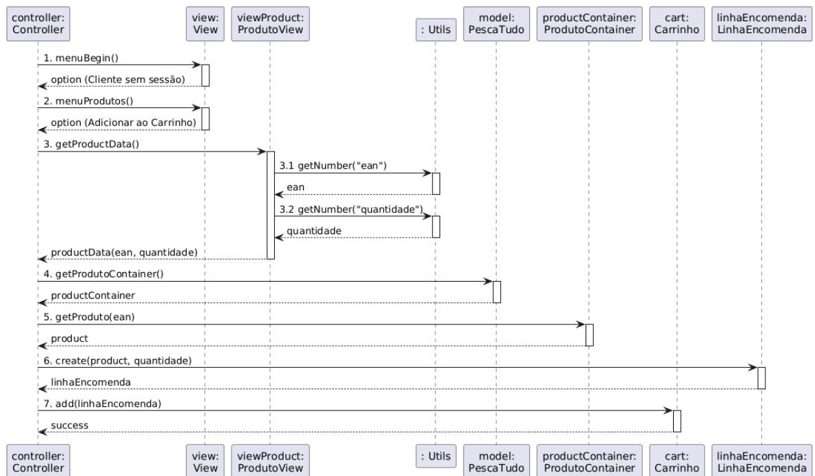
Figura 28 - Adicionar produto ao carrinho
