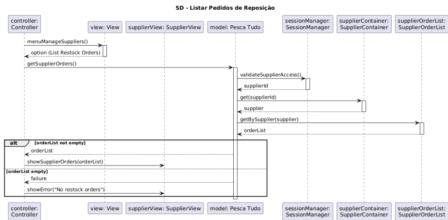
Figura 12 - Listar Pedidos de Reposição
