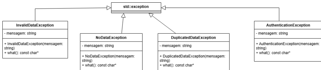
Figura 5 - Diagrama de classes de exceções
