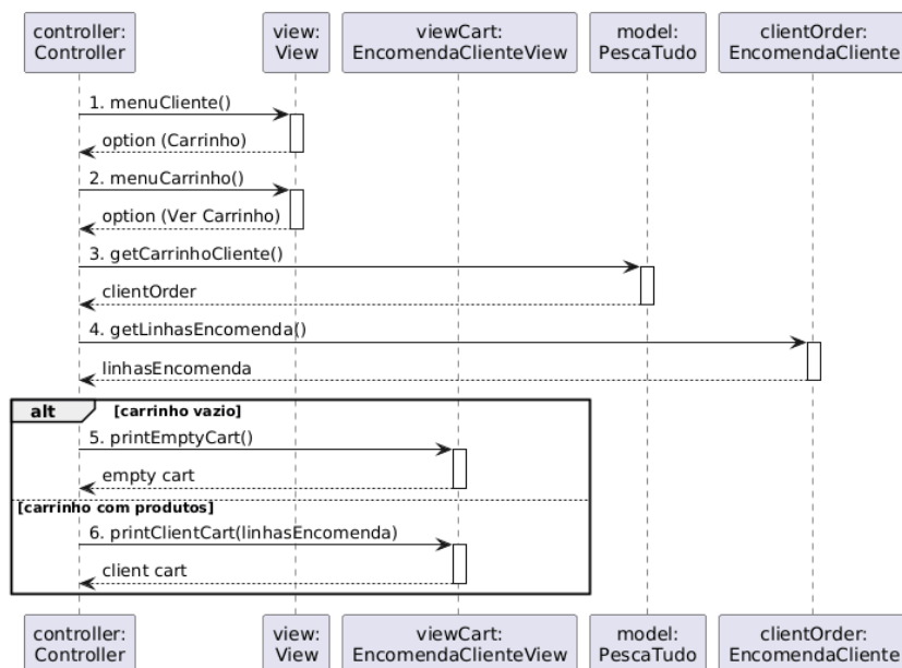
Figura 22 - Ver produtos no carrinho
