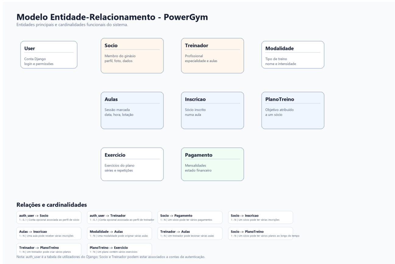
Figura 1 - Diagrama entidade-relacionamento do PowerGym.
