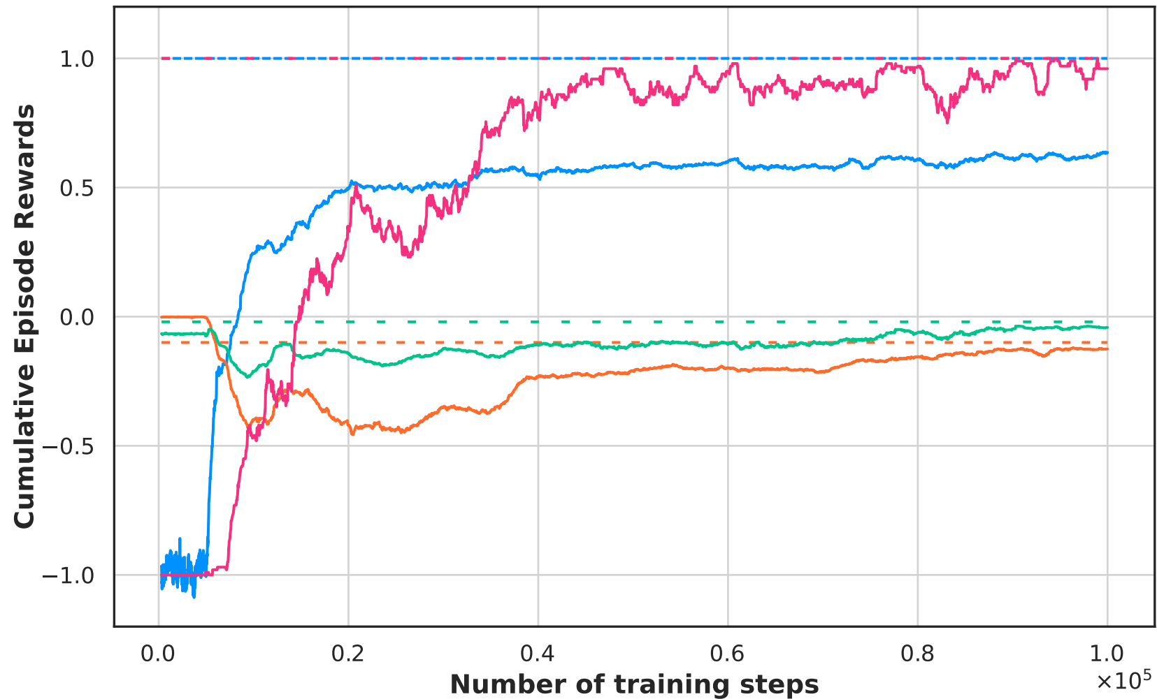
LunarLander-v2
