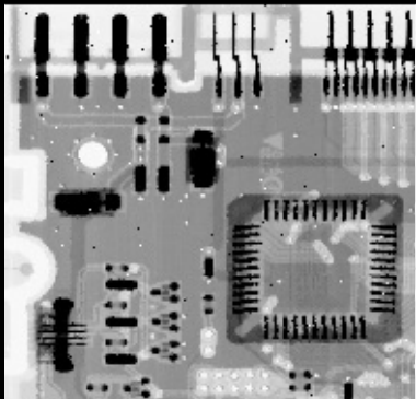
Mediana 3x3
