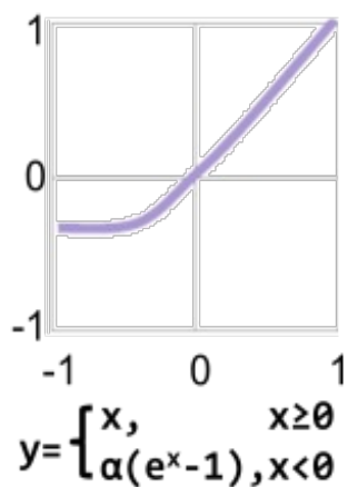
Exponential LU
