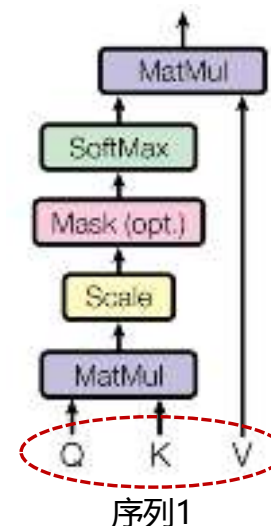
自注意力
