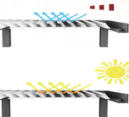
Угол поворота ламели 107°
