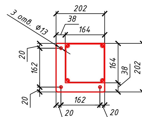
Опорные площадки колонн
