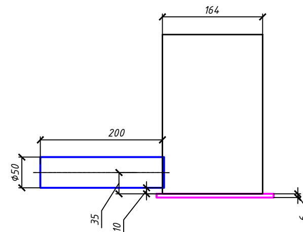
Сливные патрубки \Phi 50
