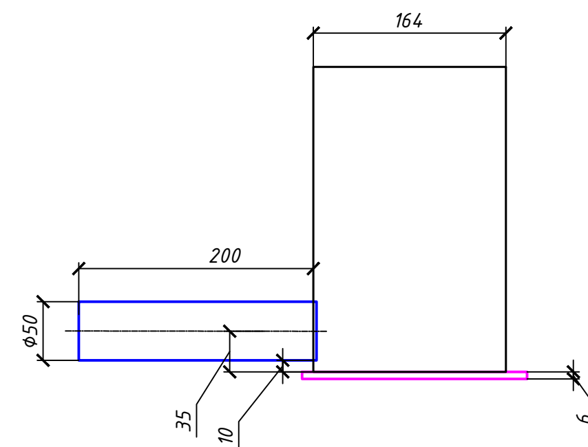
Сливной патрубок \phi 50 для колонны 3360 мм
