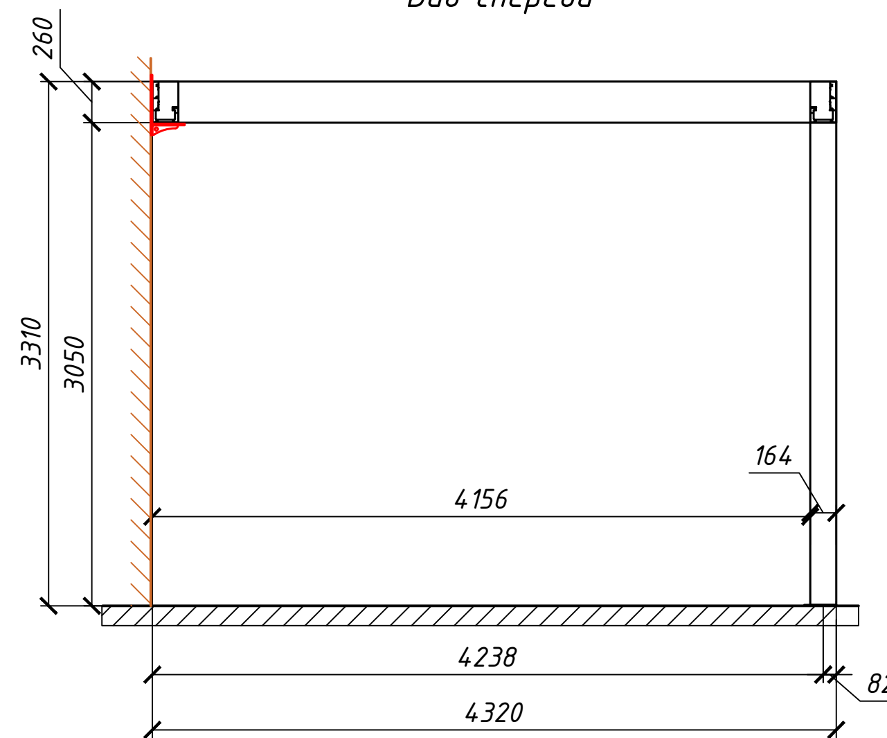
Вид спереди
