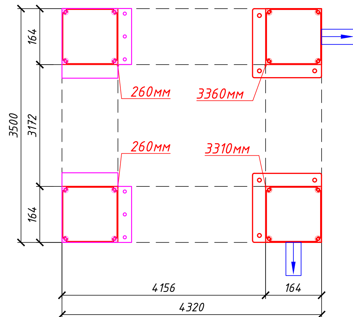
Схема опорных площадок колонн
