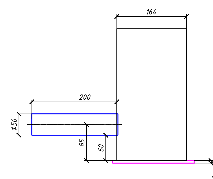
Сливной патрубок \phi 50 для колонны 3360 мм
