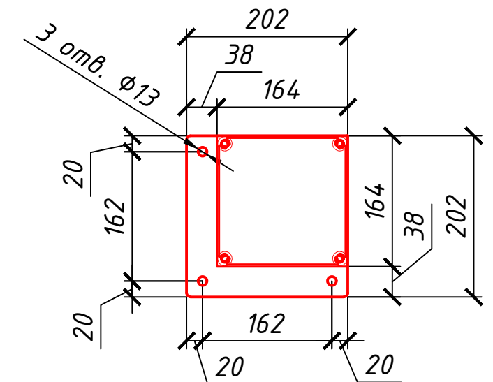
Опорные площадки колонн
