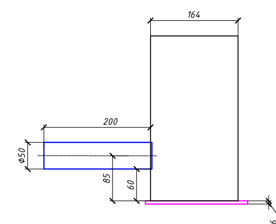
Сливной патрубок Ø50 для колонны 3360 мм
