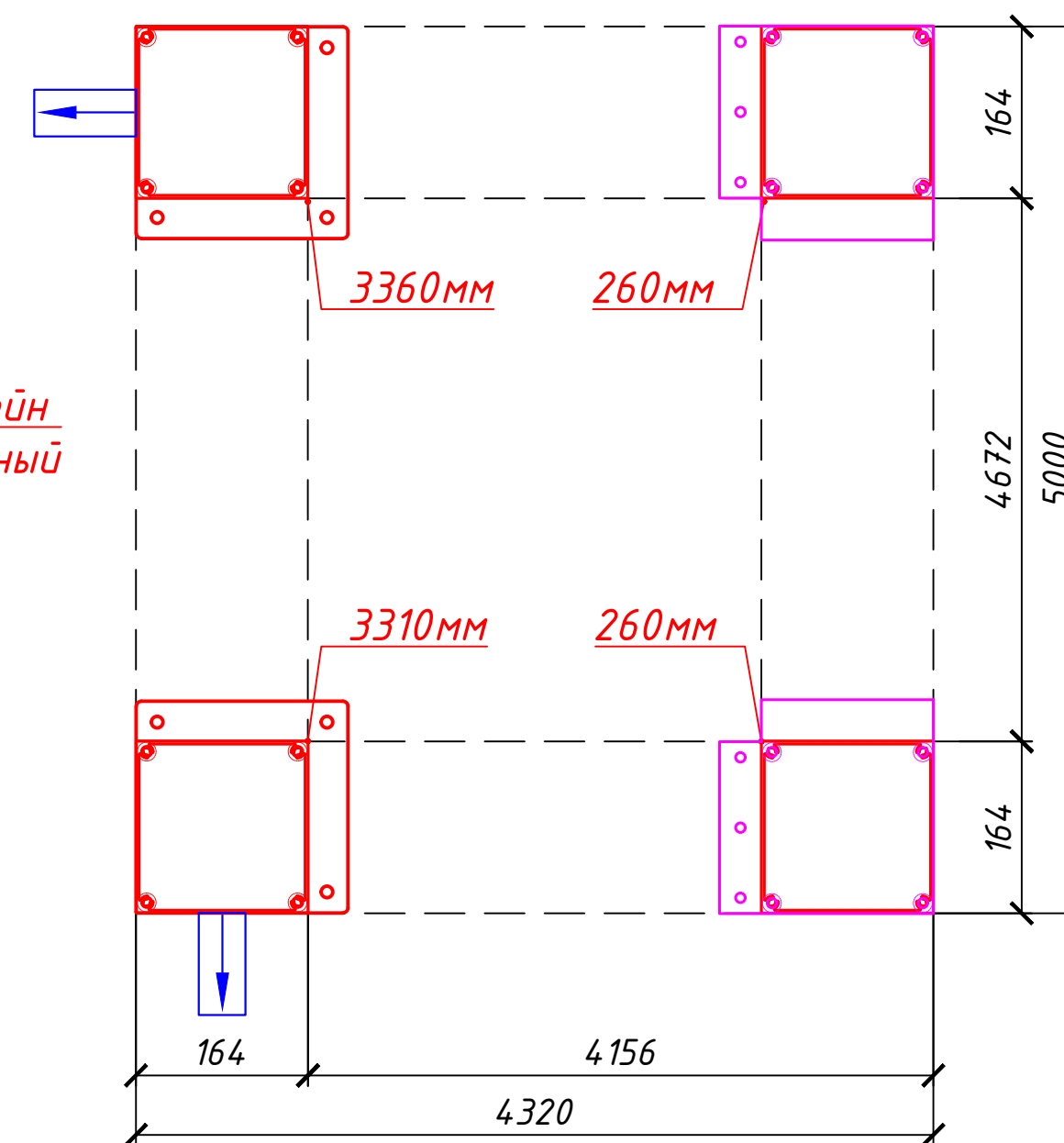
Схема опорных площадок колонн
