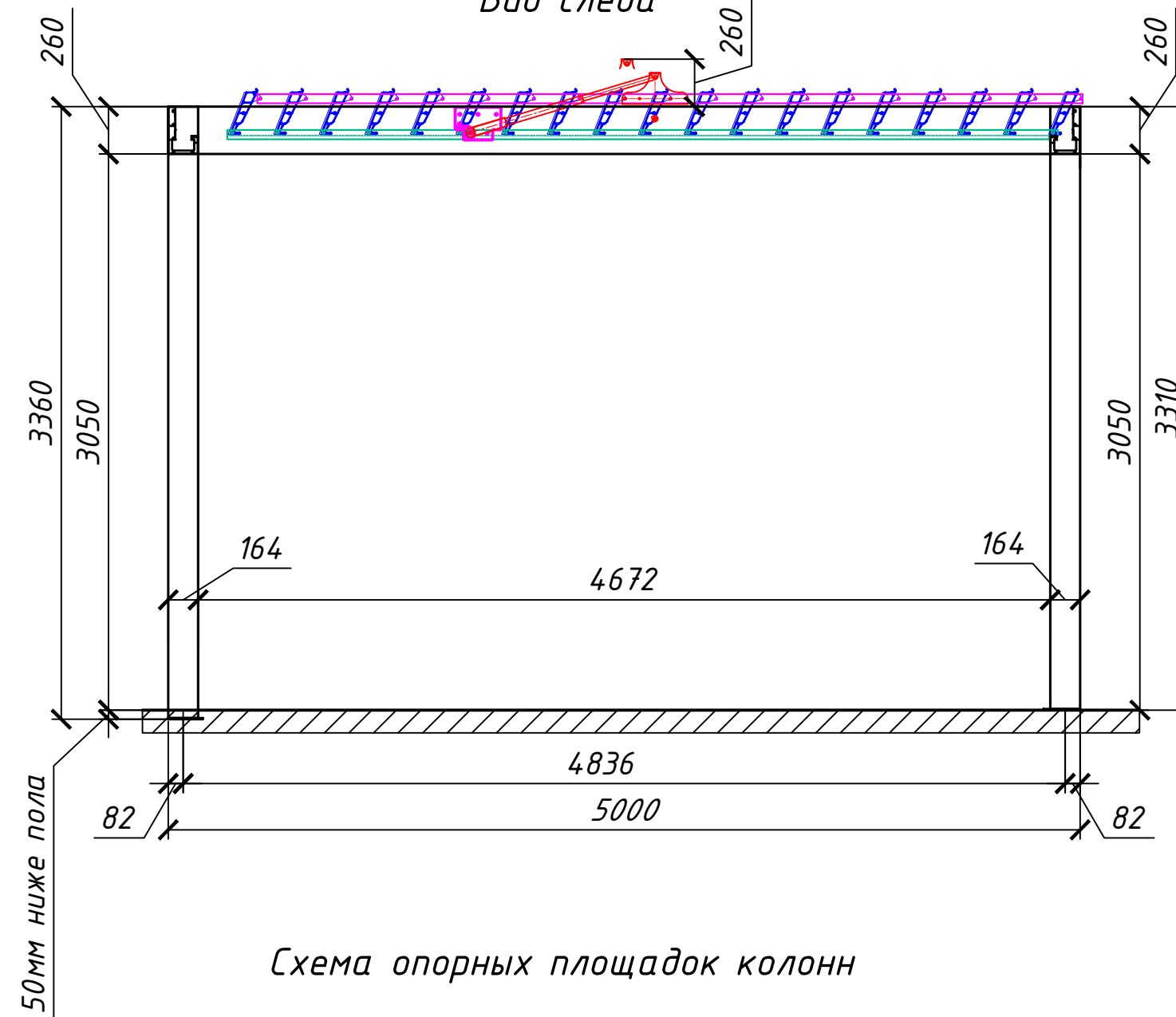
Вид слева
