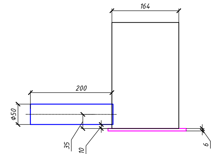
Сливной патрубок Ø50 для колонны 3360 мм
