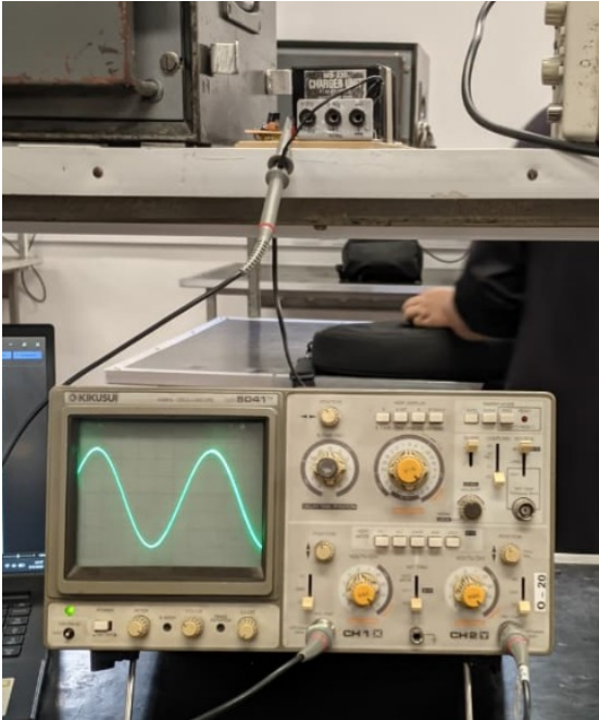
Figura 16. Señal del generador de funciones de la fuente
