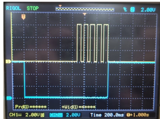
Figura 27. Señal del interruptor junto al tren de pulsos del discado
