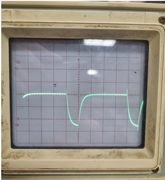
Figura 24. Señal en modo suma con inversión
