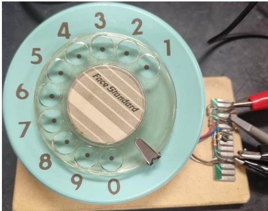
Figura 25. Conexión del teléfono de disco rotativo al osciloscopio y energía
