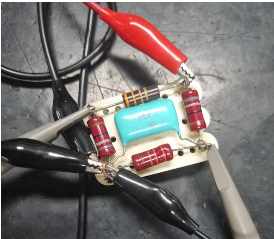
Figura 23. Circuito auxiliar
