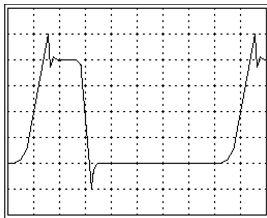
Figura 29. Señal en x10 con acoplamiento en CA
