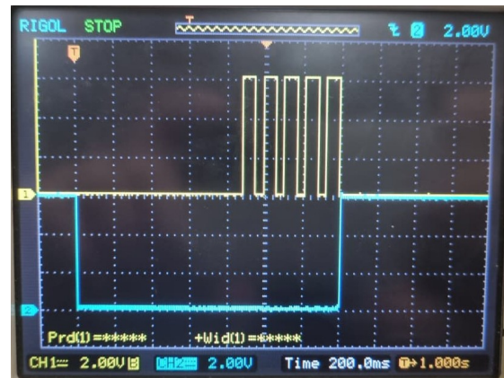
Figura 23. Señal del interruptor junto al tren de pulsos del discado
