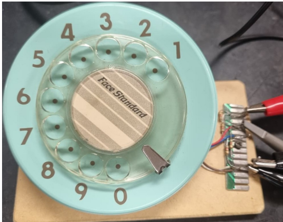
Figura 21. Conexión del teléfono de disco rotativo al osciloscopio y energía
