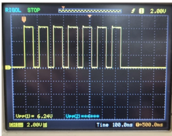
Figura 22. Señal generada al marcar el número 7
