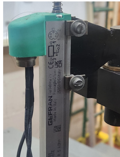
Figura 1. Imagen 1 de la máquina universal de ensayo.
