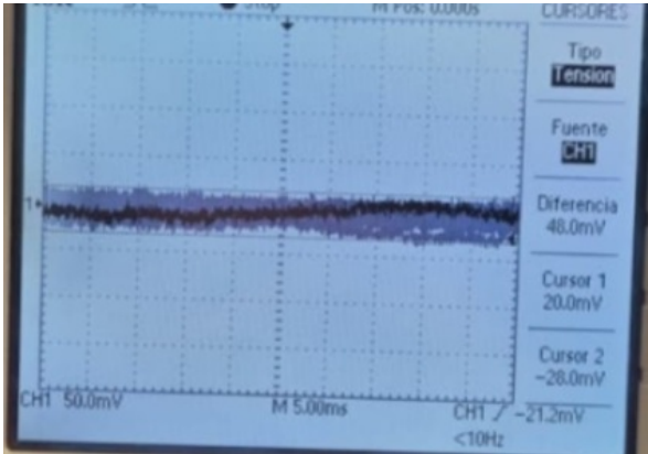
Figura 17. Celda de carga acoplada sin ruido.
