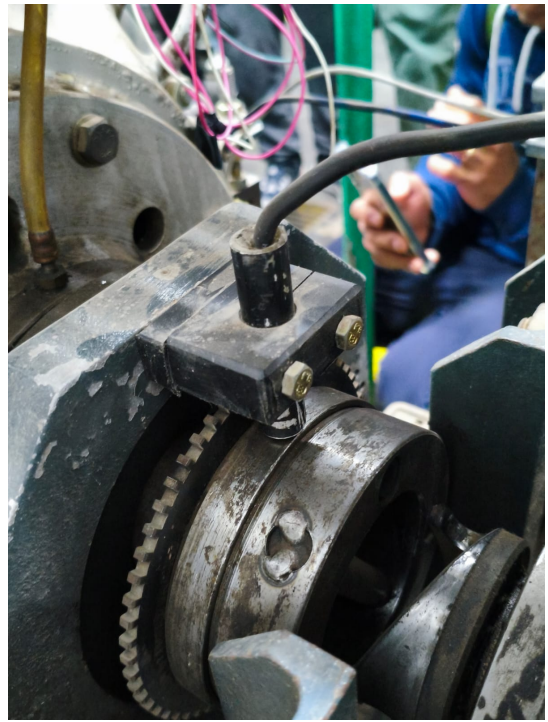
Figura 10. Sensor de velocidad magnético o inductivo.
