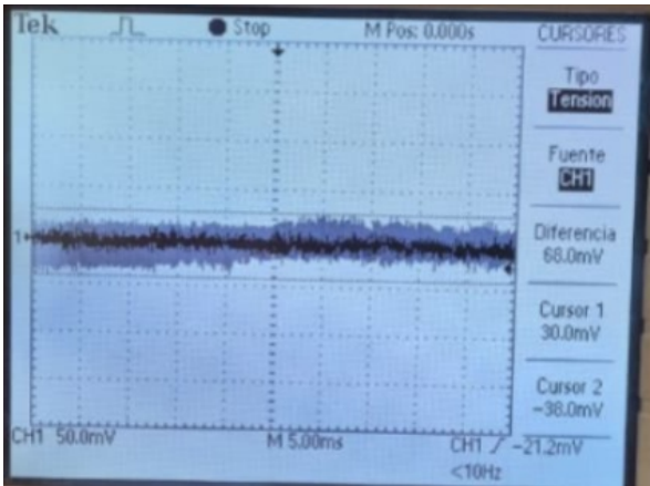
Figura 19. Celda de carga desacoplada sin ruido.
