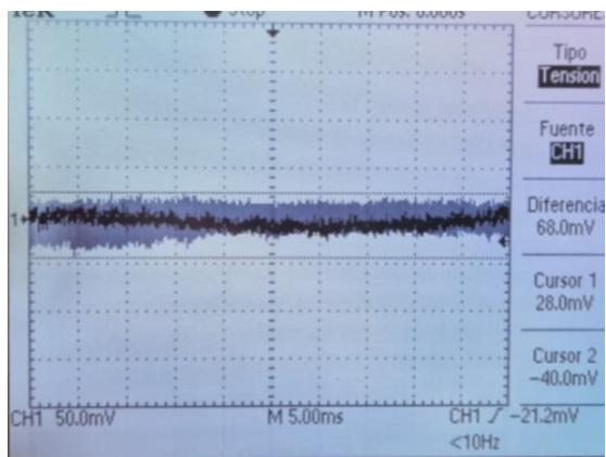
Figura 22. Celda de carga fuera del gabinete sin motor.
