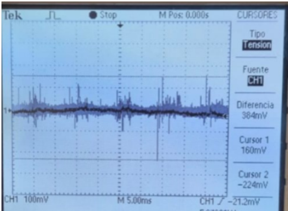
Figura 18. Celda de carga acoplada con ruido.
