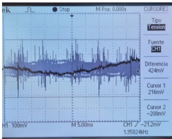
Figura 20. Celda de carga desacoplada con ruido.
