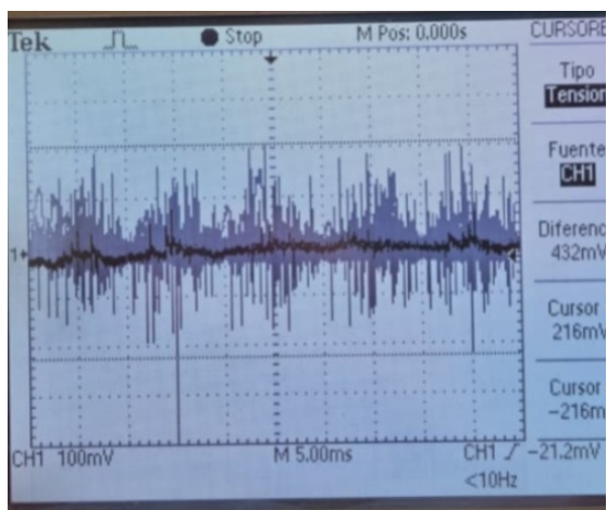
Figura 21. Celda de carga fuera del gabinete con motor encendido.
