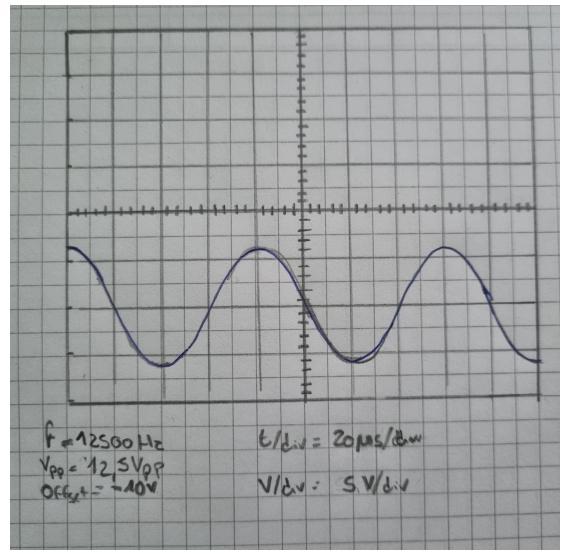
Figura 32. Señal Documentador
