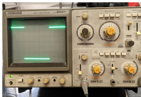
Figura 13. Señal cuadrada
