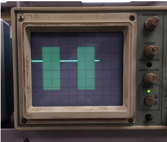
Figura 23. Señal de paquetes
