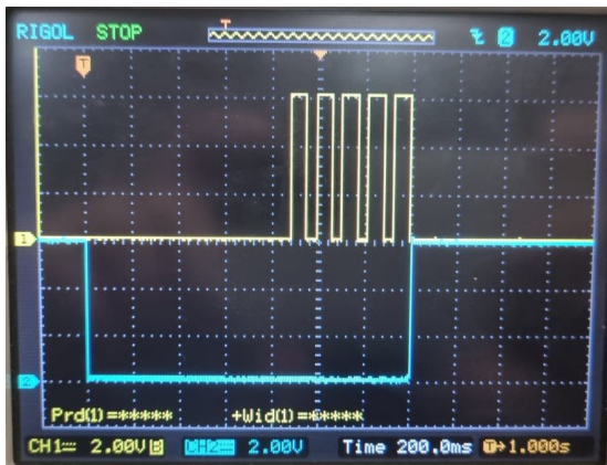
Figura 29. Señal del interruptor junto al tren de pulsos del discado
