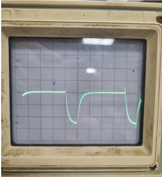
Figura 26. Señal en modo suma con inversión
