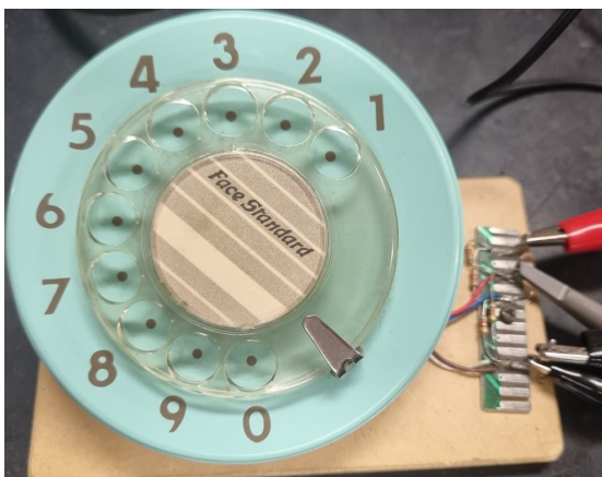
Figura 27. Conexión del teléfono de disco rotativo al osciloscopio y energía
