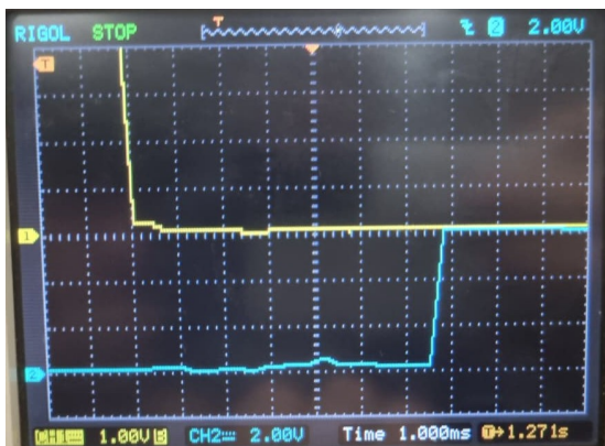
Figura 30. Demora del interruptor respecto al tren de pulsos
