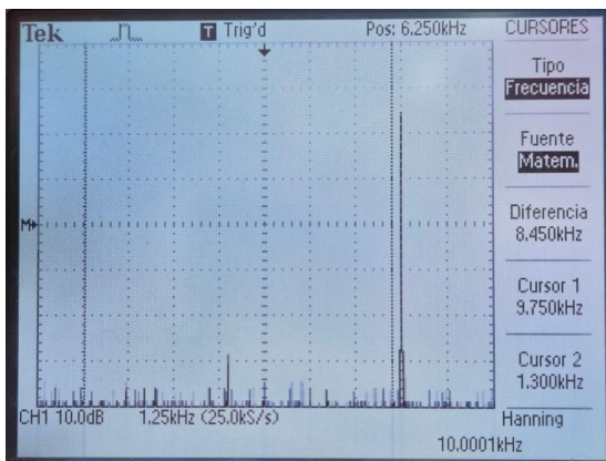
Figura 5. Señal de 10 kHz con frecuencia de muestreo de 25 kS/s
