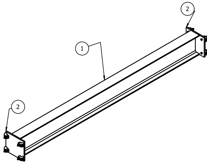
ISOMETRIC VIEW ESCALA:(1 : 25)
