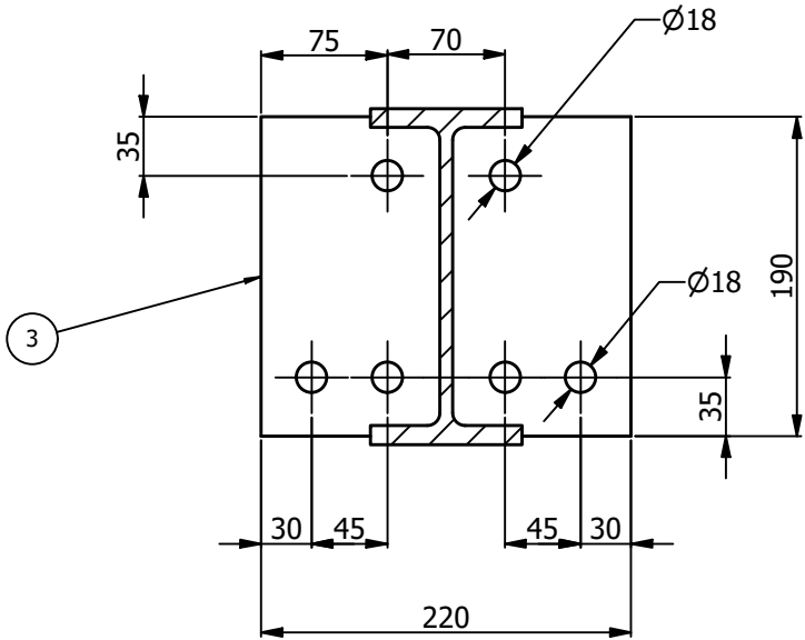
CUT A-A
