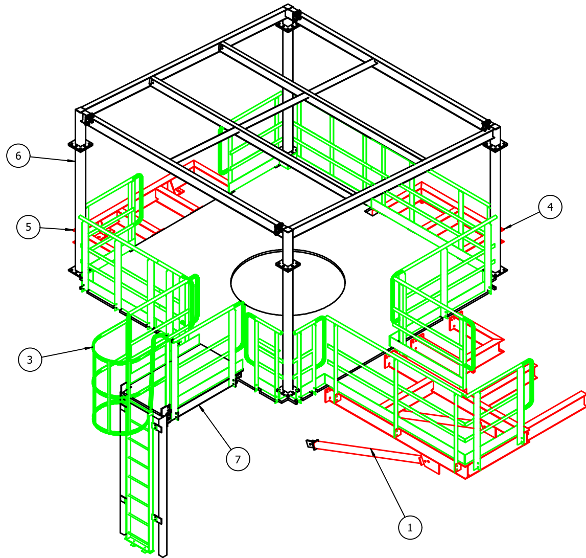
ISOMETRIC VIEW ESCALA:(1 : 50)
