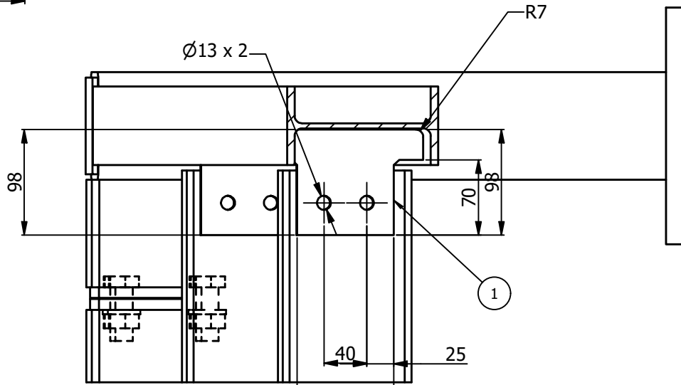
CUT EI-EI ESCALA:(1 : 5)
