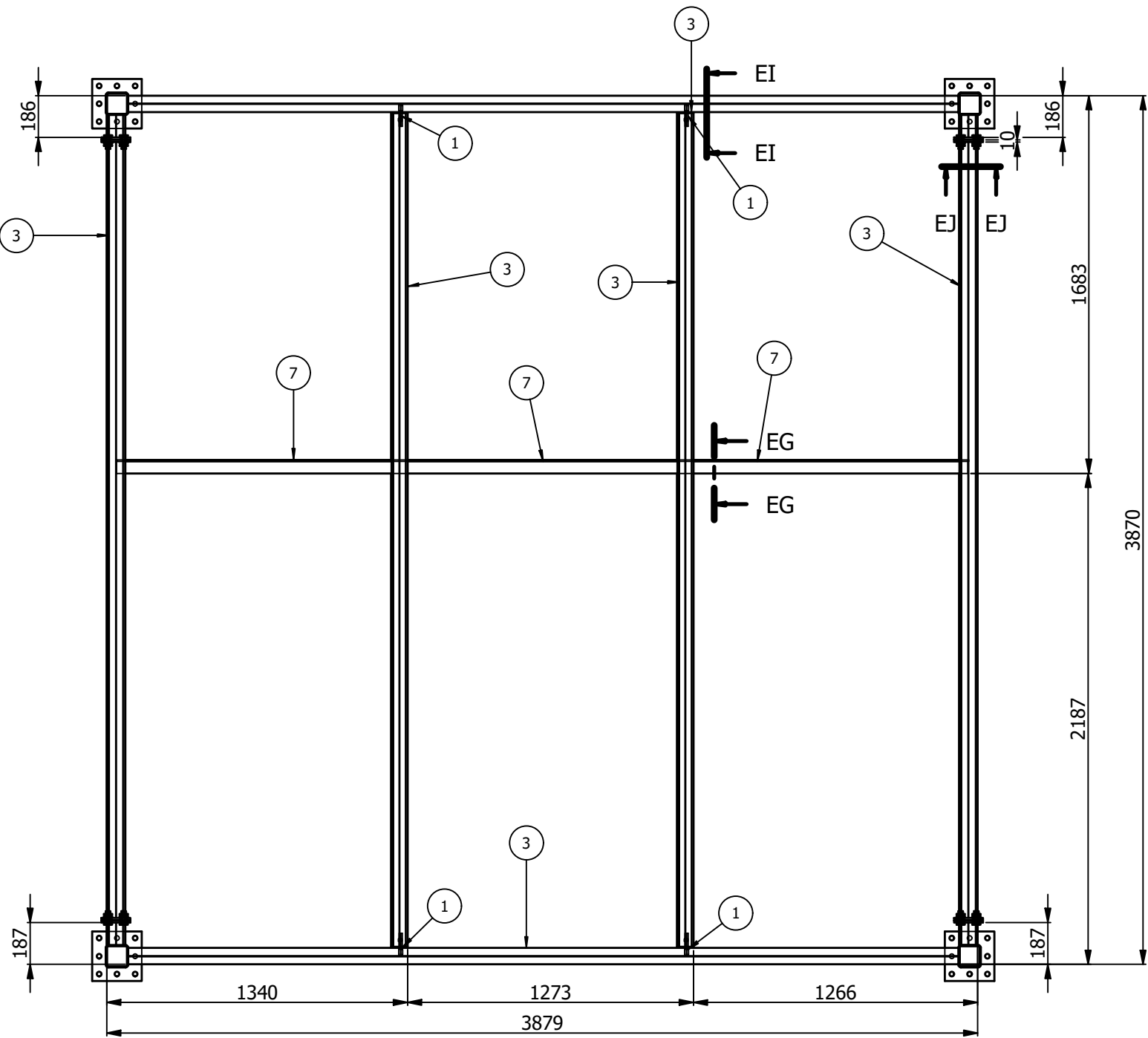
TOP VIEW ESCALA:(1 : 25)
