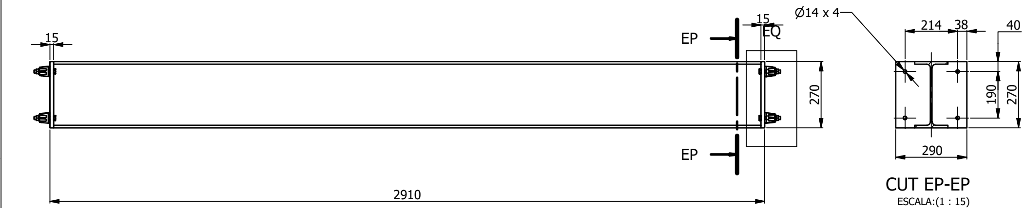
FRONT VIEW ESCALA:(1 : 15)
