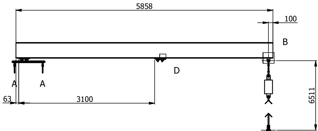
FRONT VIEW ESCALA:(1 : 50)
