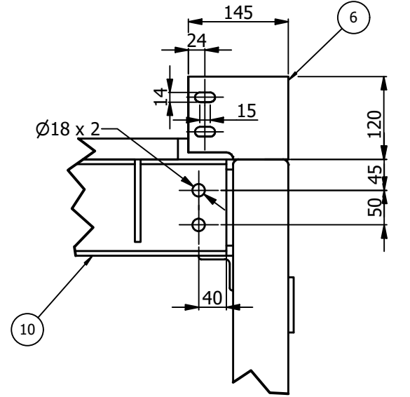
DETALLE ESCALA:(0,13 : 1)
