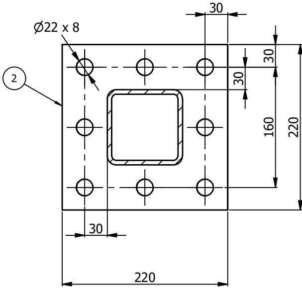
CUT A-A ESCALA:(1 : 5)
