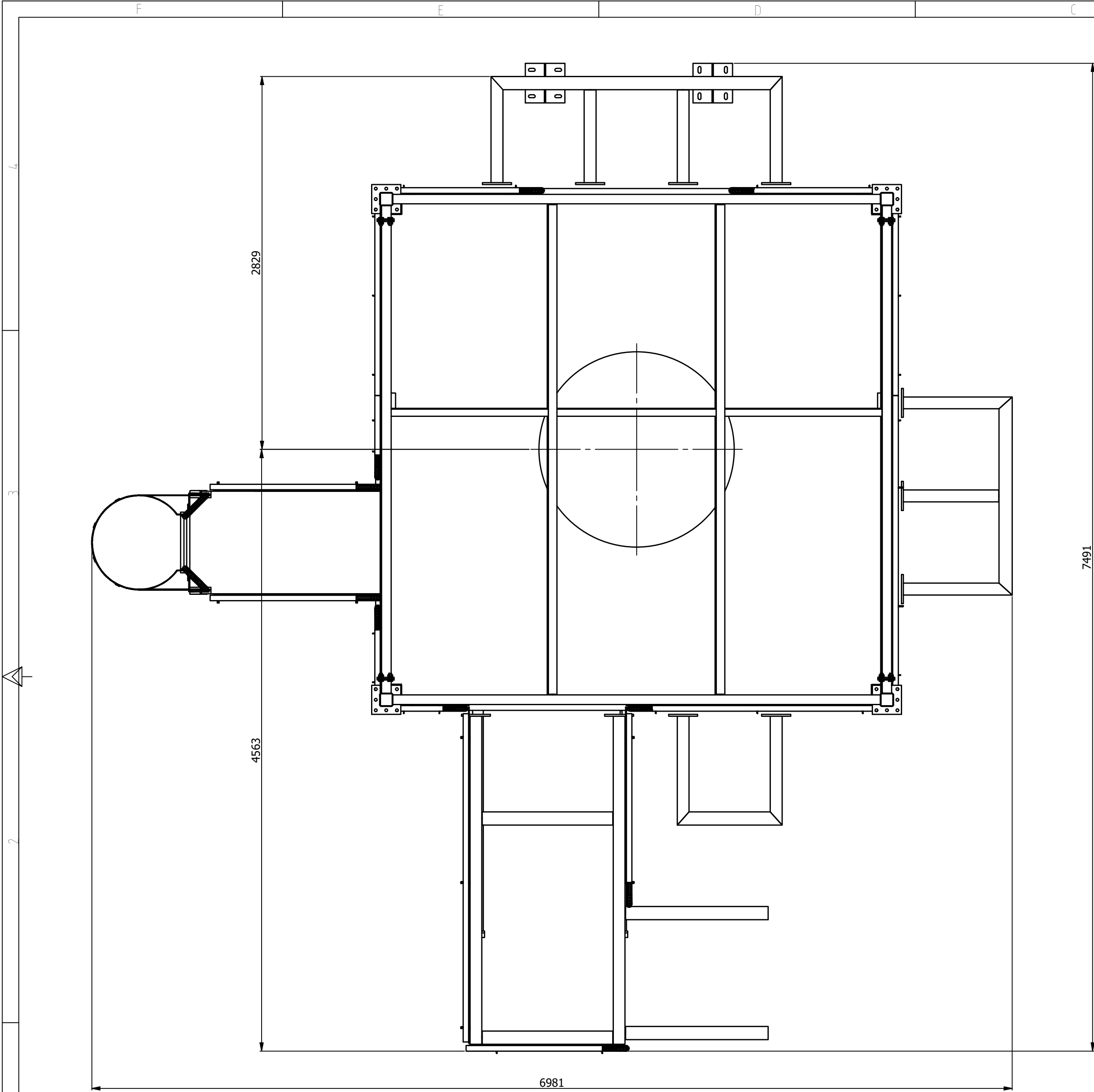
TOP VIEW ESCALA:(1 : 25)
