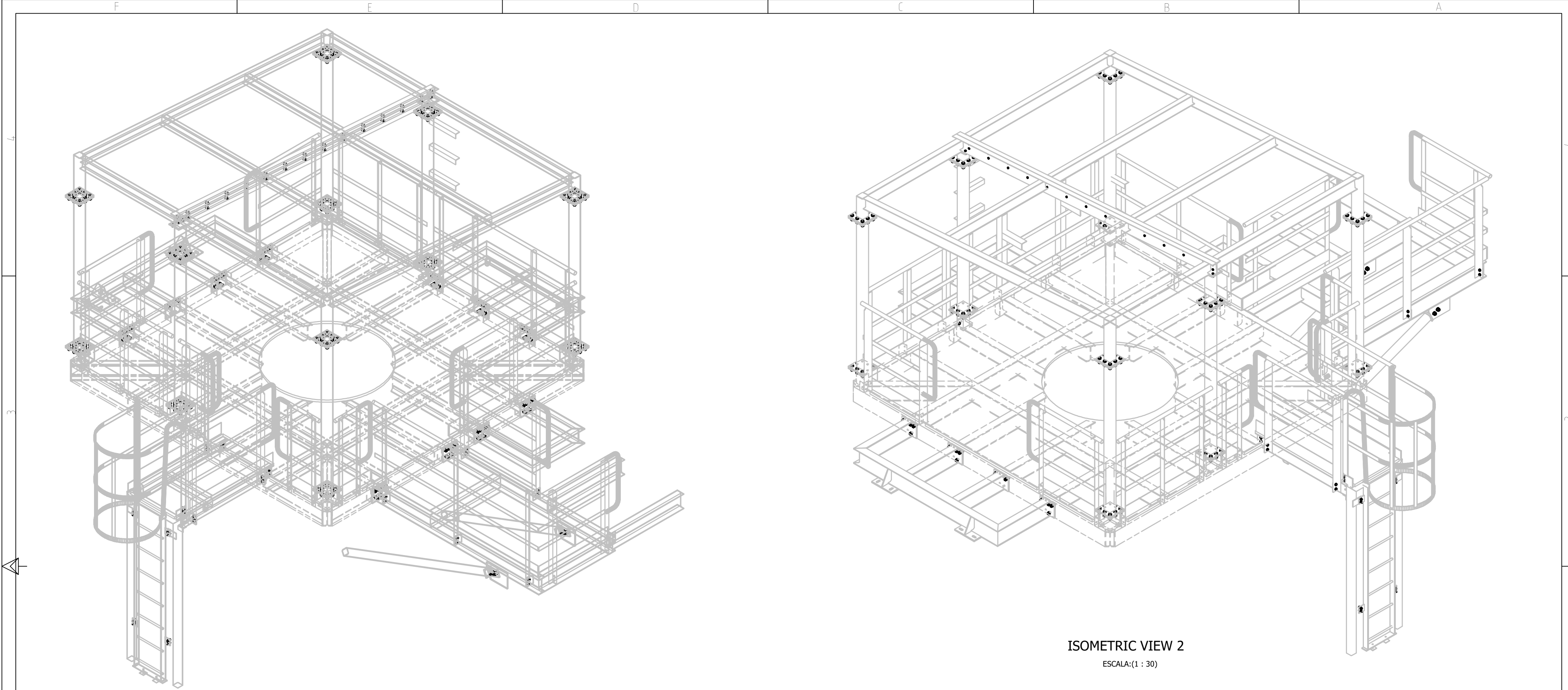
ISOMETRIC VIEW 1 ESCALA:(1 : 30)
