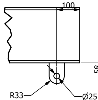
DETAIL EY ESCALA:(1 : 10)
