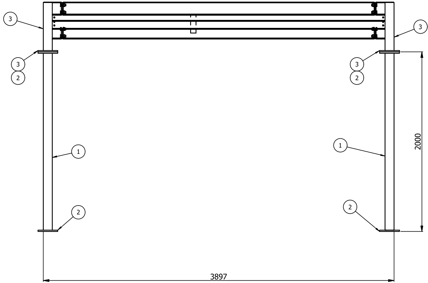
SIDE VIEW ESCALA:(1 : 25)
