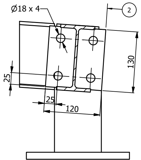
CUT EJ-EJ ESCALA:(1 : 5)
