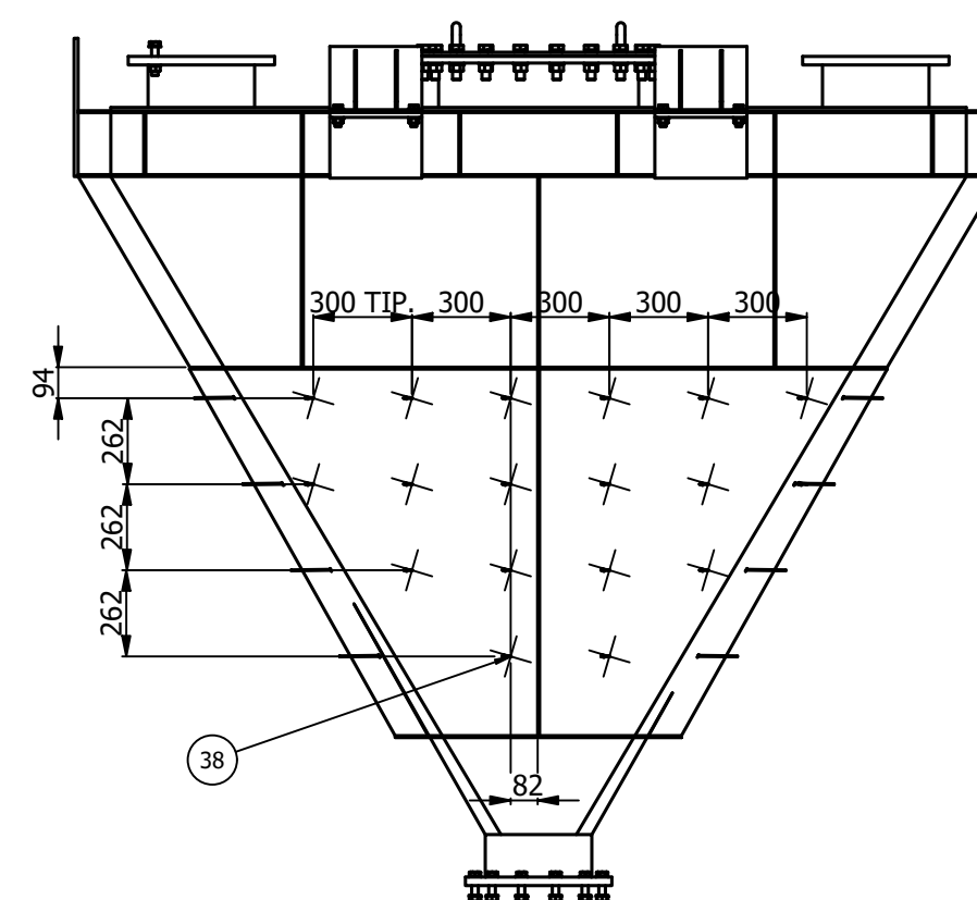
DETALLE POSICION PINES PARA AISLAMIENTO ESCALA:(1 : 25)
