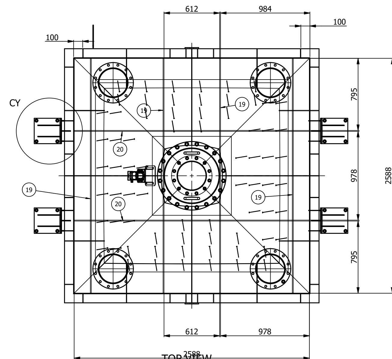
TOP VIEW ESCALA:(1 : 25)
