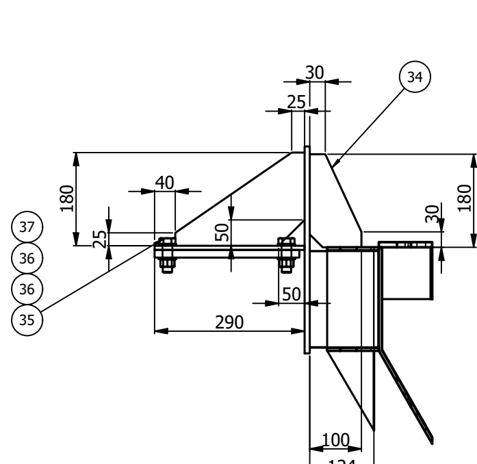
VISTA FRONTAL ESCALA:(1 : 10)
