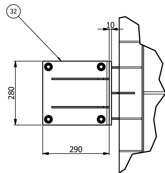
DETALLE EN PLANTA ESCALA:(1 : 10)
