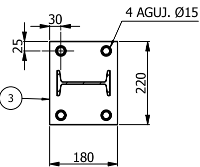
CORTE W-W
