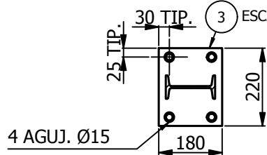
CORTE V-V
