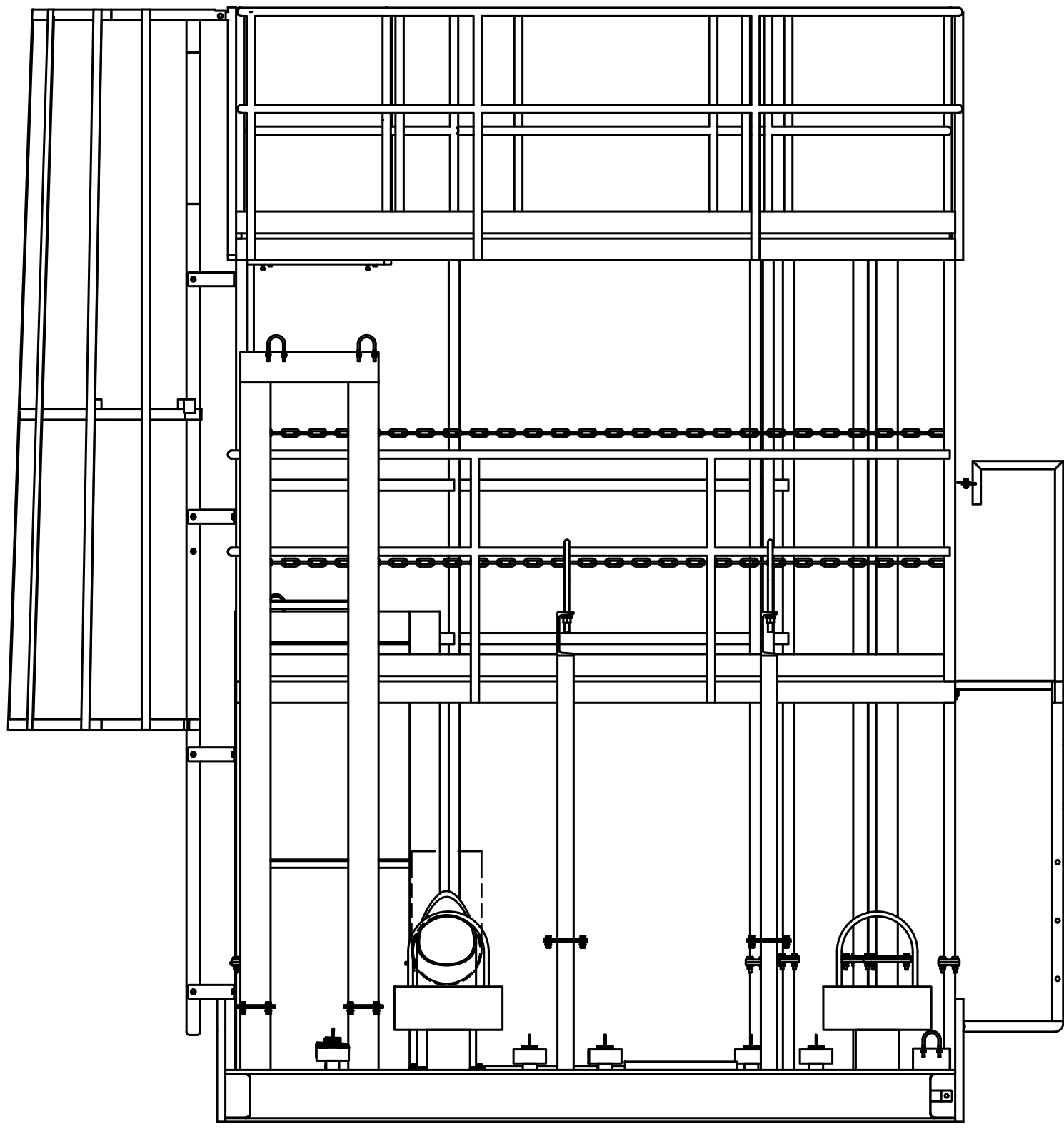
VISTA LATERAL IZQUIERDA ESCALA:(1 : 25)
