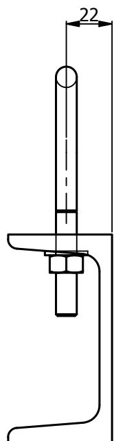
VISTA LATERAL
