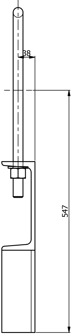
VISTA LATERAL
