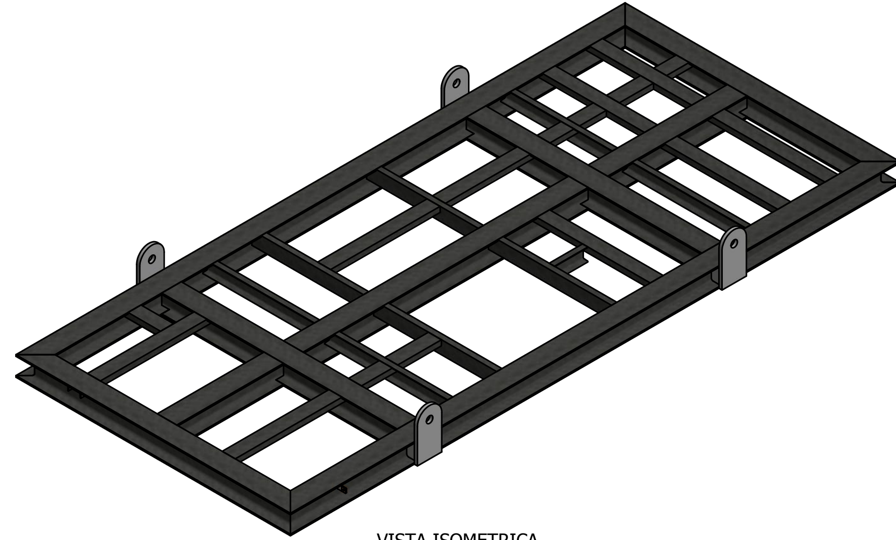
VISTA ISOMETRICA ESCALA:(0,03 : 1)
