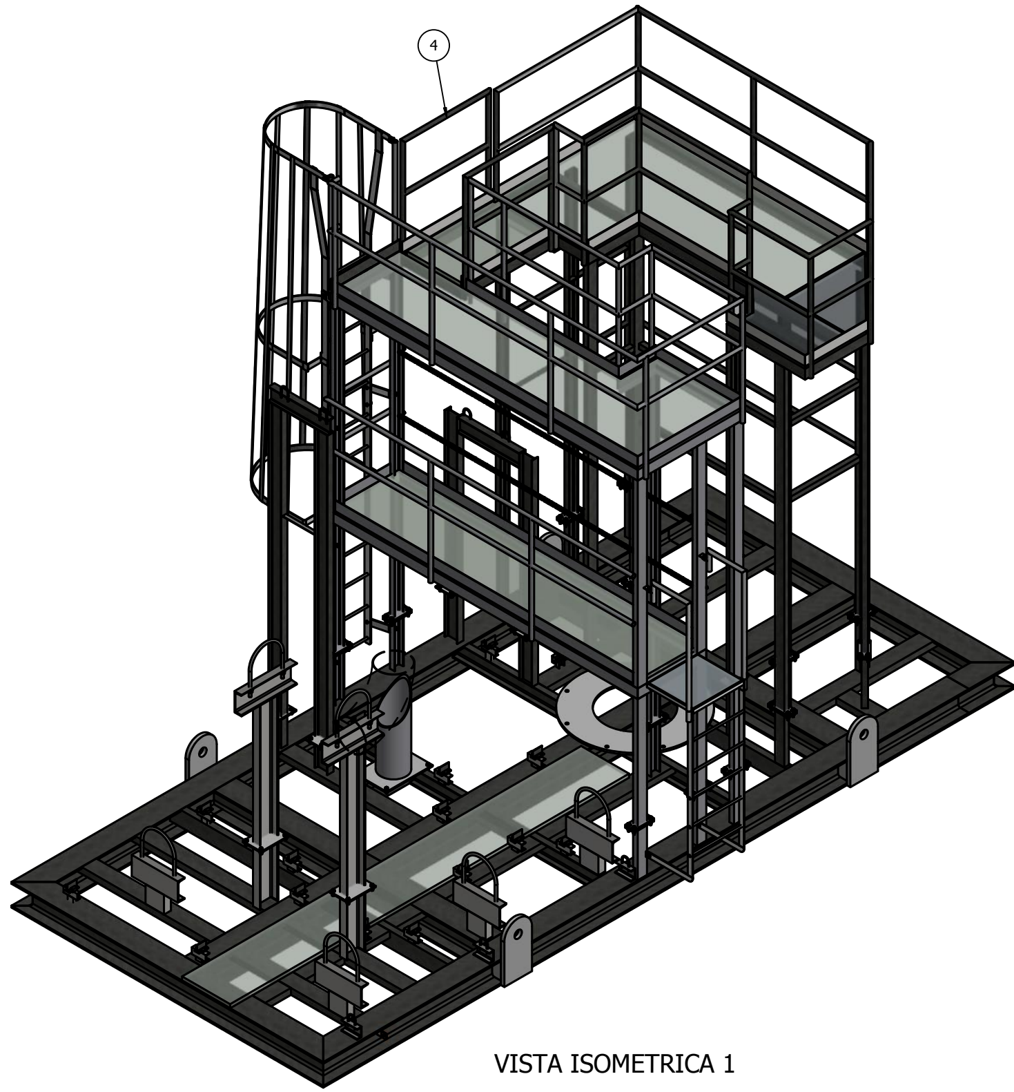
VISTA ISOMETRICA 1 ESCALA:(1 : 40)
