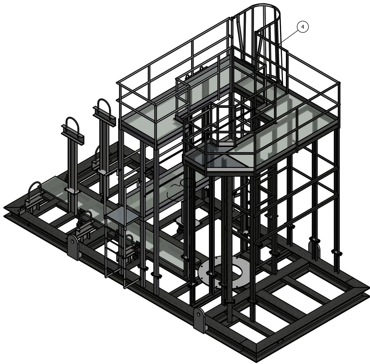
VISTA ISOMETRICA 2 ESCALA:(1 : 40)
