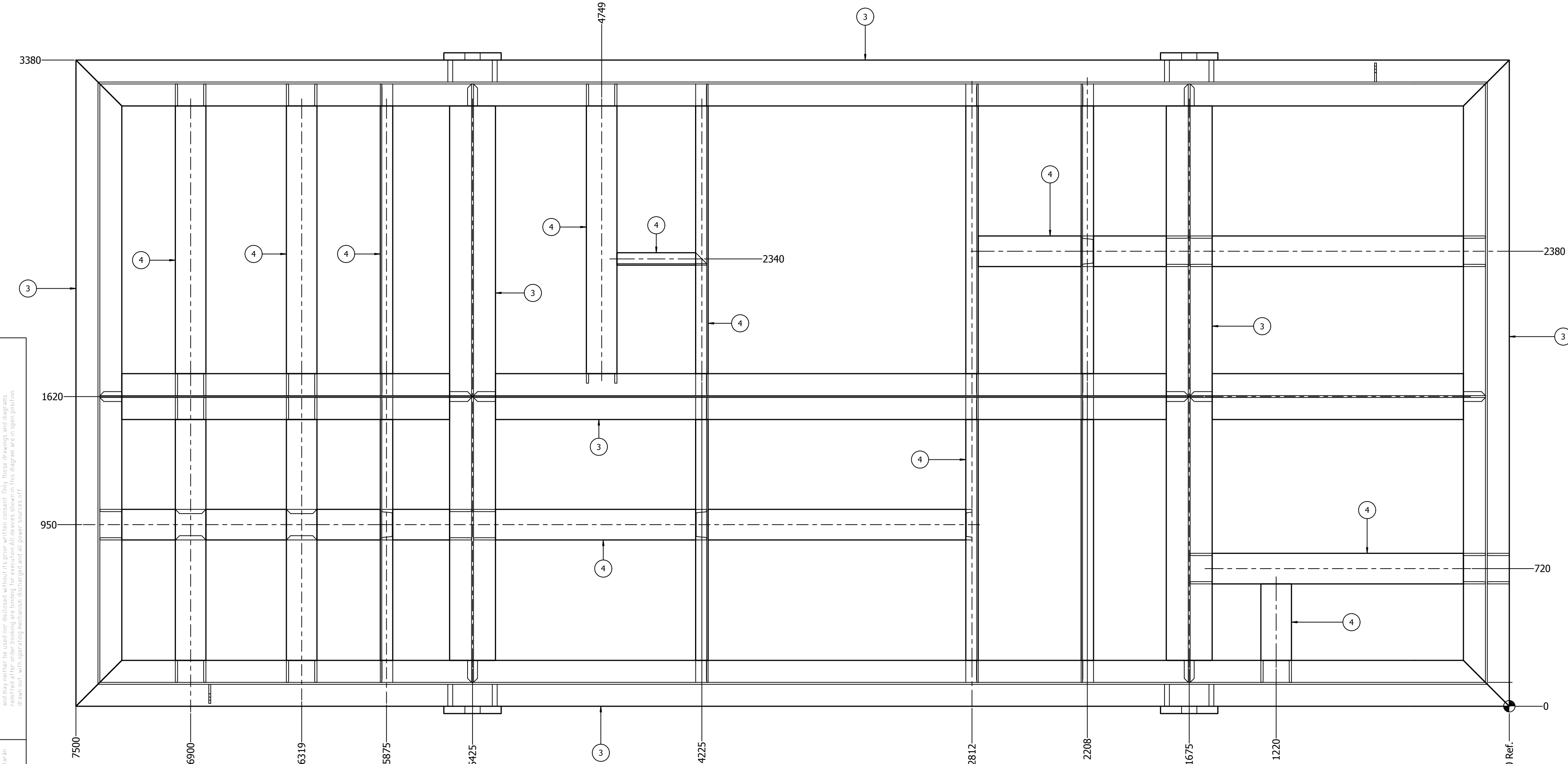
VISTA SUPERIOR ESCALA:(1:15)
