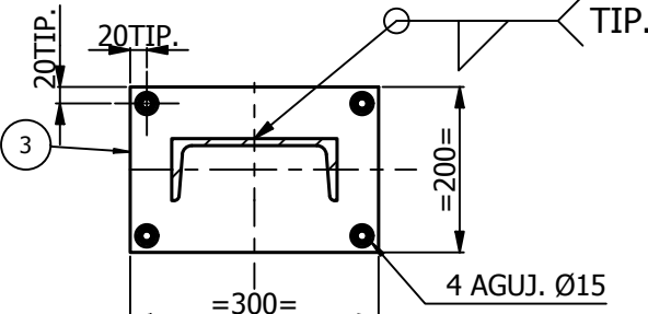
CORTE U-U
