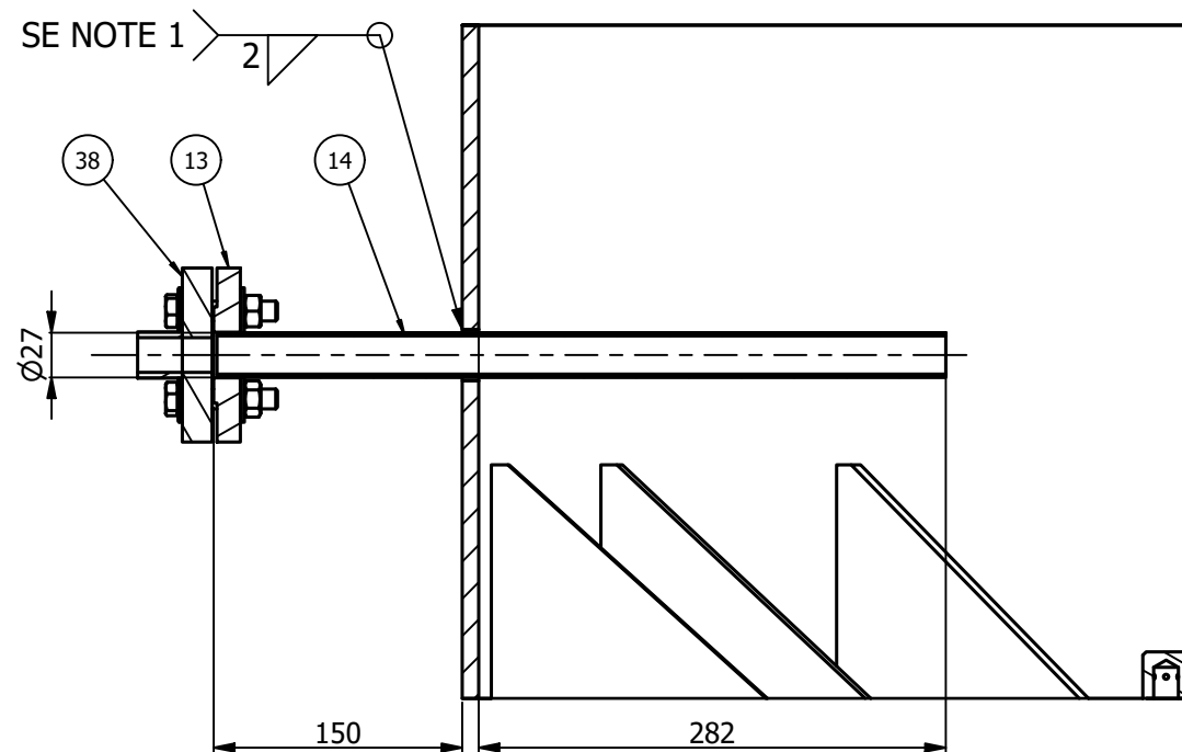
DETALLE TIPICO SENSORES DE PRESION
