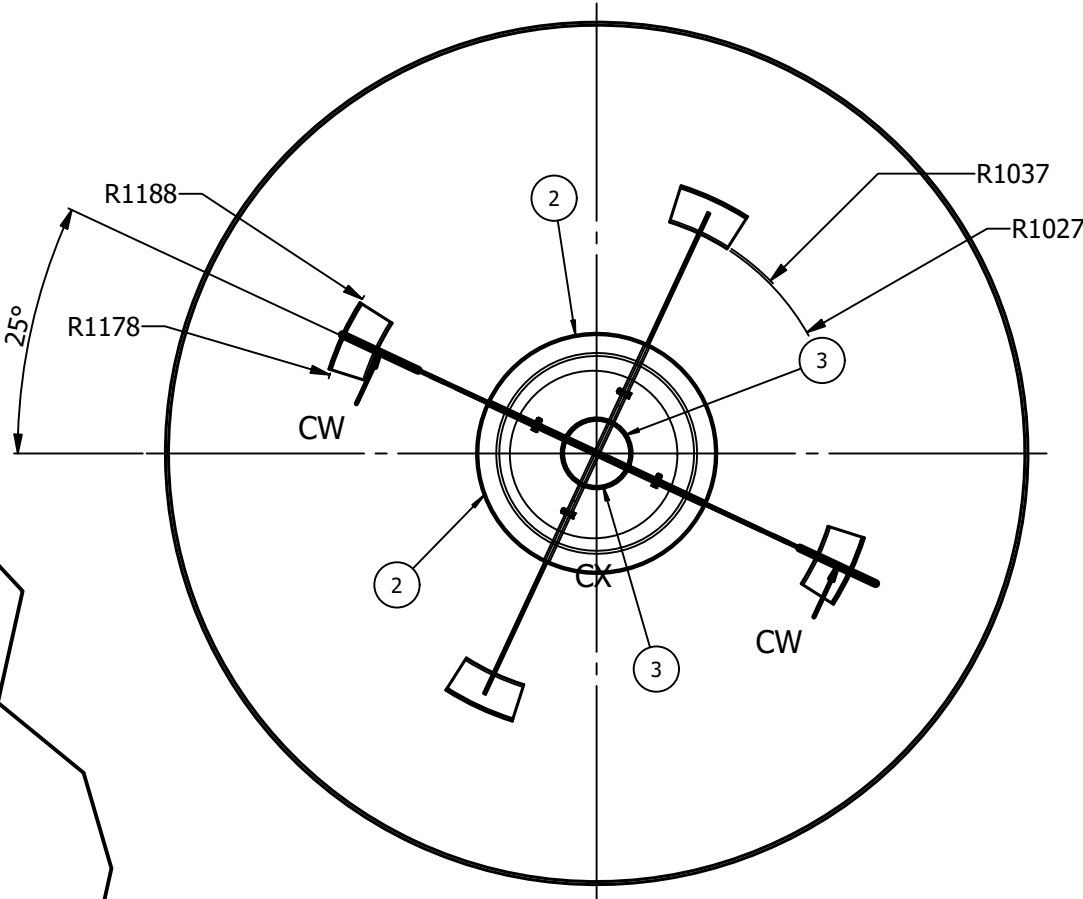
BOTTOM VIEW ESCALA:(1 : 32)
