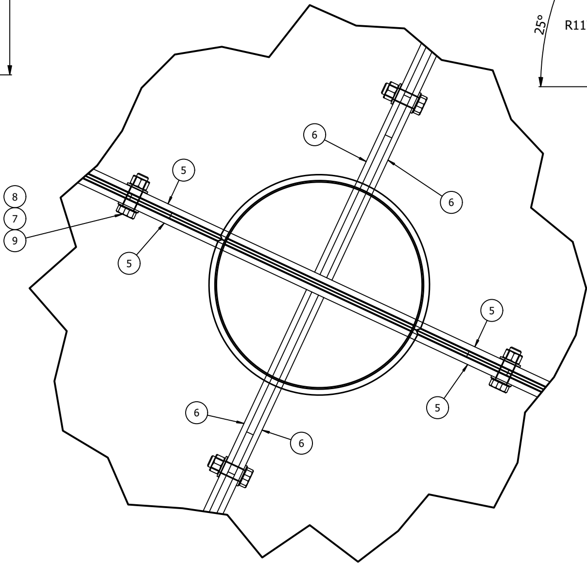
DETALLE CX ESCALA:(1 : 5)
