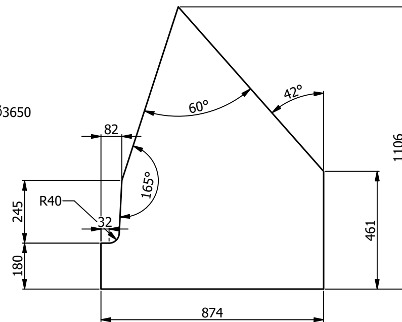
DETAIL POS. 20
