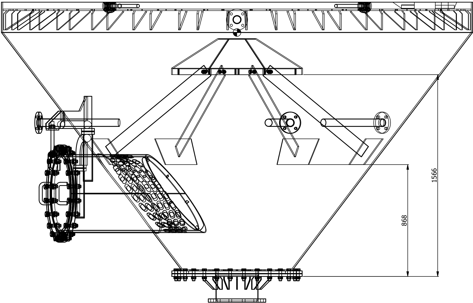
FRONT VIEW ESCALA:(1 : 15)
