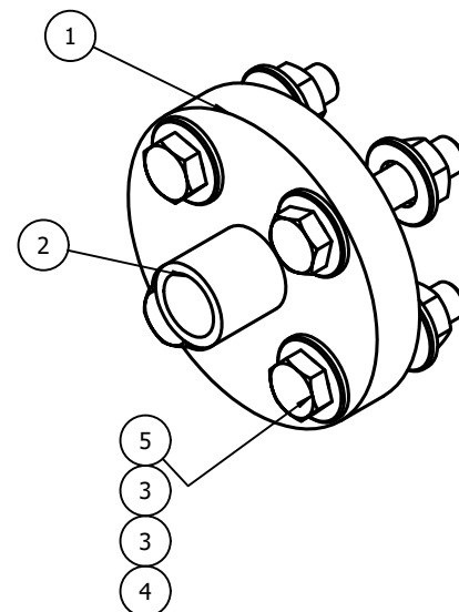
VISTA ISOMETRICA
