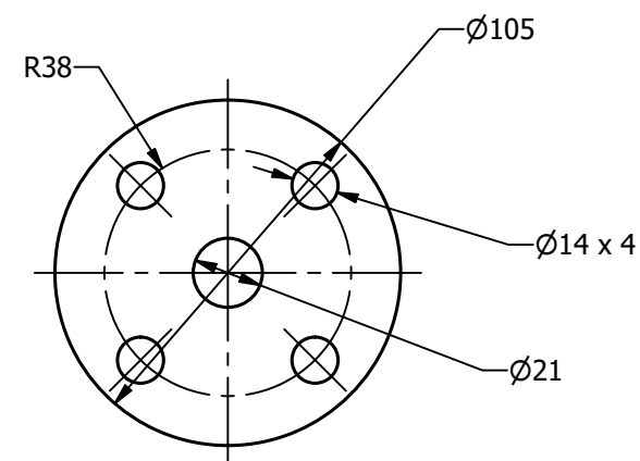
FRONTAL BRIDA MECANIZADA
