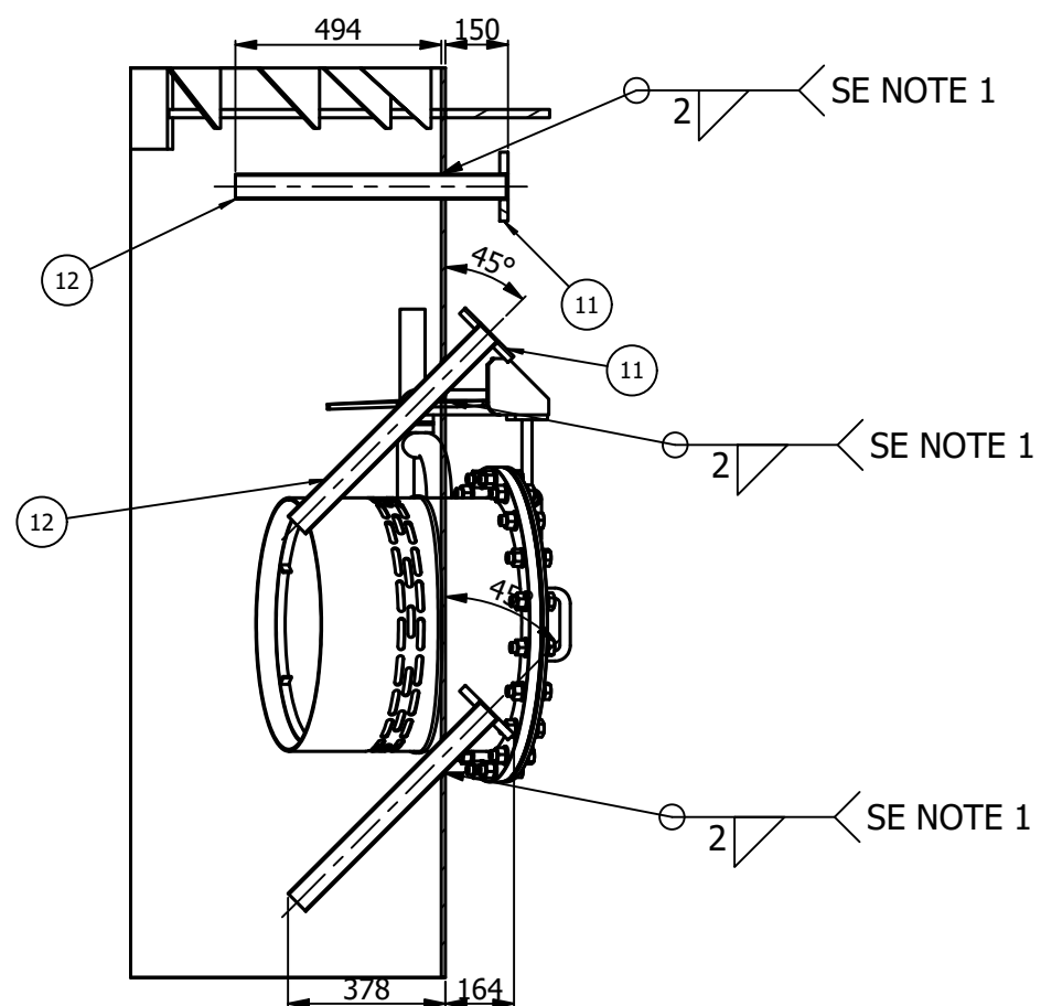
DETALLE TIPICO SENSORES DE TEMPERATURA
