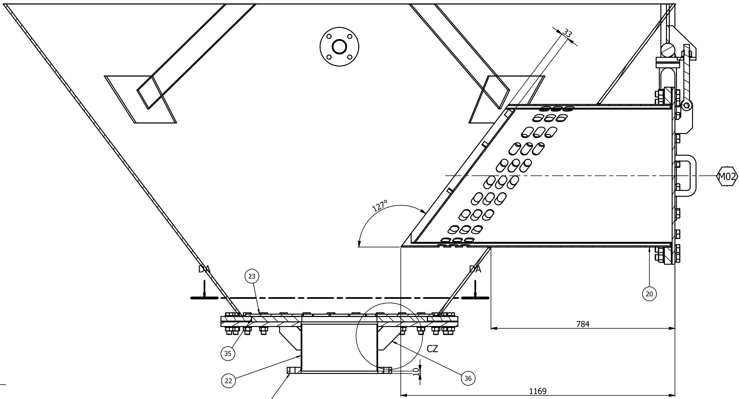
VISTA EN CORTE MANHOLE M02 ESCALA:(1 : 10)
