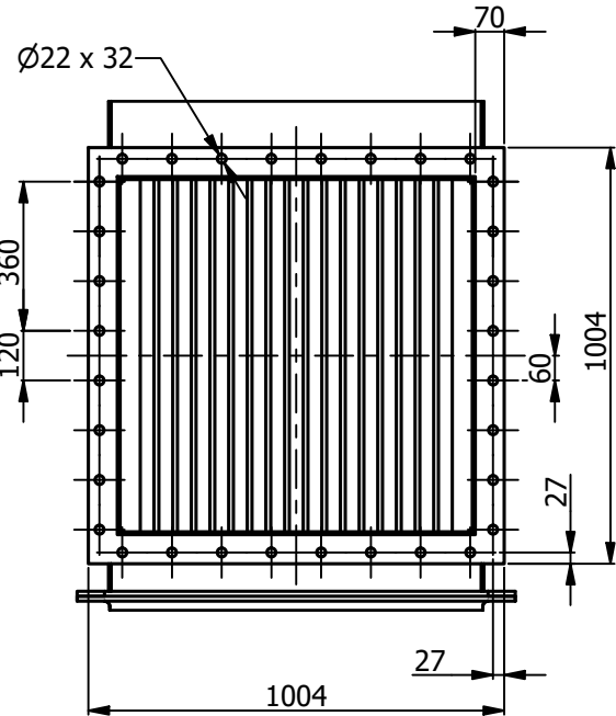
DETAIL CG ESCALA:(1 : 20)
