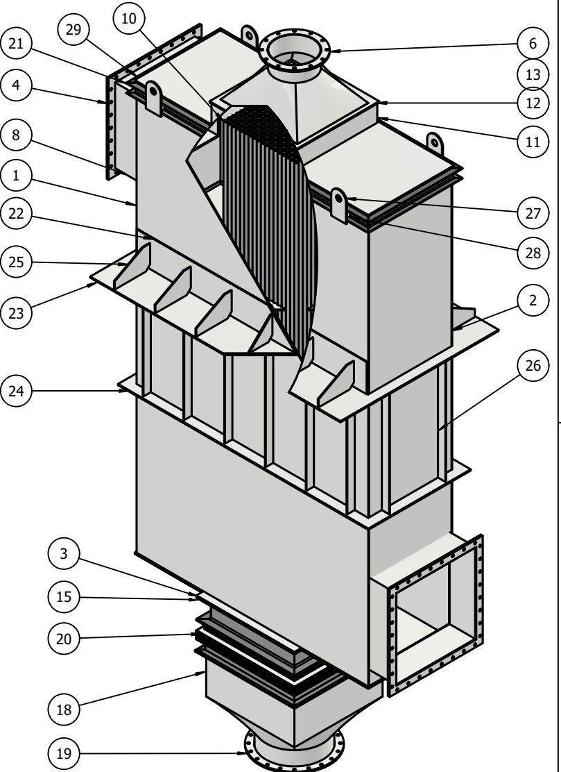
ISOMETRIC VIEW ESCALA:(1 : 40)
