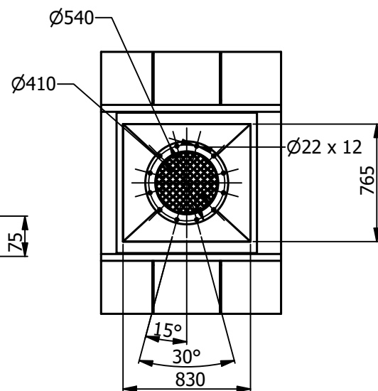
DETAIL CF ESCALA:(1 : 35)
