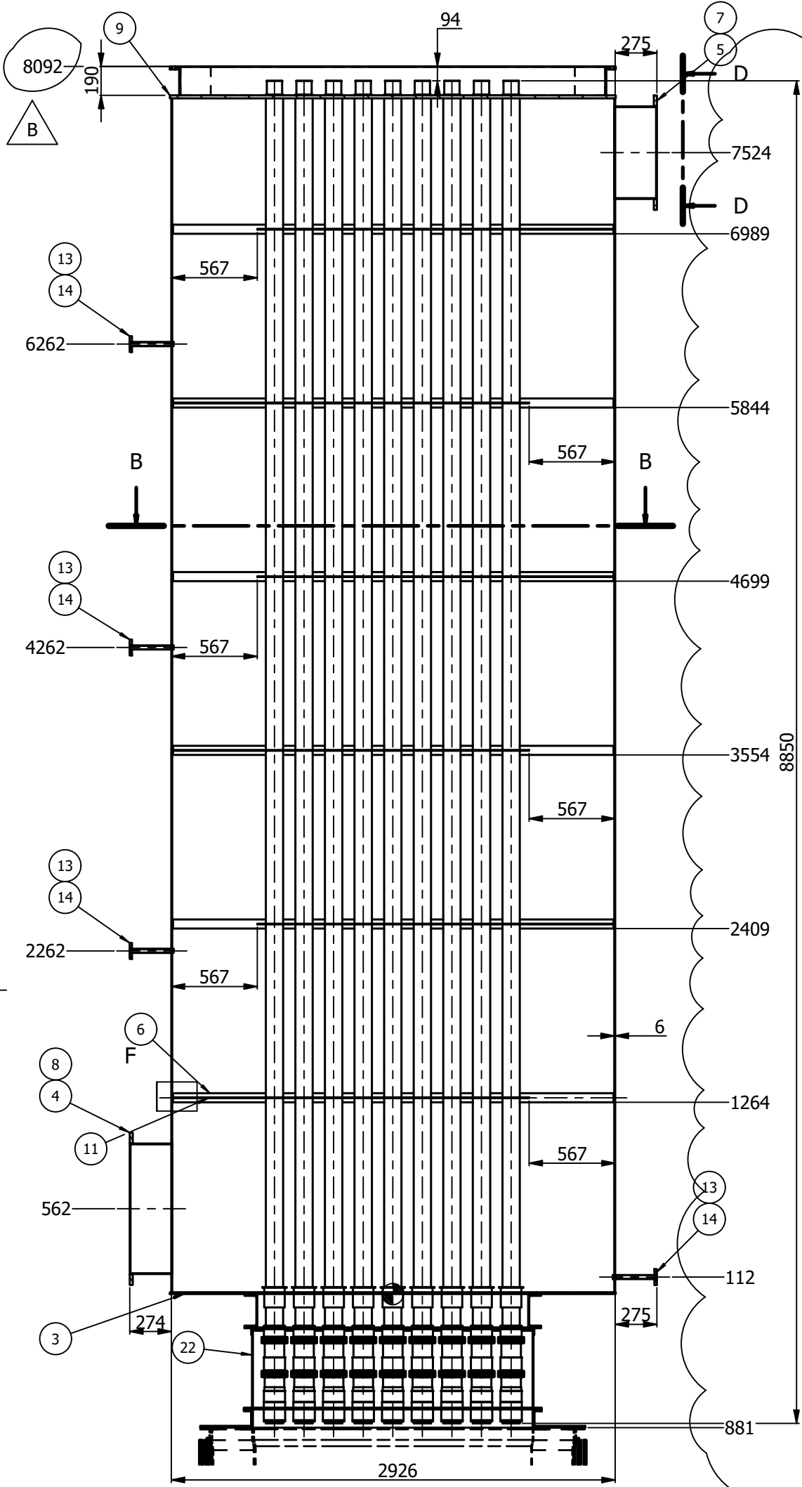
CUT A-A
