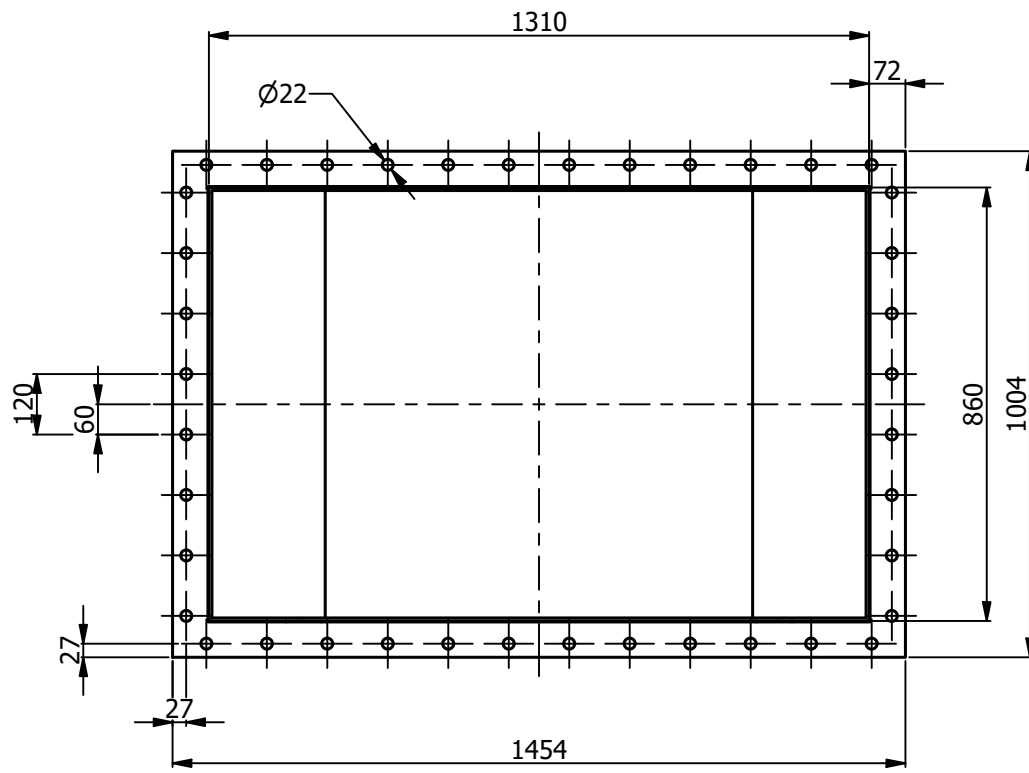
CUT B-B ESCALA:(1 : 15)
