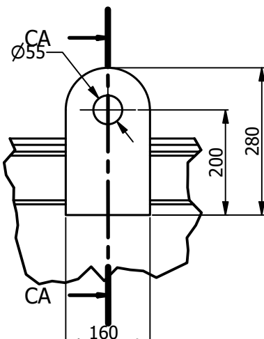
DETAIL BZ ESCALA:(1 : 10)
