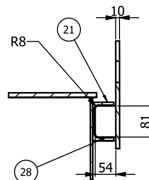
CUT CA-CA ESCALA:(1 : 10)
