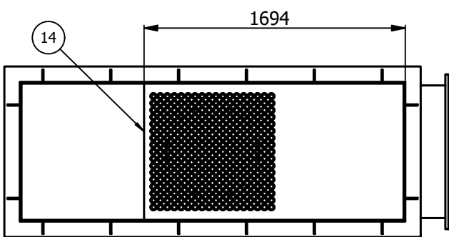
CUT B-B ESCALA:(1 : 35)
