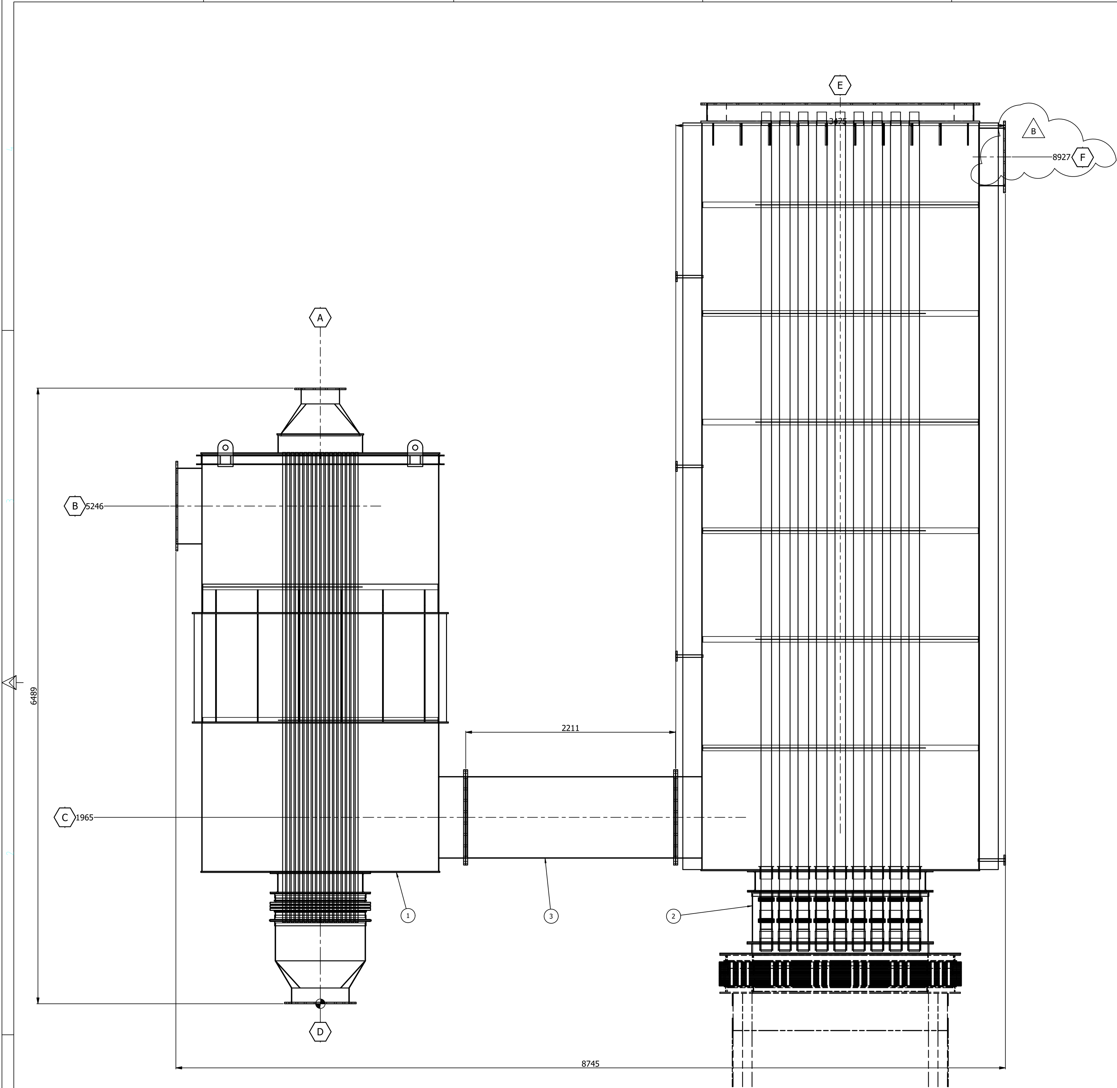
SIDE VIEW ESCALA:(1 : 25)
