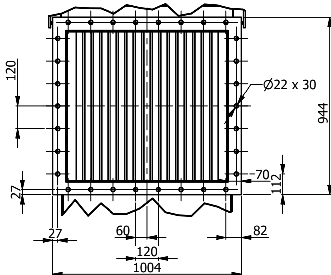
DETAIL D ESCALA:(1 : 20)
