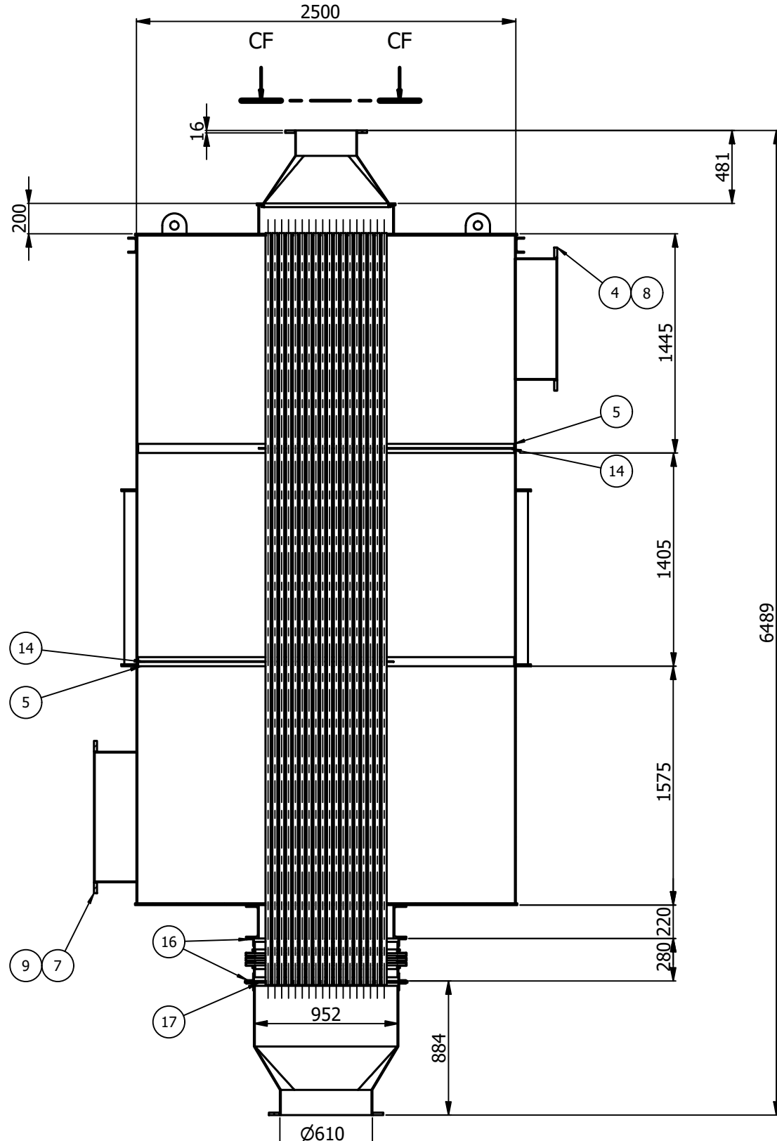
CUT B-B ESCALA:(1 : 35)
