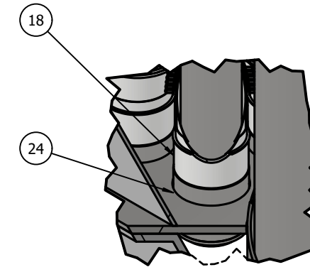
DETAIL CI
