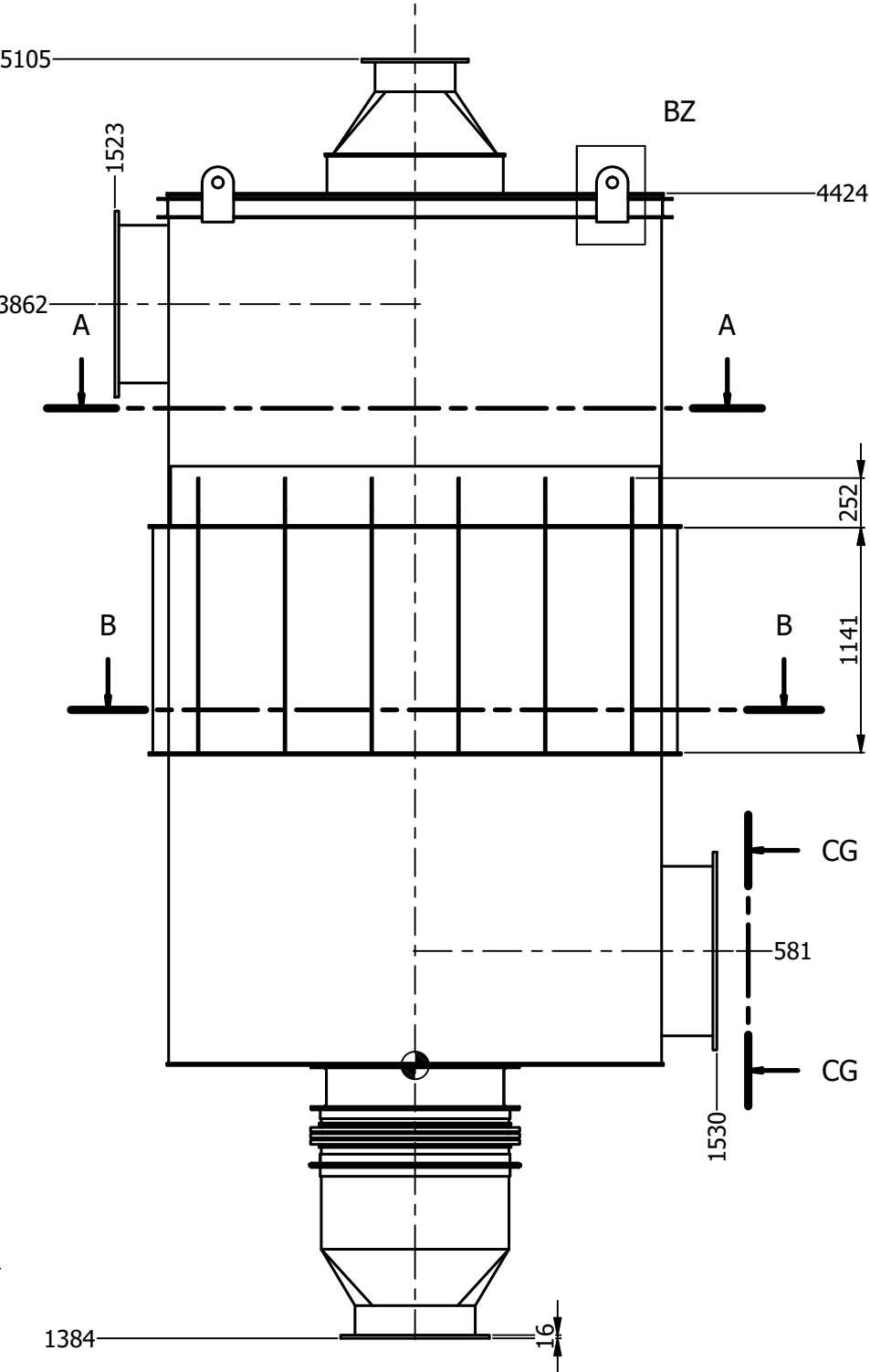
FRONT VIEW ESCALA:(1 : 35)
