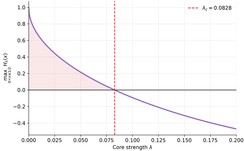
Figura 3: Verificación numérica del criterio de monotonía. El cruce por cero de \max_{0 < x \leq 1/2} [A_\lambda + 2xA'_\lambda] determina \lambda_c \simeq 0.0828 ; para valores mayores, la fuerza aumenta monótonamente al aproximarse las células.
