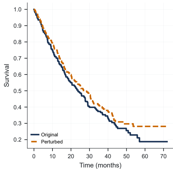
CSF1R
