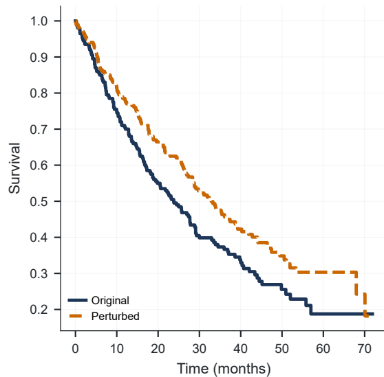
CTLA4-BLOCKADE
