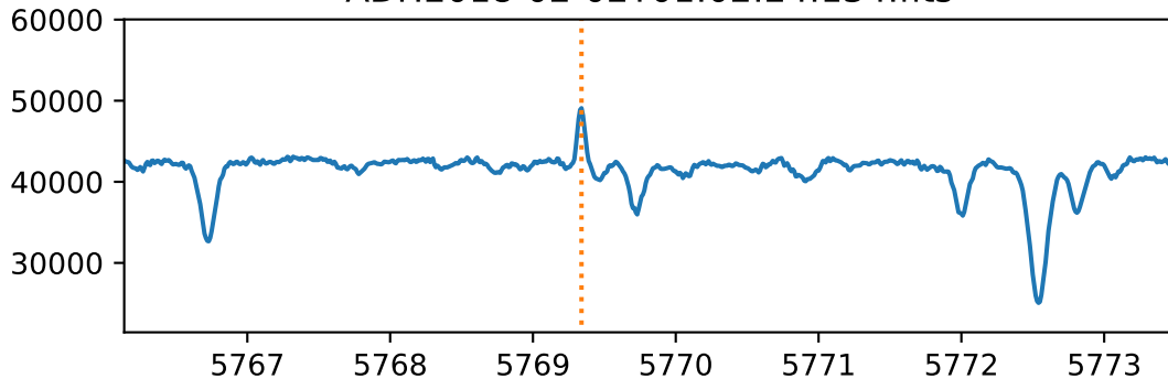
ADP.2018-02-02T01:02:24.134.fits
