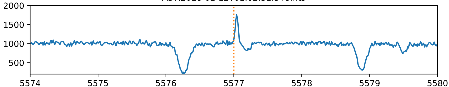
HARPS.2018-02-11T01_10_40.579.fits
