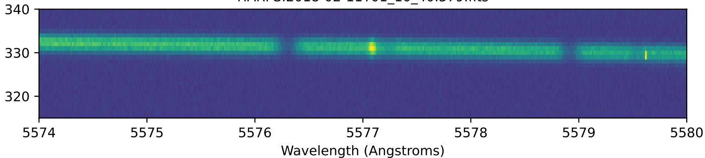
HARPS.2018-02-11T01_10_40.579.fits
