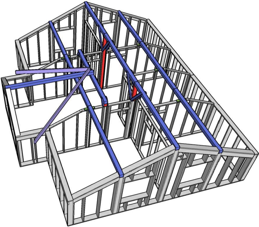
Расположение элементов каркаса.
