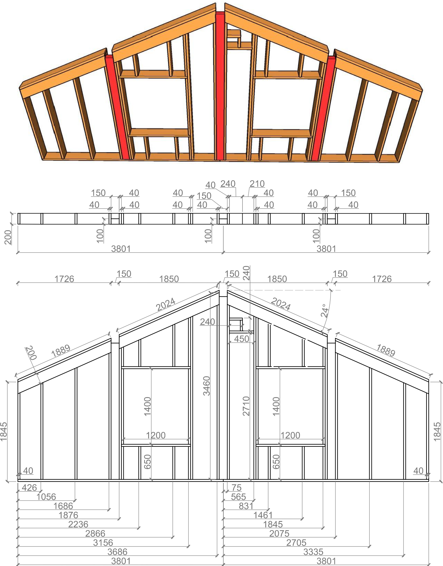
Стена по оси 4 (2-й этаж).
