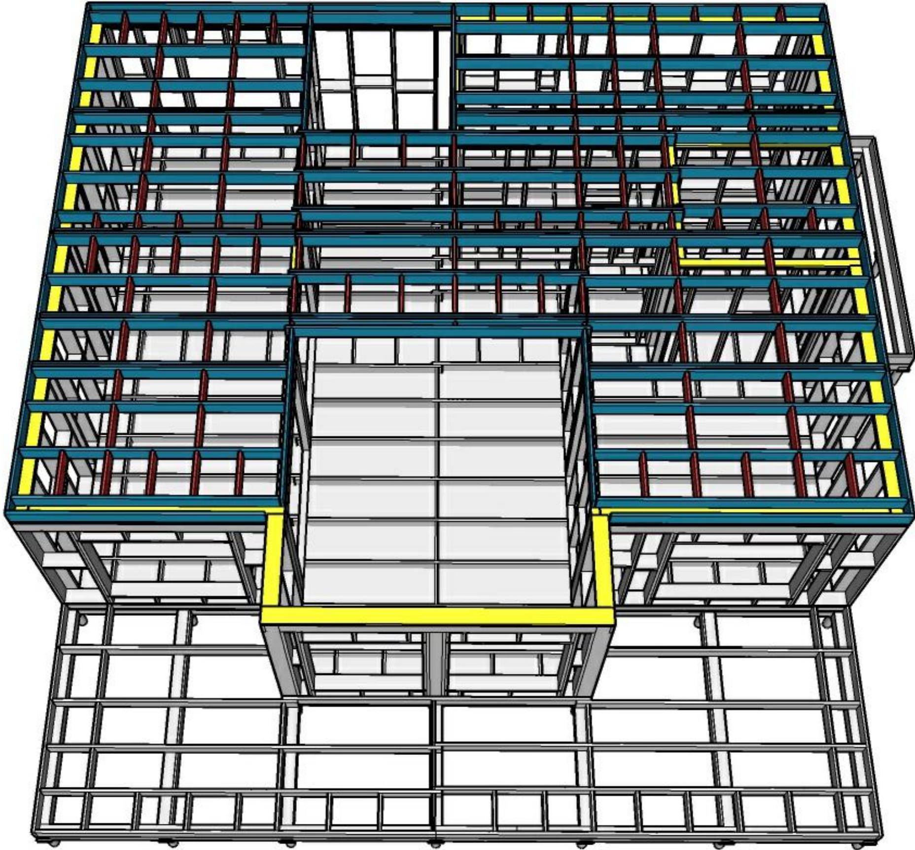
Платформа 2-го мансардного этажа. Общий вид.
