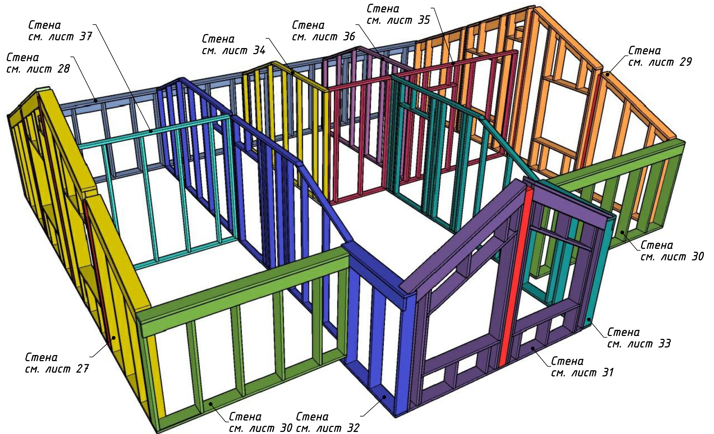
Стены 2-го мансардного этажа. Общий вид.
