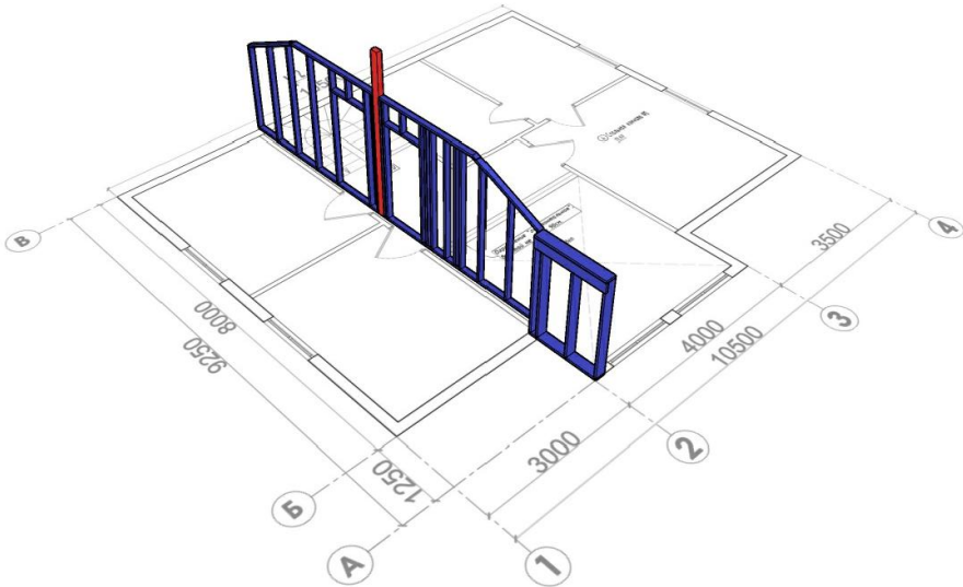
Расположение элементов каркаса.
