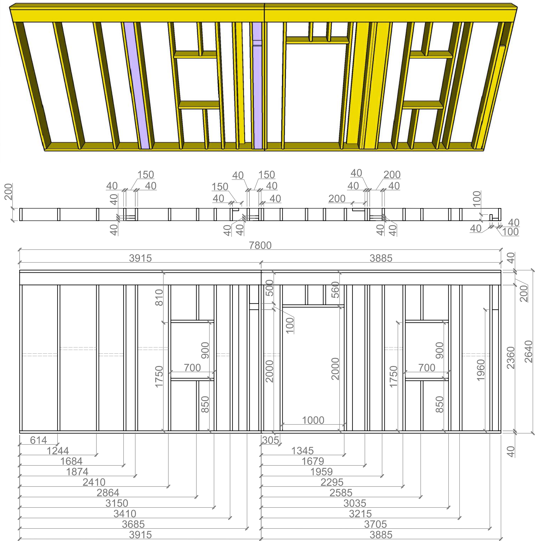
Стена по оси 4 (1-й этаж).
