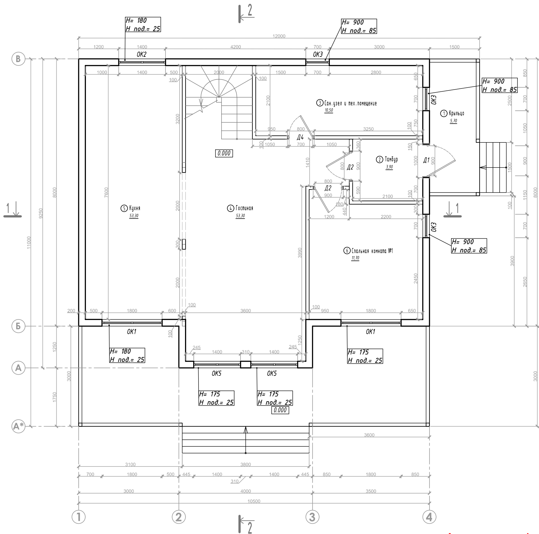
План 1-го этажа на отм. +0,000. Планировочное решение.
