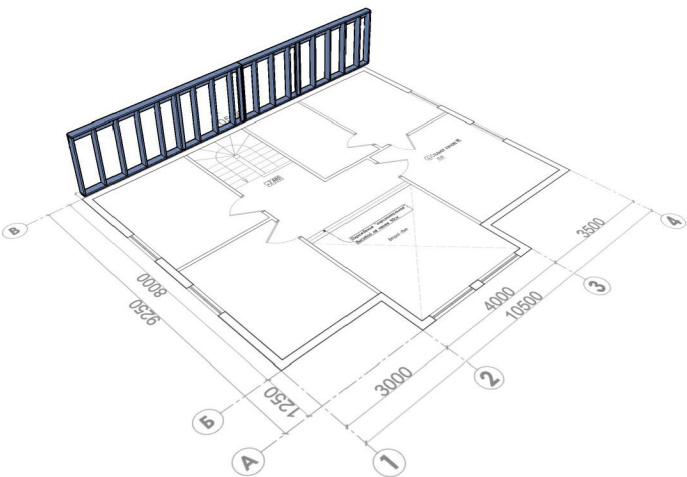
Расположение элементов каркаса.
