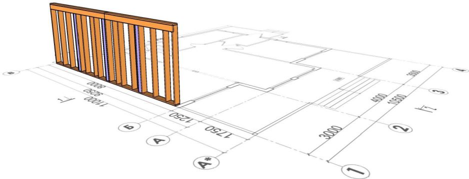
Расположение элементов каркаса.
