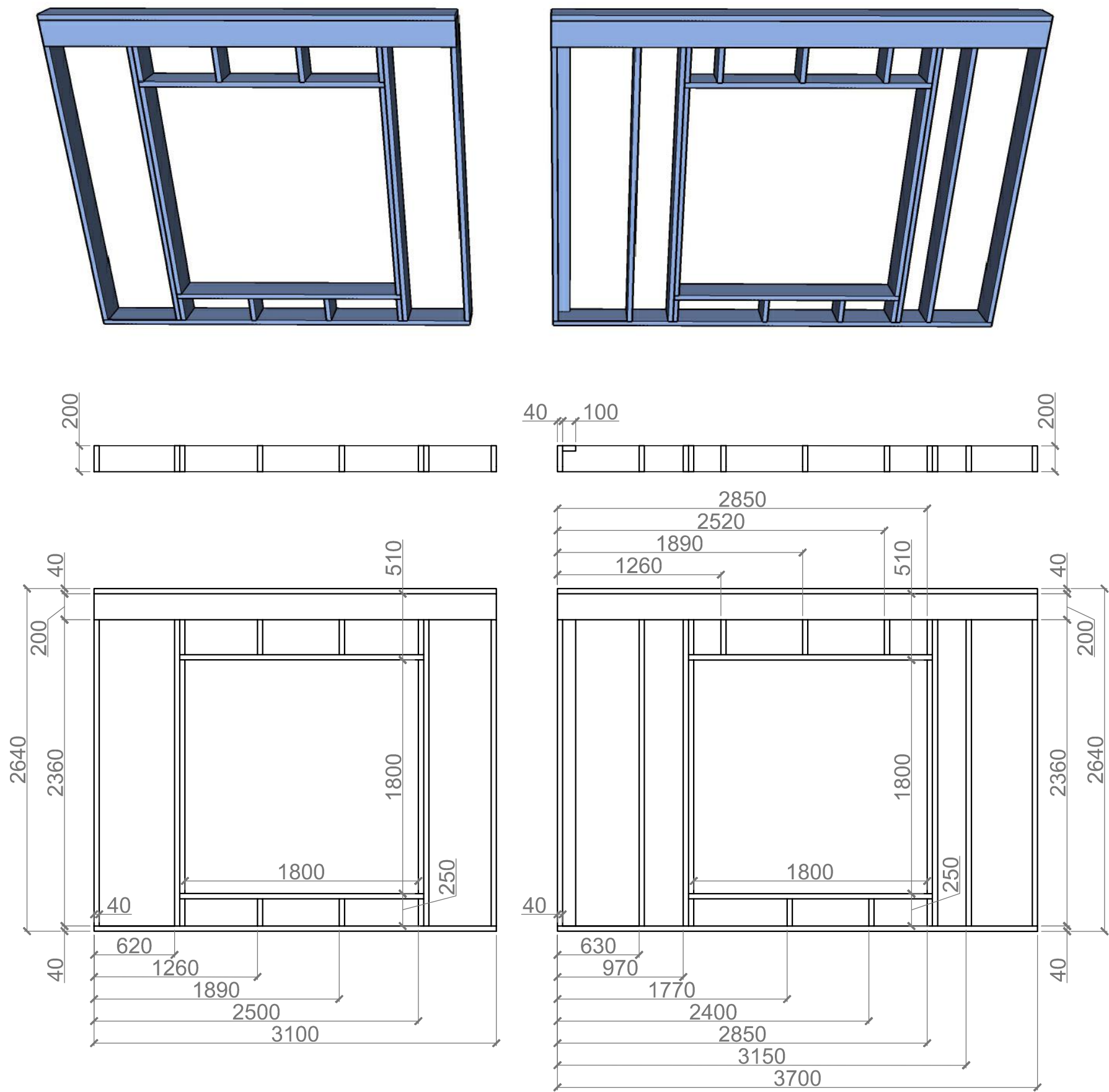
Стена по оси Б (1-й этаж).
