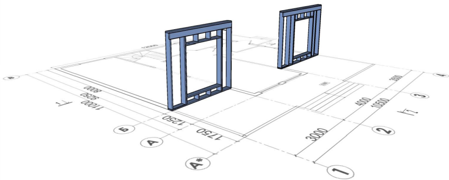
Расположение элементов каркаса.
