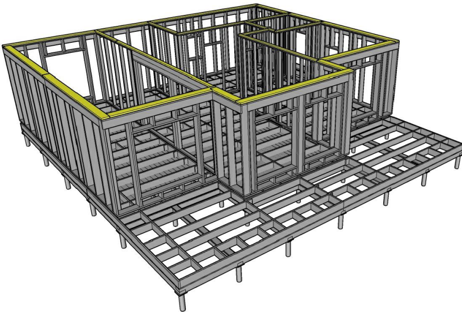
Расположение элементов каркаса.
