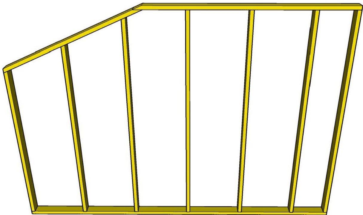
Перегородка 1 (2-й этаж).
