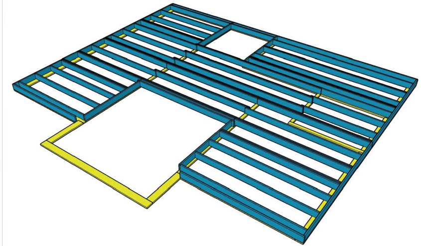
Расположение элементов каркаса.
