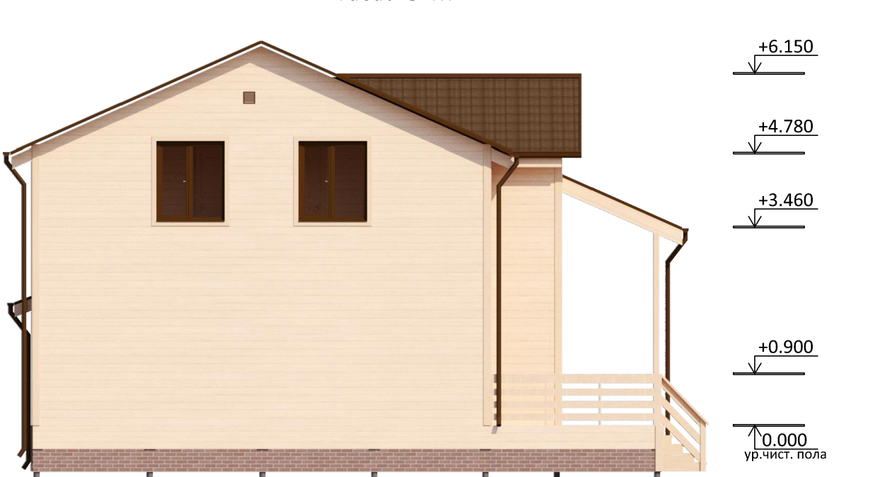
Фасад В-А.
