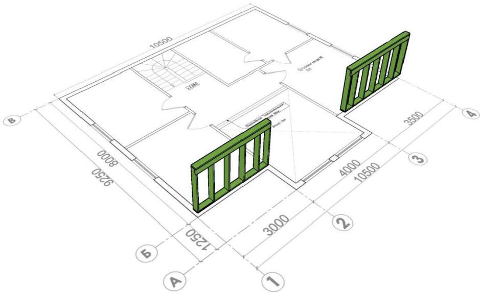
Расположение элементов каркаса.
