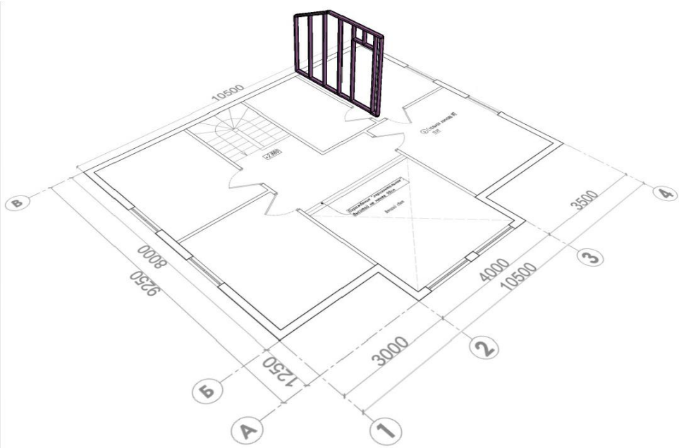
Расположение элементов каркаса.
