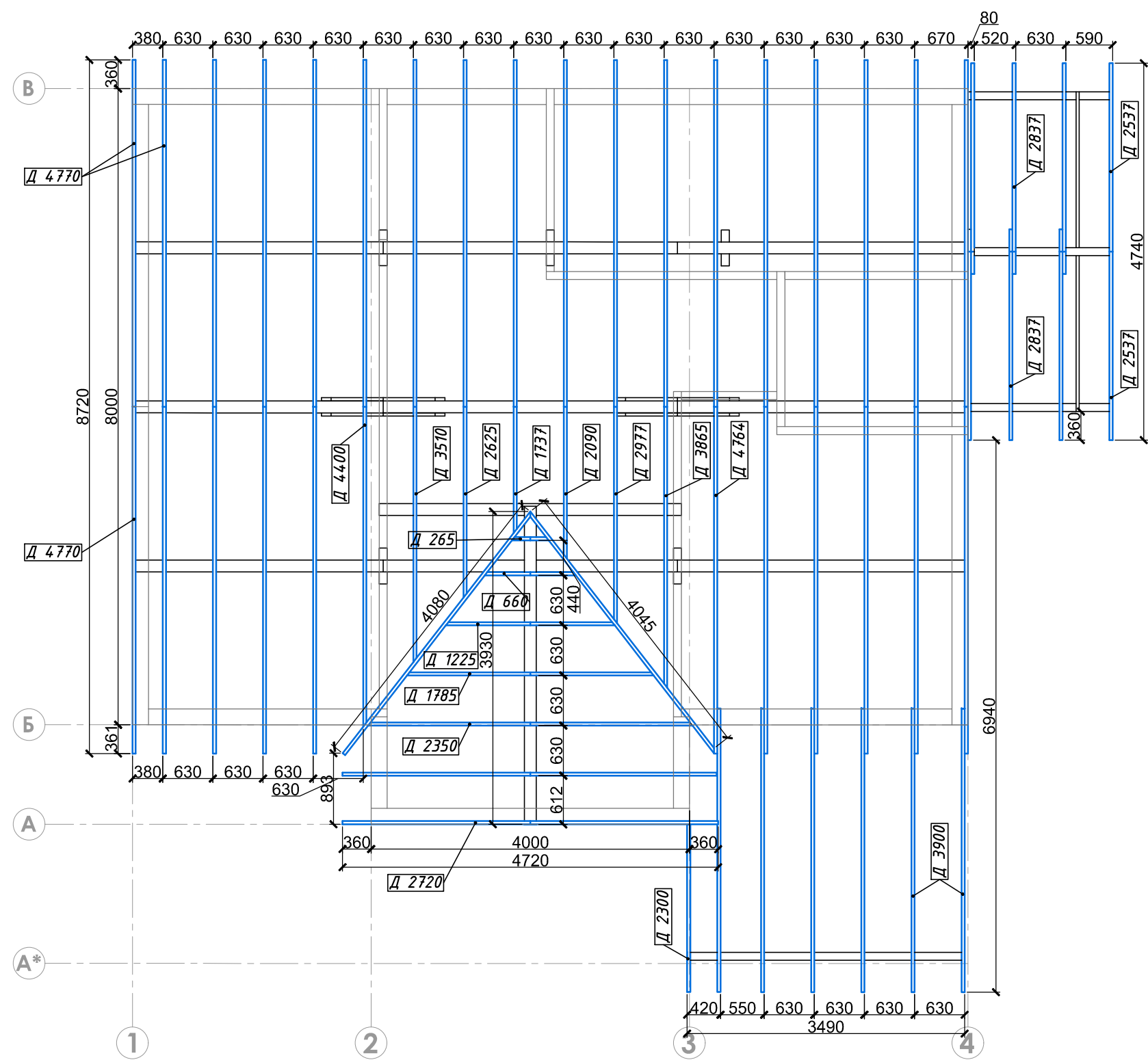
Стропильная система. Схема раскладки.
