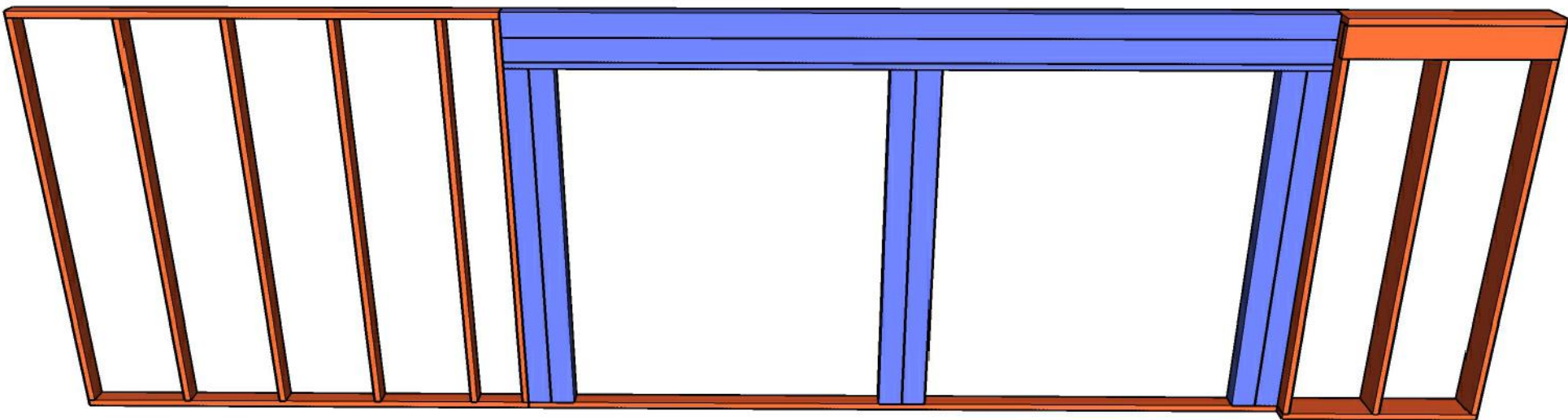
Стена по оси 2 (1-й этаж).
