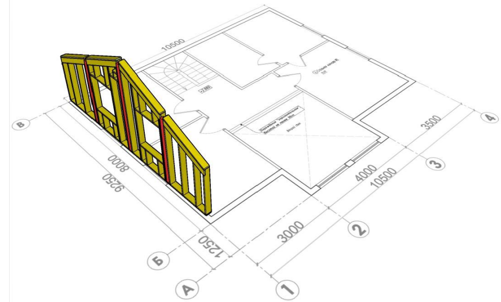
Расположение элементов каркаса.
