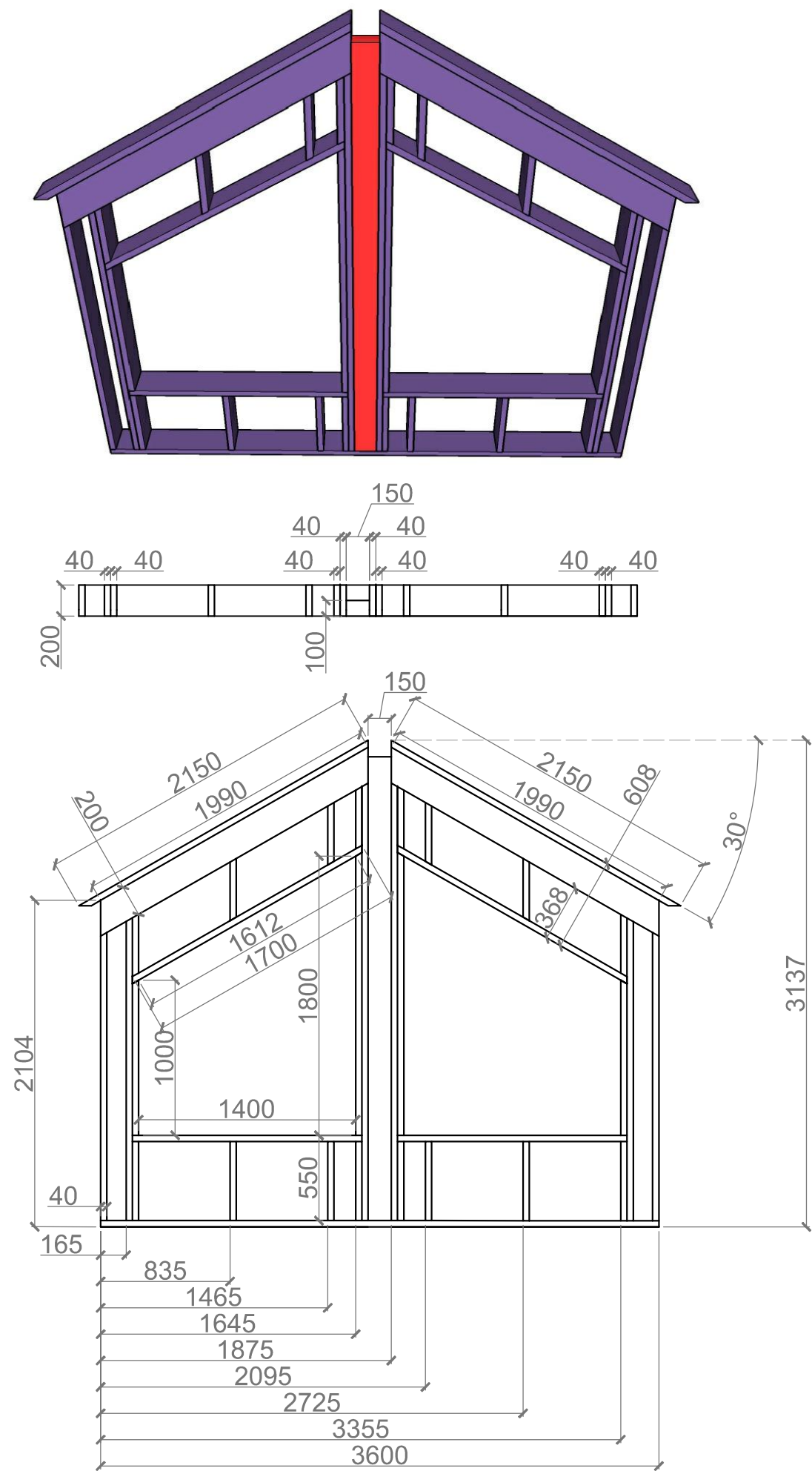
Стена по оси А (2-й этаж).
