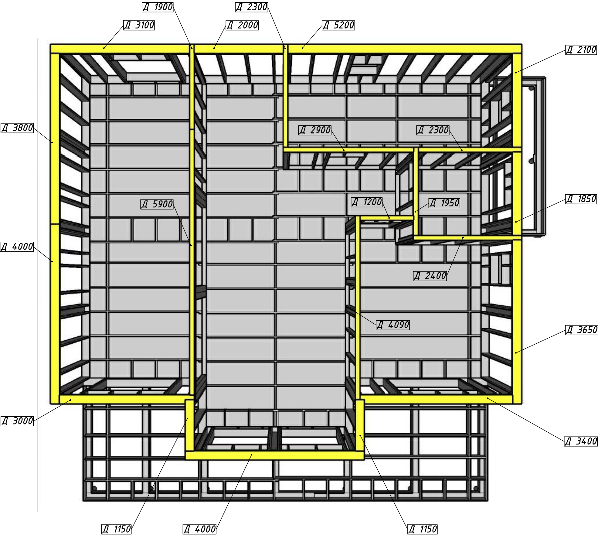
Схема обвязки стен 1-го этажа.
