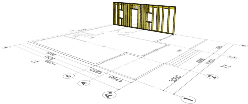
Расположение элементов каркаса.
