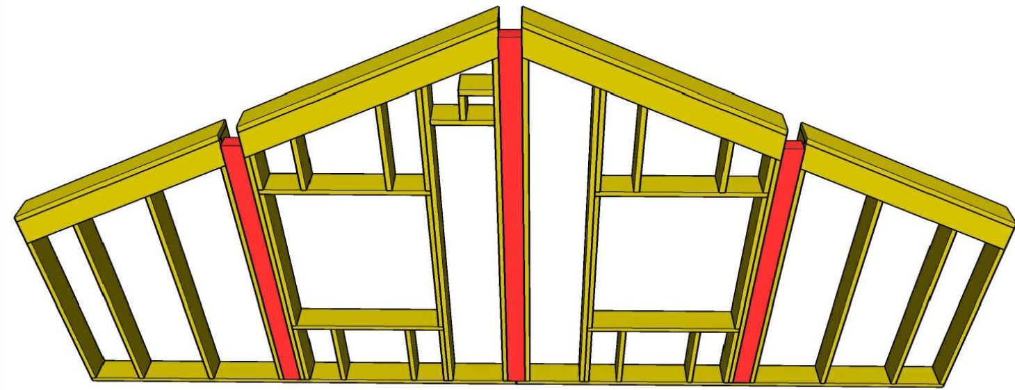
Стена по оси 1 (2-й этаж).
