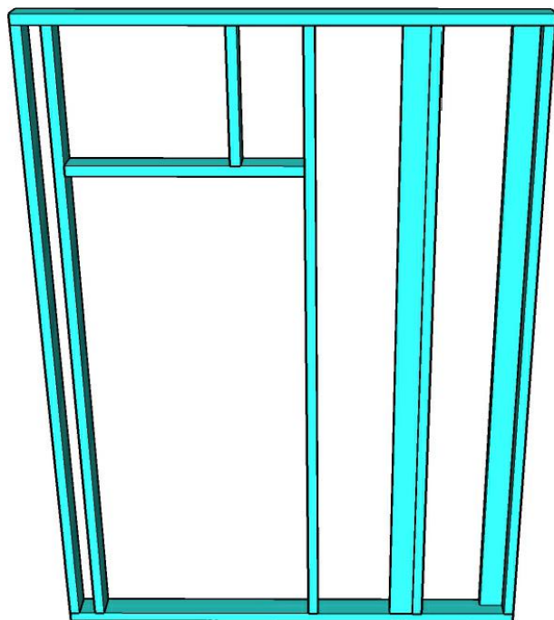
Перегородка 4 (1-й этаж).
