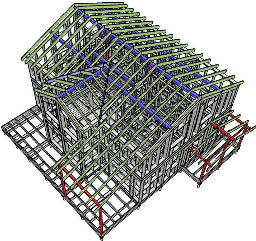
Стропильная система. Общий вид.
