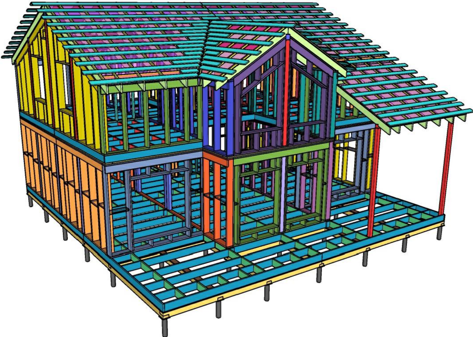
Крыша. Общий вид.
