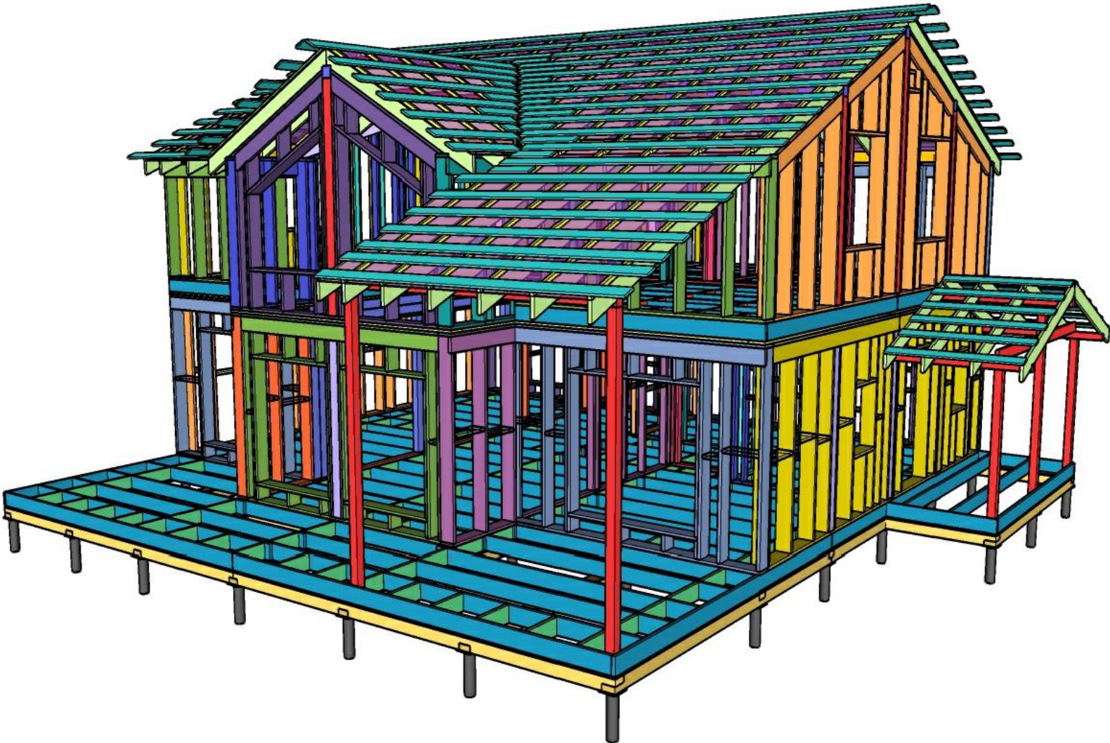
Крыша. Общий вид.
