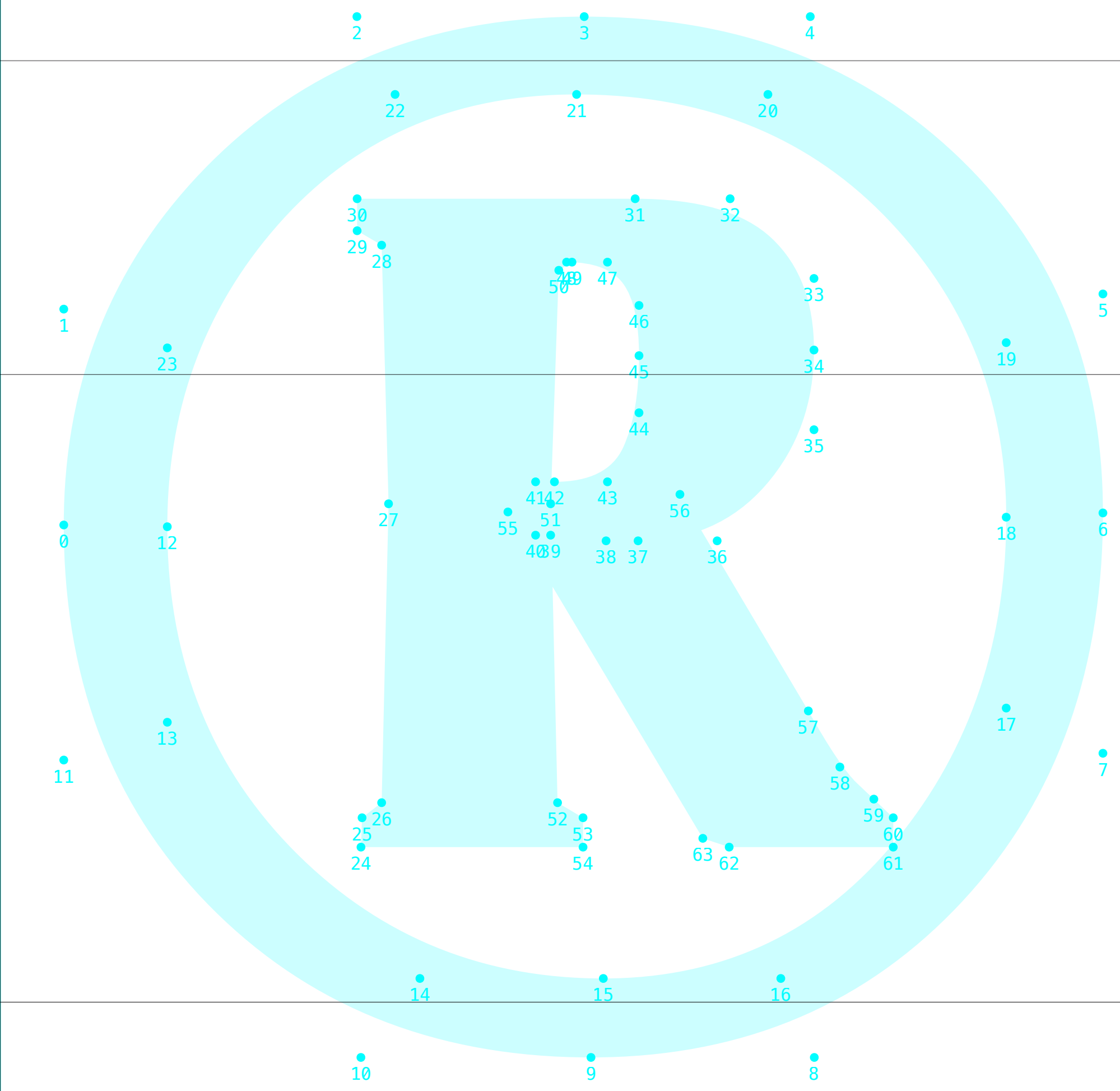
parametric
