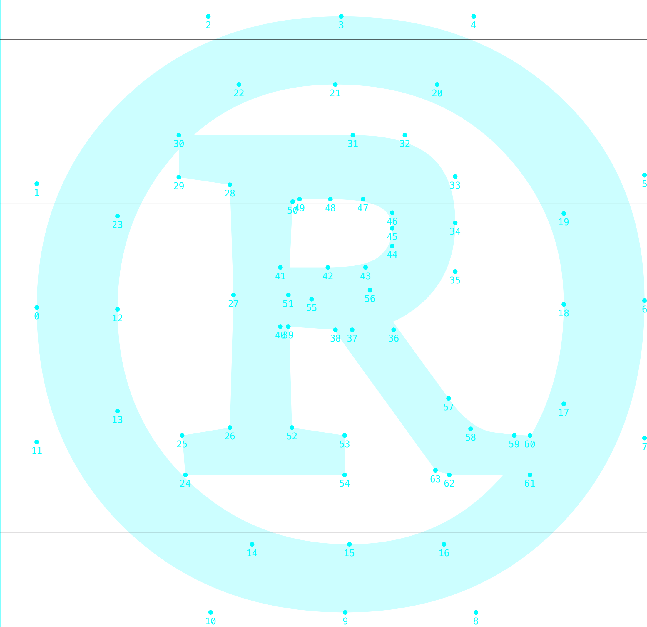
parametric
