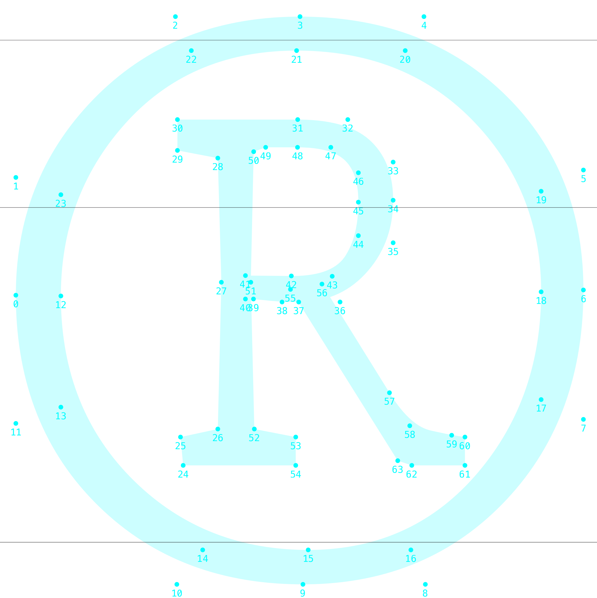
parametric
