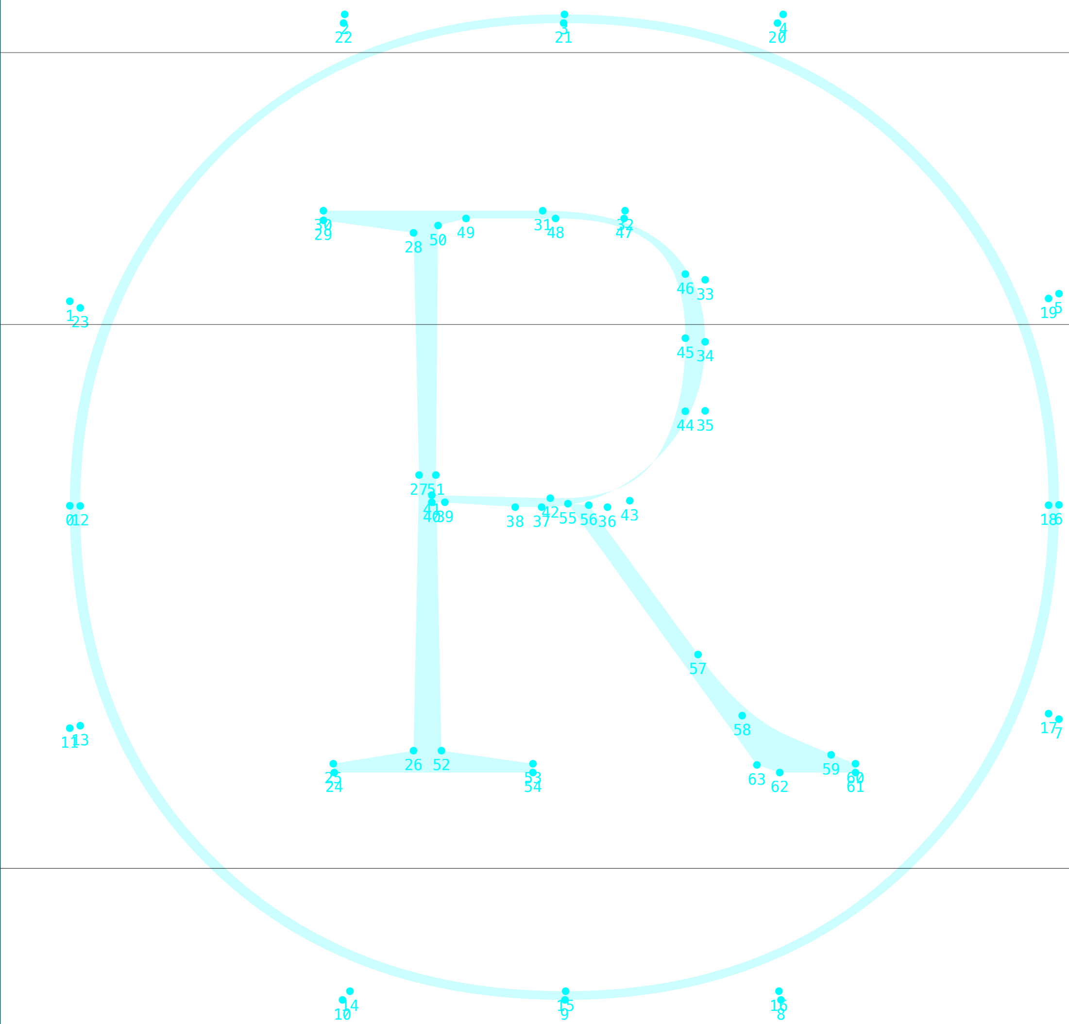
parametric
