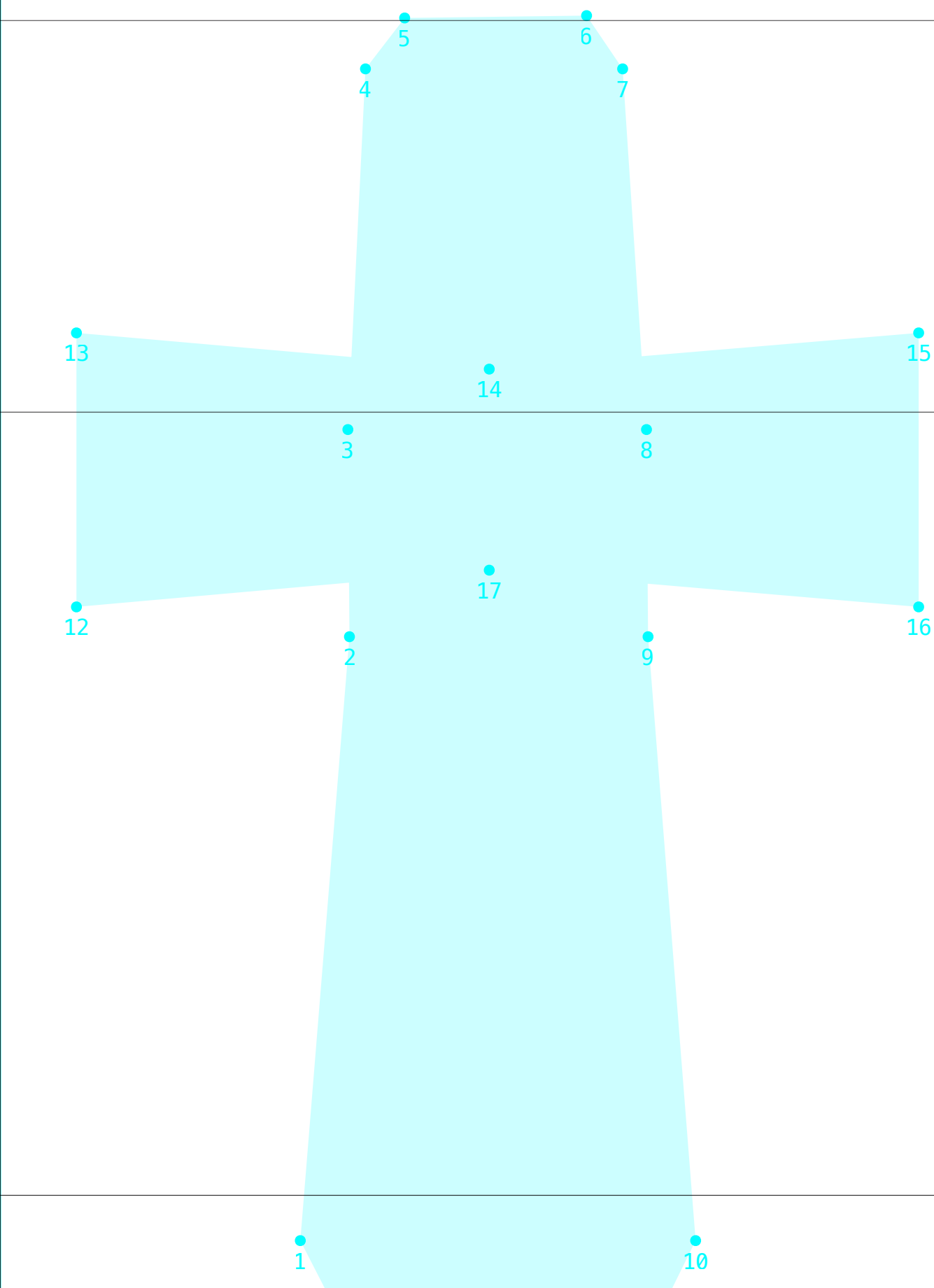
parametric
