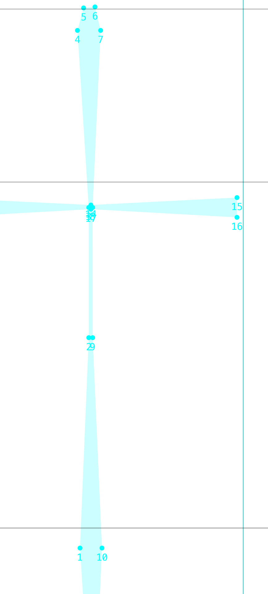
parametric
