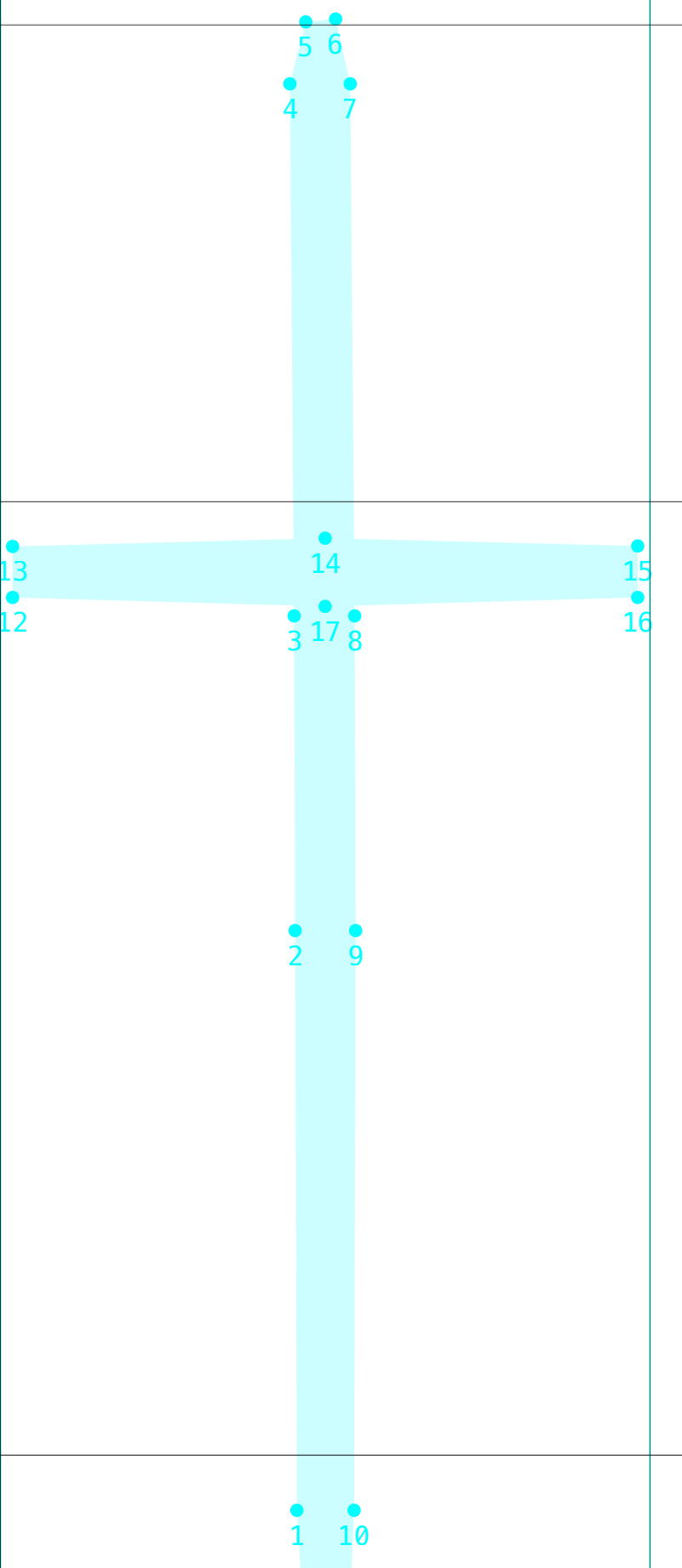
parametric
