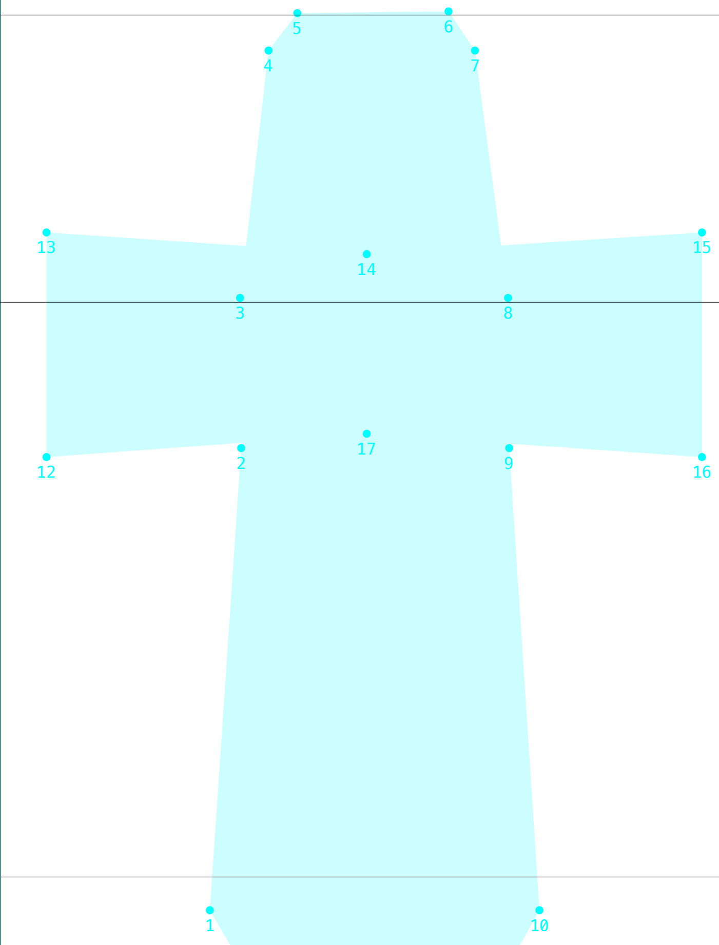
parametric
