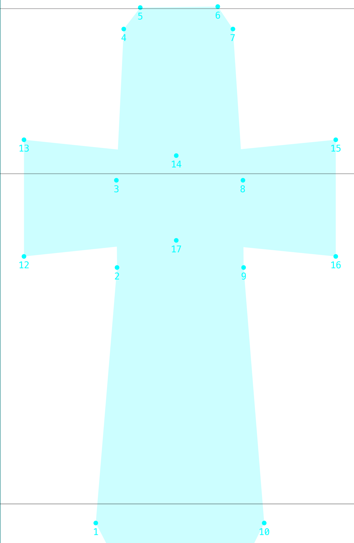
parametric
