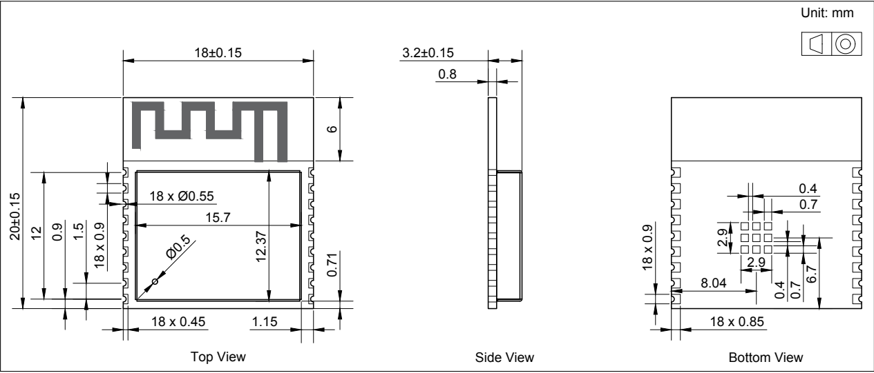
图 10-1. ESP32-C3-WROOM-02 尺寸
