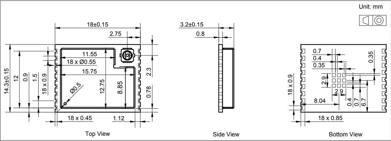
图 10-2. ESP32-C3-WROOM-02U 尺寸
