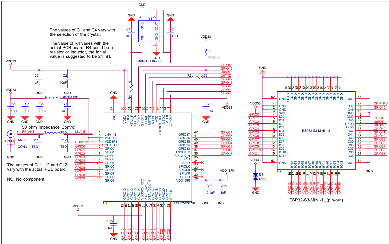
图 8-2. ESP32-S3-MINI-1U 原理图
