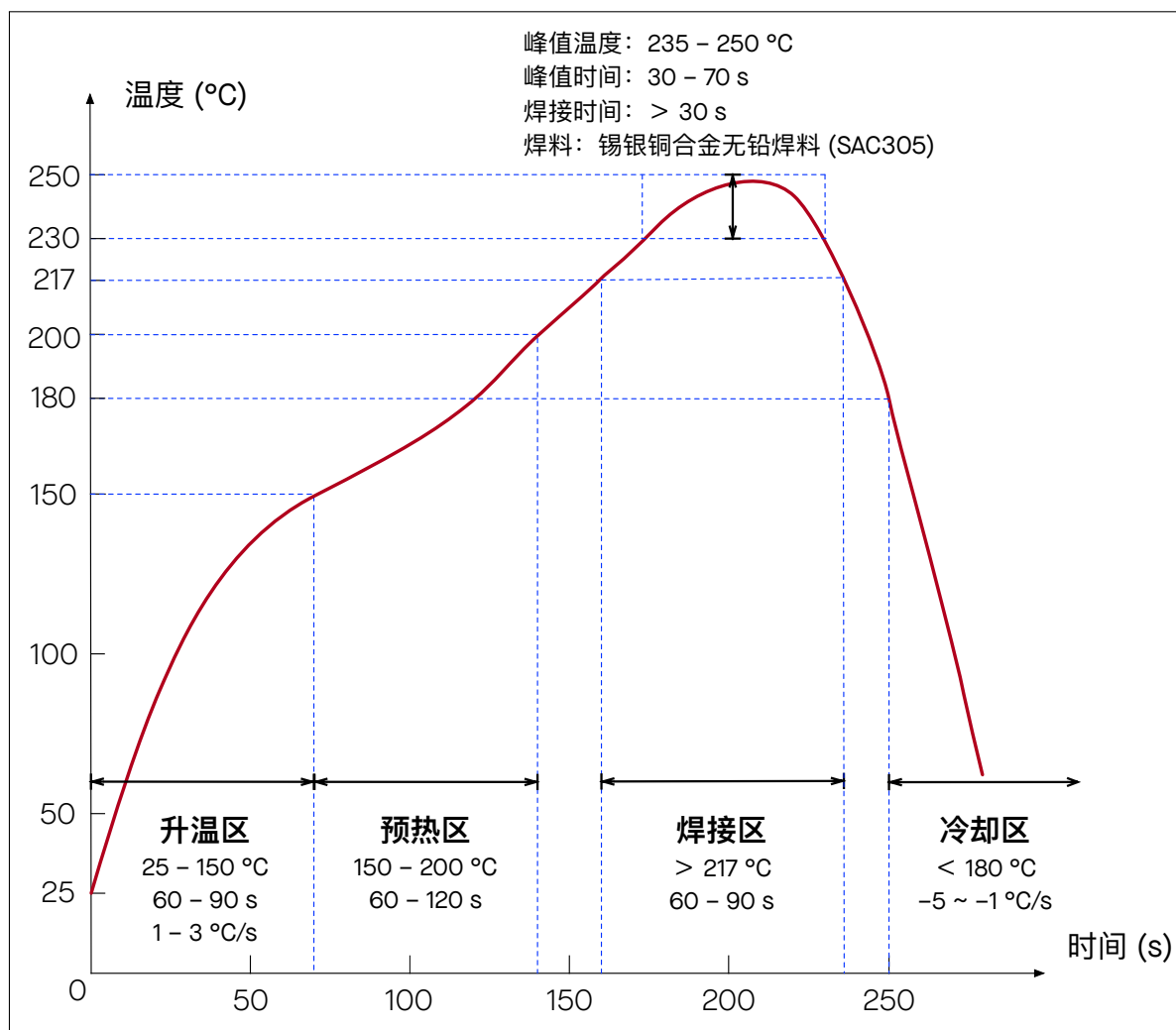
图 12-1. 回流焊温度曲线
