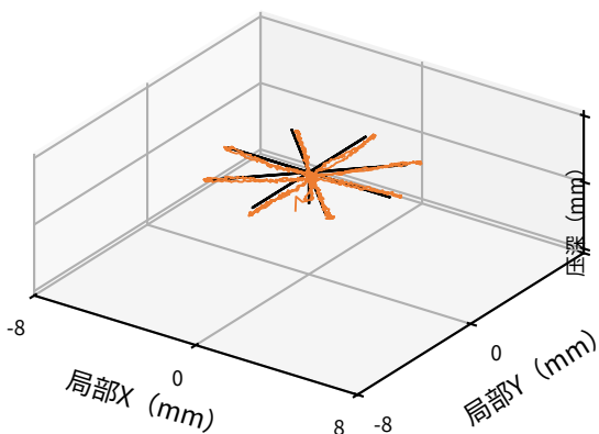
圆弧 原始/消偏 0.318/0.243 mm 覆盖率 99.8%
