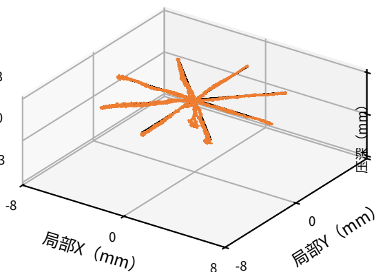
半球 原始/消偏 0.189/0.172 mm 覆盖率 99.9%
