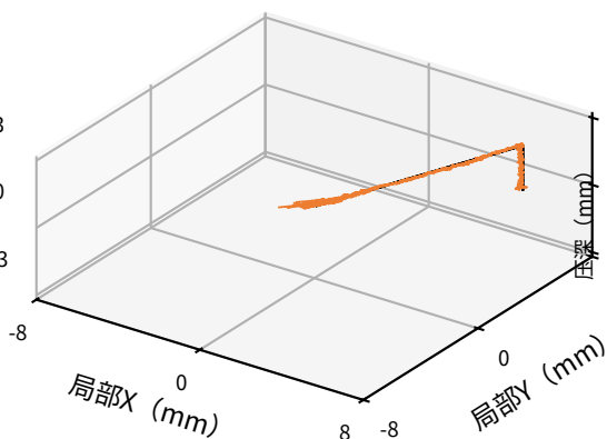
半球 原始/消偏 0.119/0.110 mm 覆盖率 99.8%
