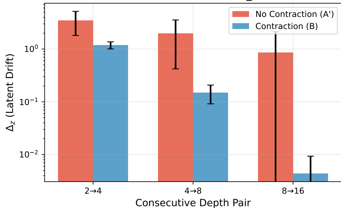
INCREMENTAL DRIFT: \Delta_z (B0)
